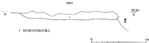
第27図 遺構面5 粘土貯蔵穴(S 541)断面図 1/20
