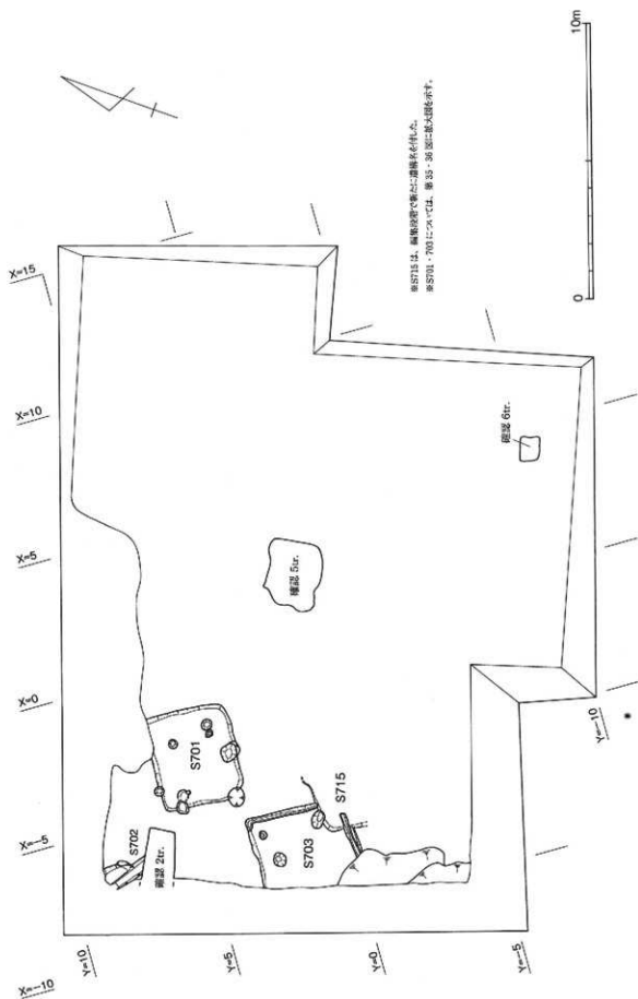
第34図 透視面7 透視配置図 1/150
