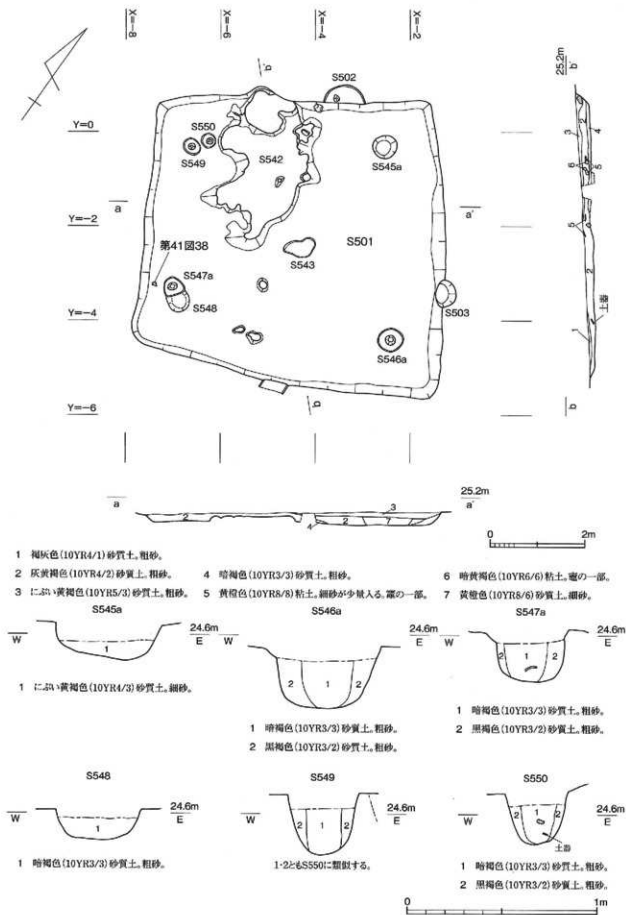
第25図 遺構面5 竪穴住居(S501)平面・断面図 1/80・関連ピット断面図 1/20
