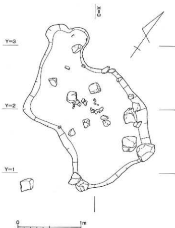
第32図 遺構面6 不定形土坑（S 608）平面図 1/30
