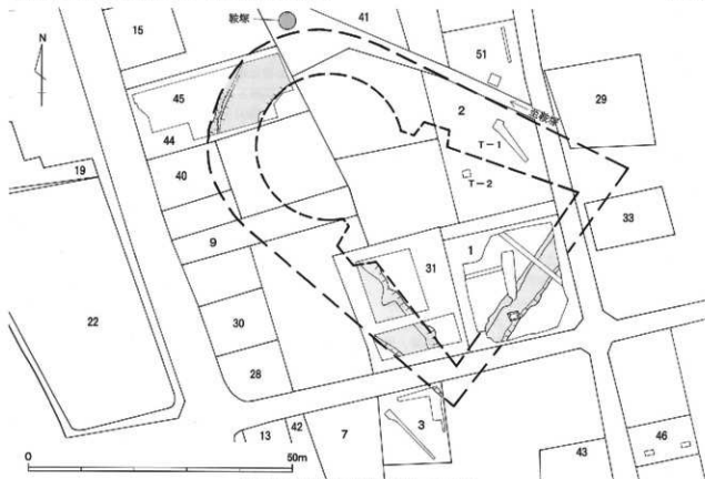
第56図 打出小竈古墳範囲推定図 1 / 800
