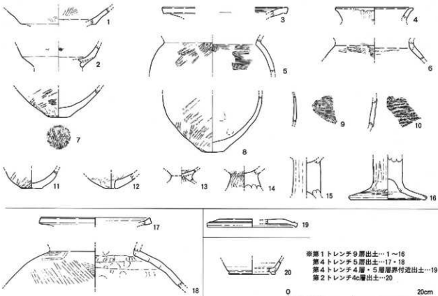
第7図 遺物実測図 1/4
