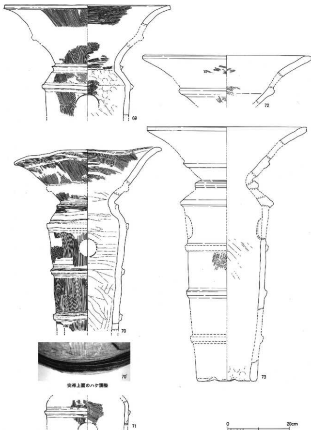
第49図 東区周濠出土銅器形輪実測図 1 / 6
