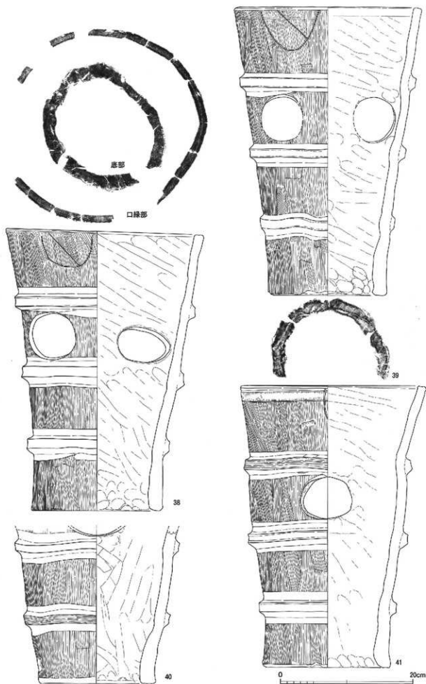
第44图 东区周濠出土普通円筒埴輪実測図(1) 1/4
