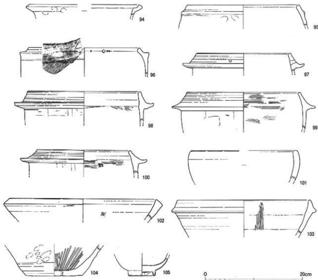
第52図 東区S D01出土遺物実測図(2) 1/4
