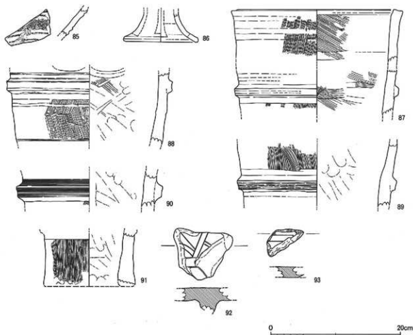
第51図 東区SD01出土遺物実測図(1) 1/4
