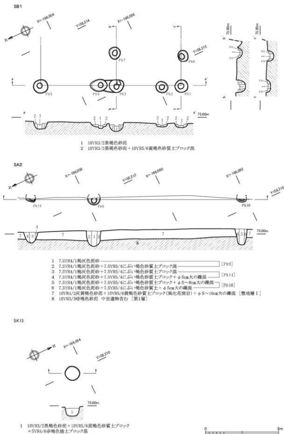
第5次調査区(2トレンチ)SB1、SA2、SK13平・断面図(1:50)
