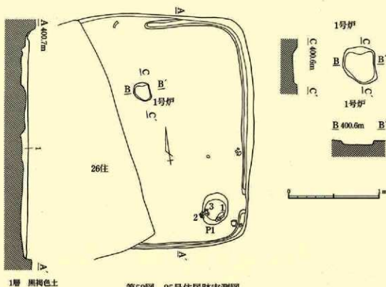
第52図 25号住居跡実測図
