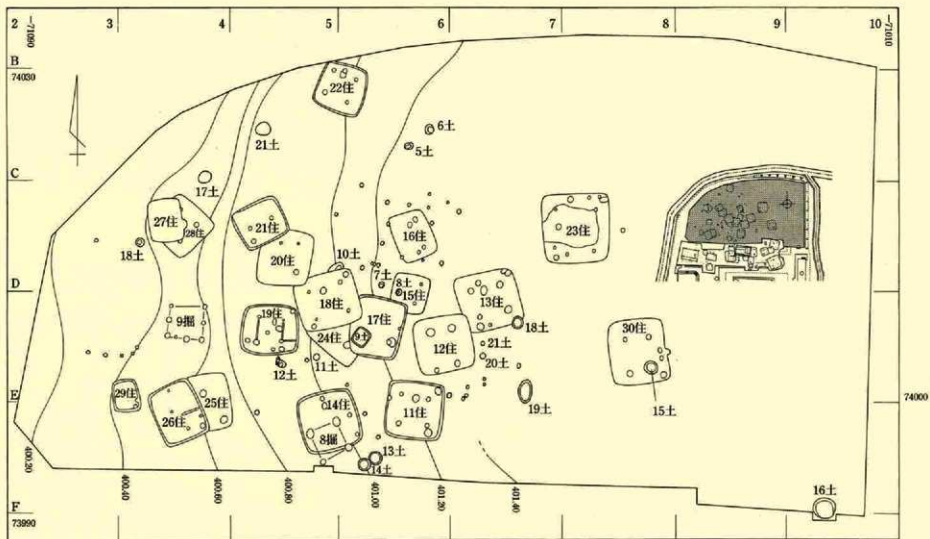
第36図 平成14年度調査区全体図
