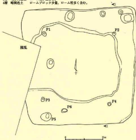
第51図 23号住居跡実測図
