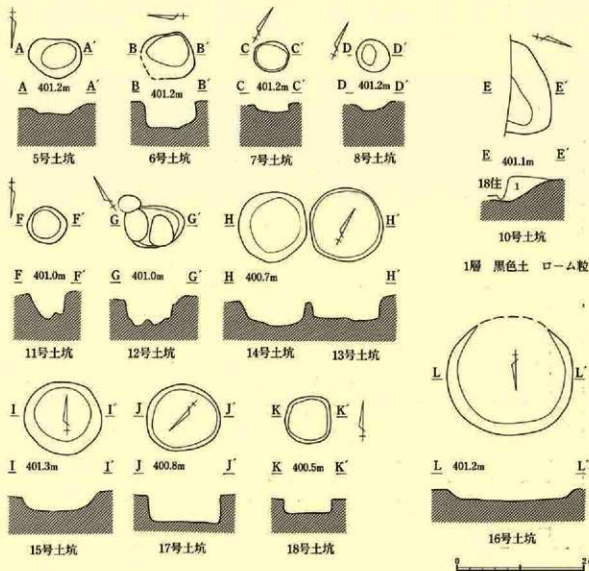
第75图 5~18号土坑実測図
