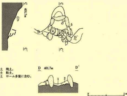
第27図 1号住居跡実測図
