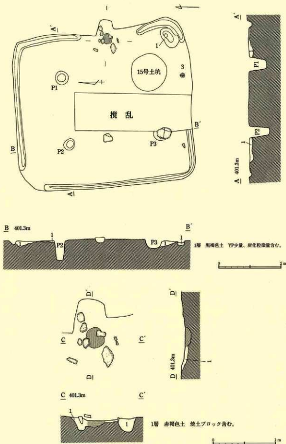
第71図 30号住居跡実測図
