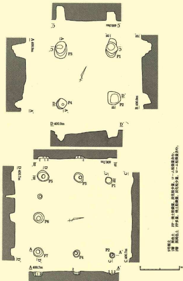
第72図 8・9号掘立柱建物跡実測図
