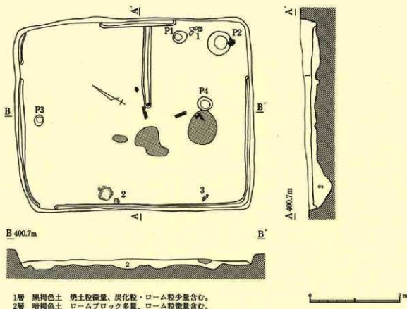
第53図 26号住居跡実測図
