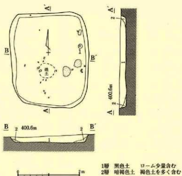
第17図 10号住居跡実測図
