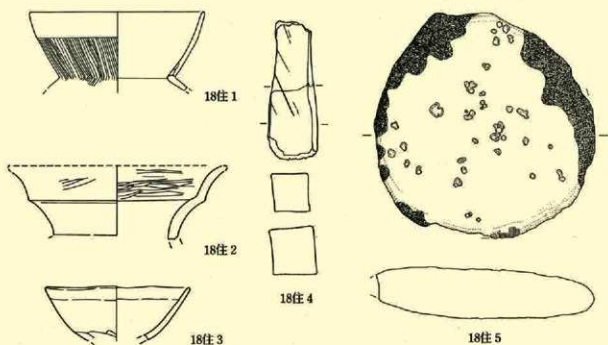
第60图 18号住居跡出土遺物実測図
