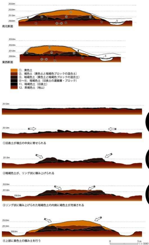
第204図 15号墳墳丘構築方法復元図
