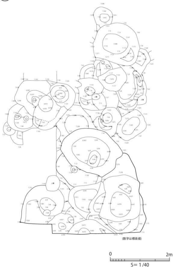
第 17 図 SD2 完掘状況平面図
