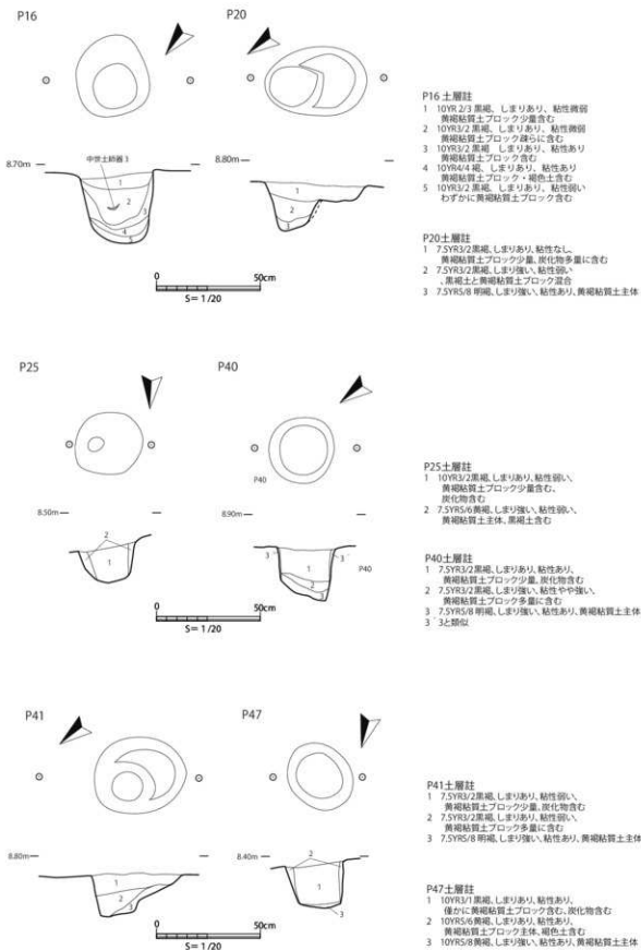
第 20 図 ピット遺構図
