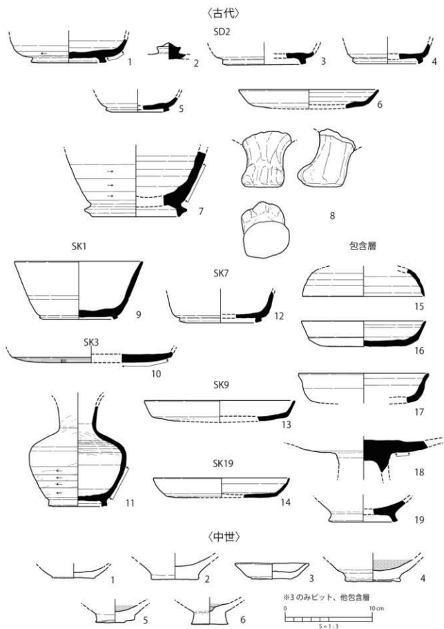
第 21 図 出土遺物実測図
