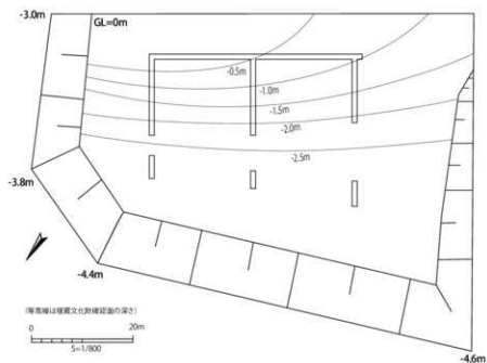
第2図 試掘調査のトレンチ配置図
