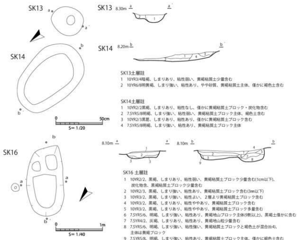
第 14 図 土坑遺構図 (SK13・SK14・SK16)
