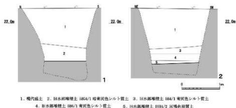
第 14 図 第 28 次調査土層断面図 (1/50)
