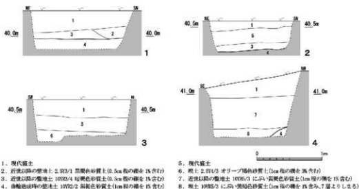
第 10 図 土層断面図 (1/40)
