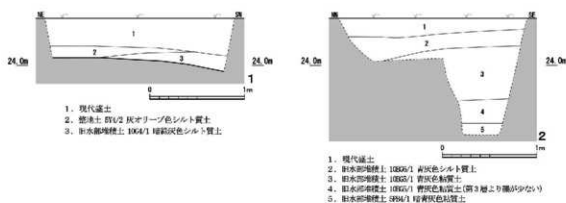
第 17 図 土層断面図 (1/40)
