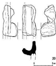
第25図 第12次調査出土竈実測図(1/3)
