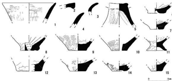
第7図 第3次調査出土遺物実測図(1/3)
