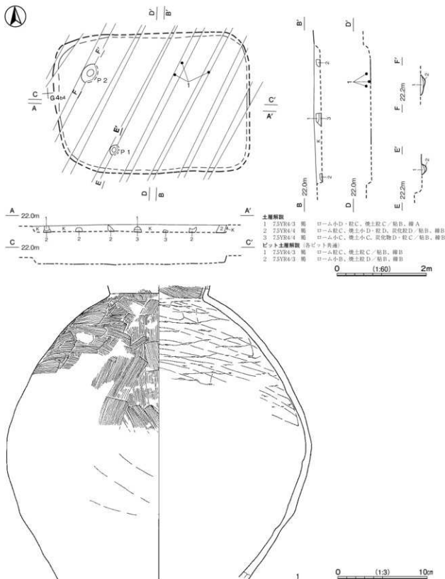
第 323 図 第 48 号竪穴建物跡・出土遺物実測図
