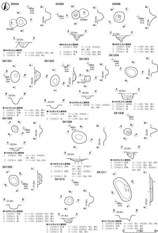
第 357 図 その他の土坑実測図③
