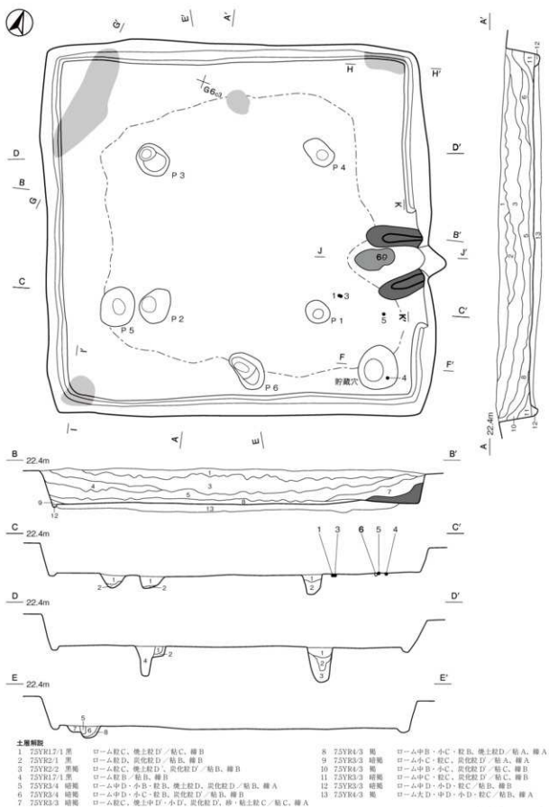
第331図 第113号堅穴建物跡実測図
