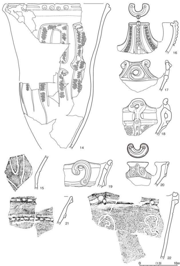
第 395 図 遺構外出土遺物実測図(2)
