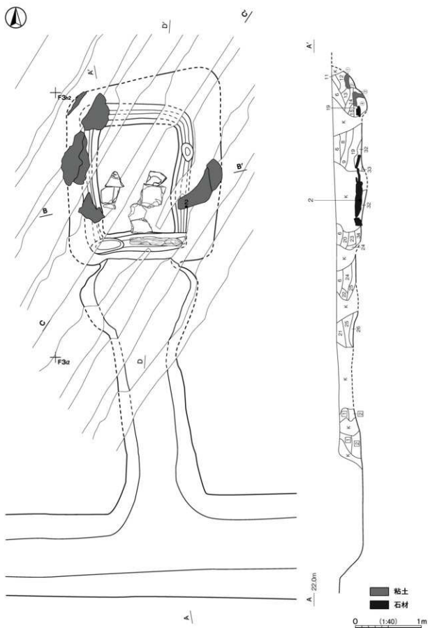
第 339 图 第 1 号墳石室実測図(1)
