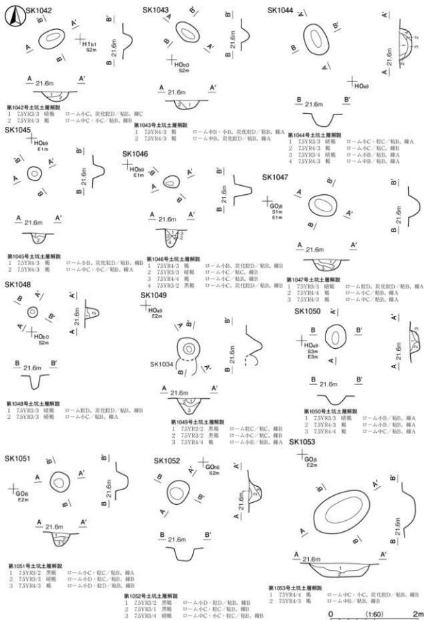
第 360 図 その他の土坑実測図99
