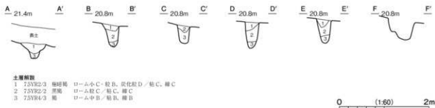
第391図 第5号溝跡実測図
