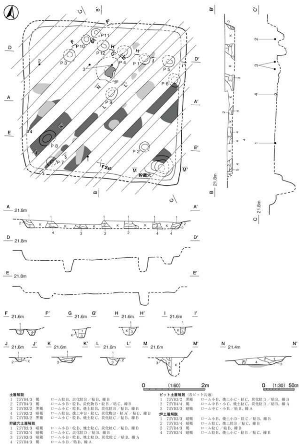
第 327 図 第 71 号竪穴建物跡実測図
