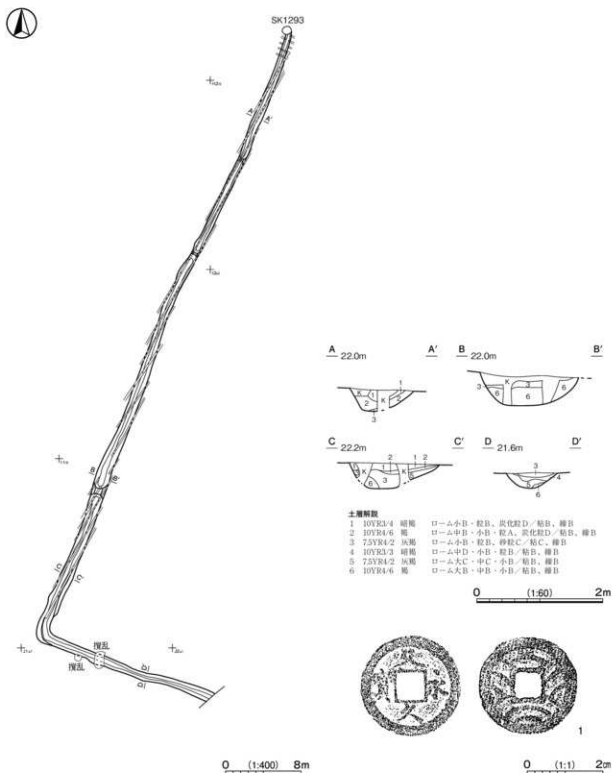
第388図 第3号溝跡・出土遺物実測図
