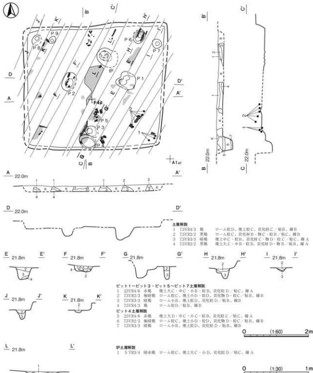
第 324 図 第 53 号竪穴建物跡実測図
