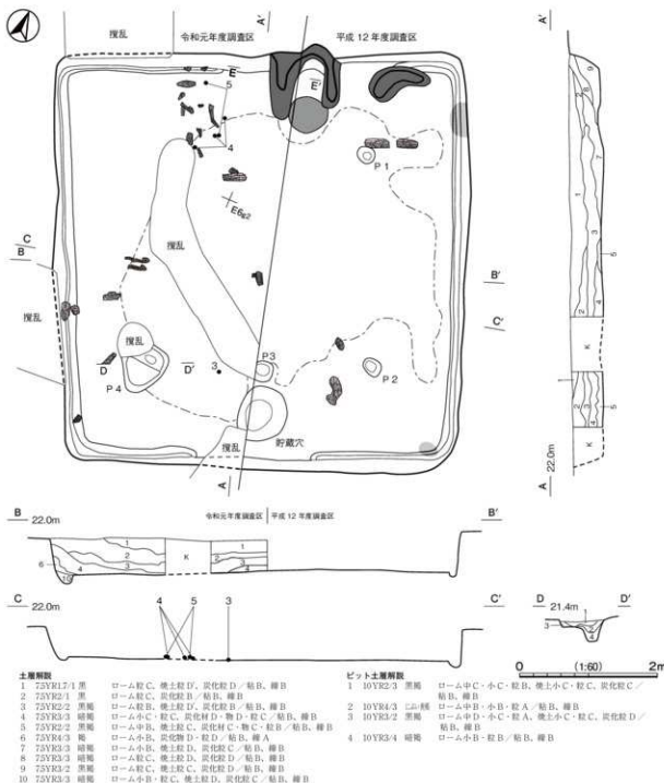
第317図 第15号堅穴建物跡実測図
