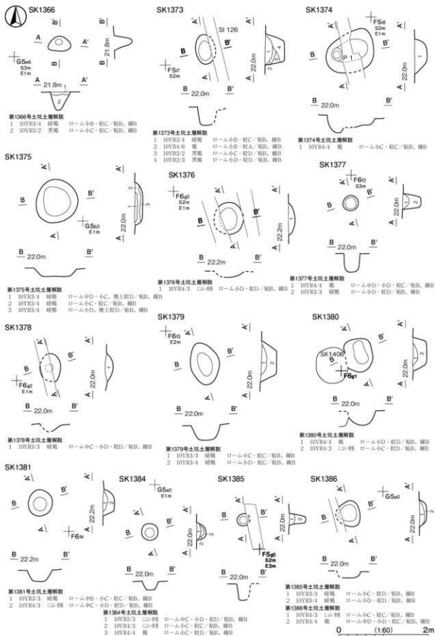
第378図 その他の土坑実測図③
