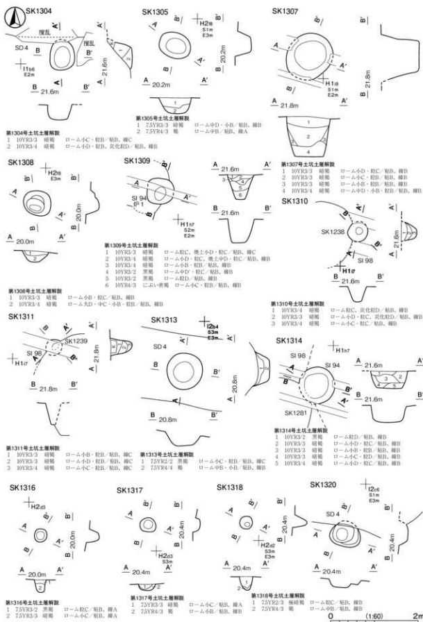
第 375 図 その他の土坑実測図34
