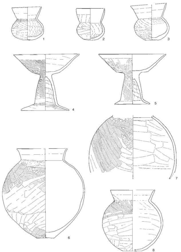
第330図 第112号竪穴建物跡出土遺物実測図
