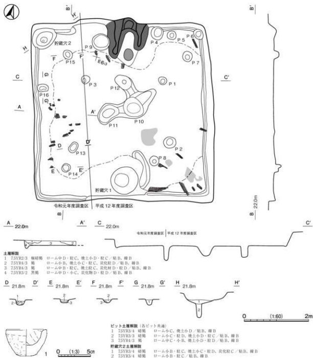
第 319 図 第 16 号堅穴建物跡・出土遺物実測図
