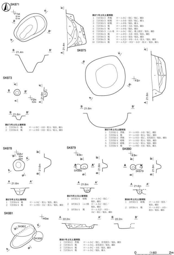
第 349 図 その他の土坑実測図(8)
