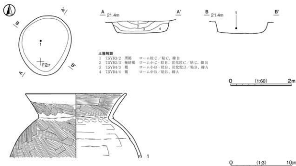
第337図 第888号土坑・出土遺物実測図
