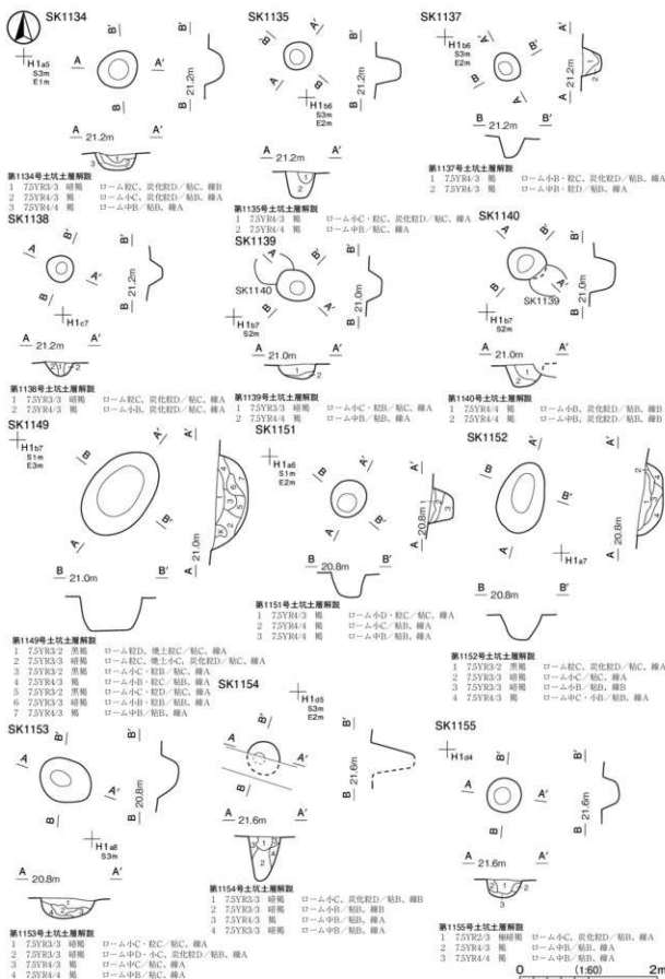
第 367 図 その他の土坑実測図②
