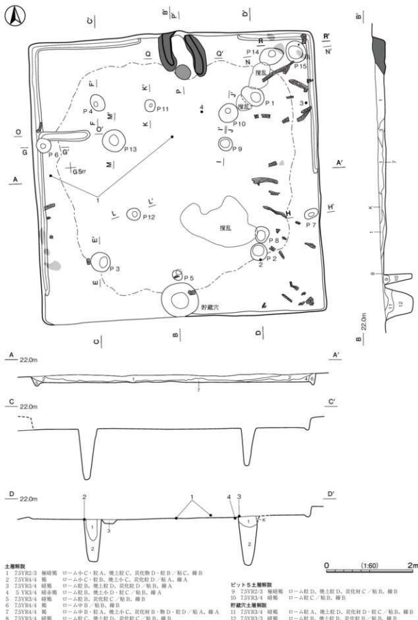
第 333 図 第 114 号堅穴建物跡実測図
