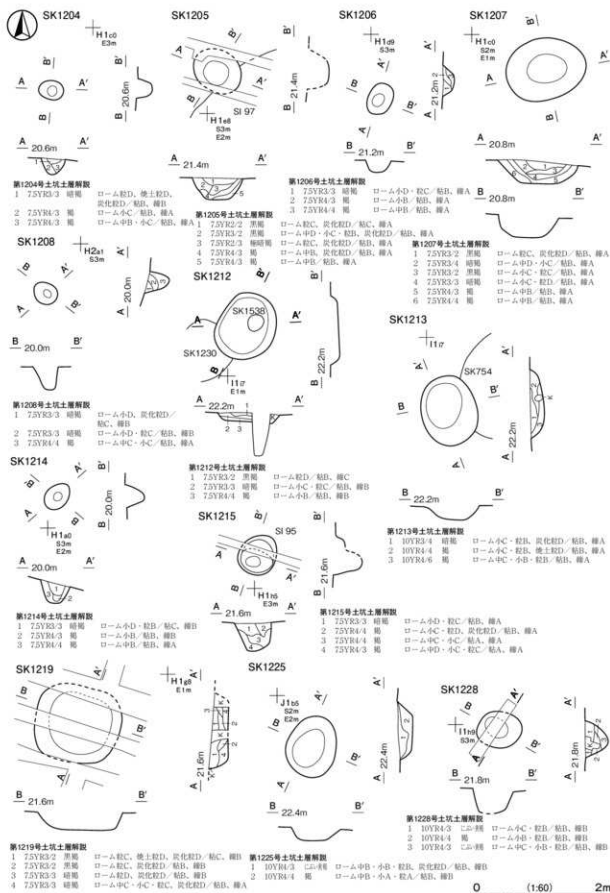
第370図 その他の土坑実測図(29)
