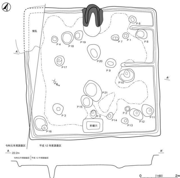
第 320 図 第 17 号竪穴建物跡実測図
