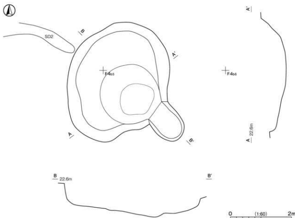
第637図 第22号土坑実測図
