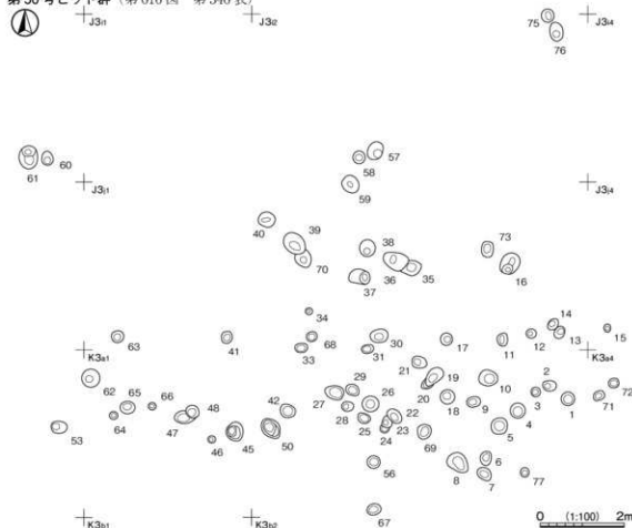
第616図 第50号ビット群実測図
