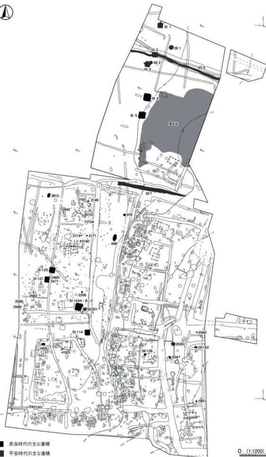
第 645 図 奈良・平安時代の主要遺構分布図
