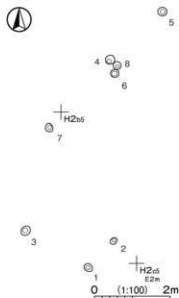
第627図 第72号ビット群実測図
