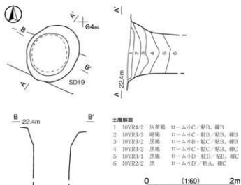
第634図 第3号井戸跡実測図
