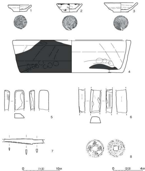
第601図 第38号ピット群出土遺物実測図
