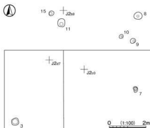
第597図 第34号ビット群実測図
