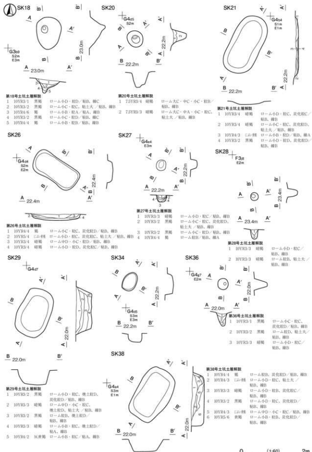
第 641 図 時期不明のその他の土坑実測図(2)
