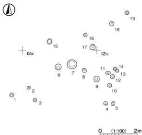
第623図 第58号ビット群実測図
