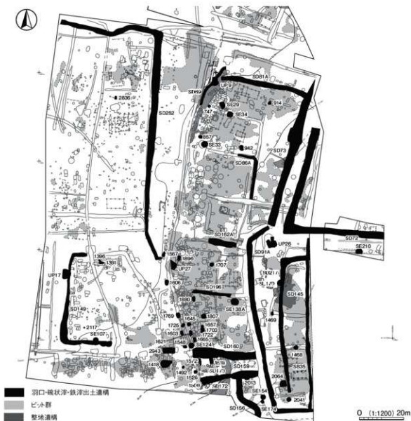
第651図 羽口・椀状滓・鉄滓出土遺構分布図
