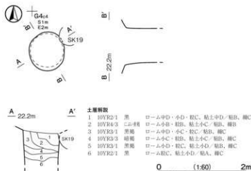
第635図 第4号井戸跡実測図
