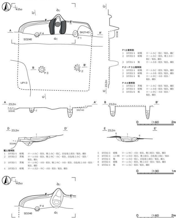
第633図 第119号竪穴建物跡実測図
