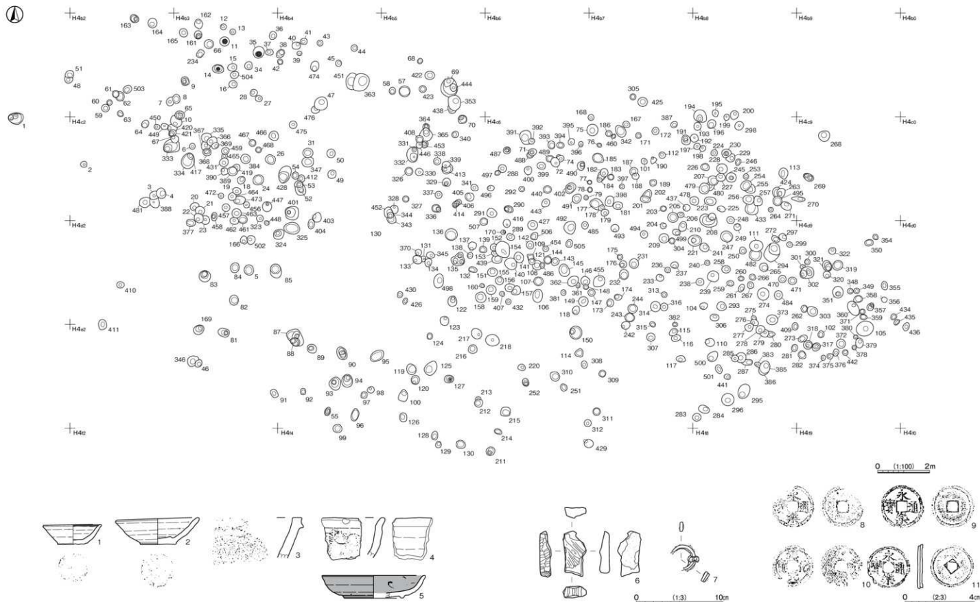
第590図 第20号ピット群実測図・出土遺物実測図
