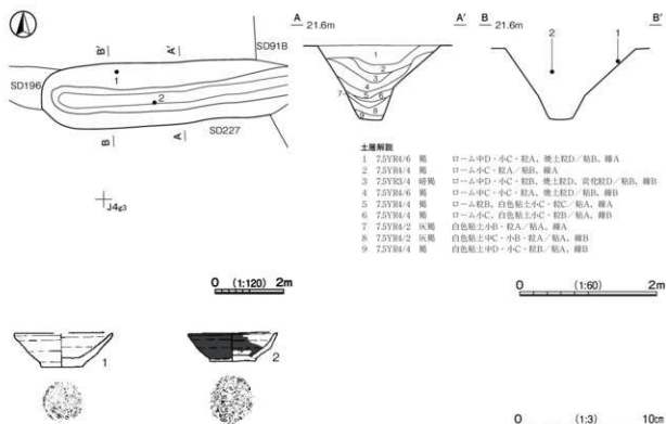
第353図 第227号堀跡・出土遺物実測図
