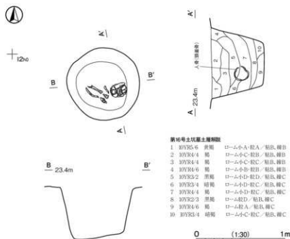
第391図 第16号土坑墓出土遺物実測図
