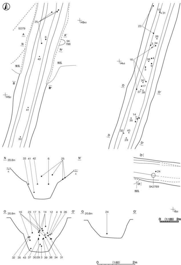
第 296 図 第 72 号堀跡実測図(2)
