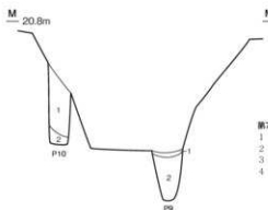
第297図 第72号掘跡実測図(3)
