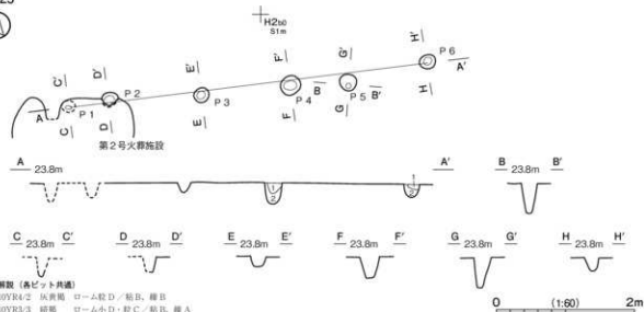
第380図 室町時代から江戸時代の柱穴実測図(3)
