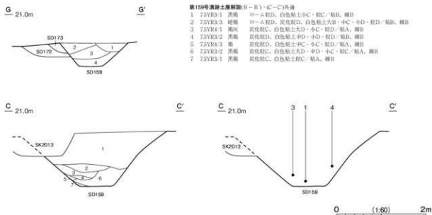
第334図 第159号堀跡実測図
