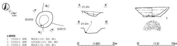
第548図 第1491号土坑・出土遺物実測図
