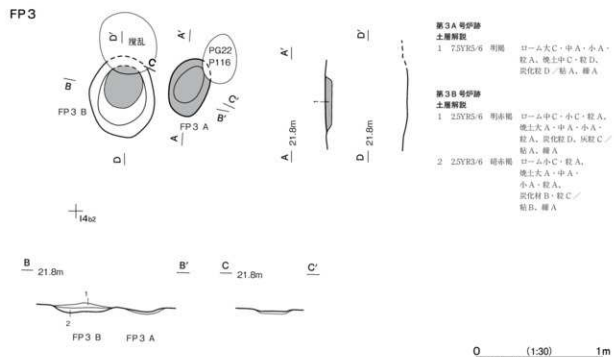
第384図 室町時代から江戸時代の炉跡実測図(1)
