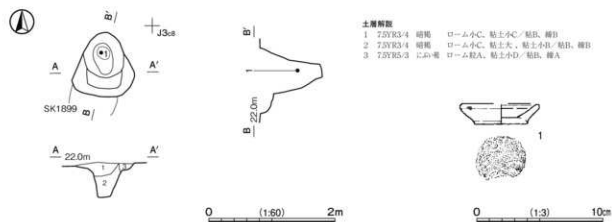
第563図 第1910号土坑・出土遺物実測図
