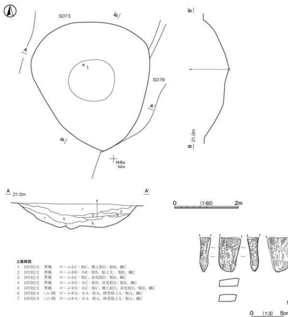
第 503 図 第 794 号土坑・出土遺物実測図
