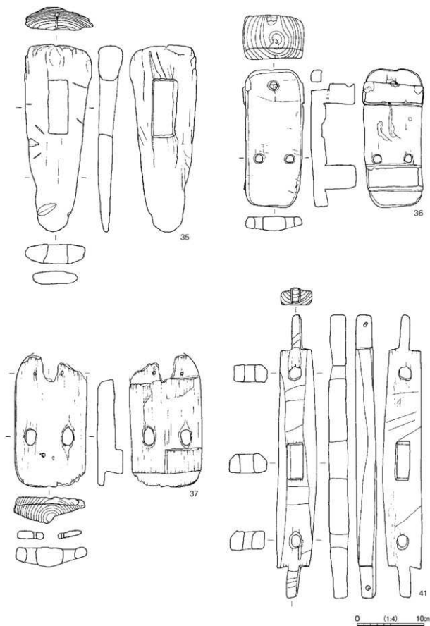
第302図 第72号堀跡出土遺物実測図(5)
