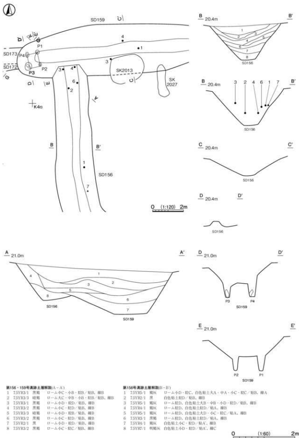
第333図 第156・159号堀跡実測図
