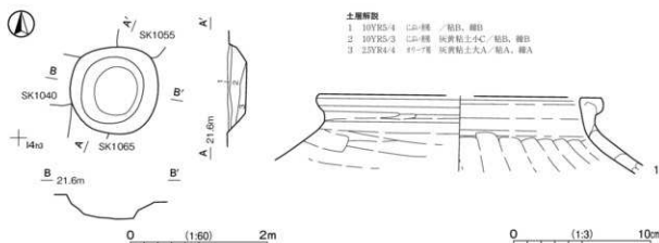
第528図 第1054号土坑・出土遺物実測図
