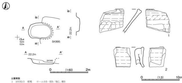
第524図 第996号土坑・出土遺物実測図
