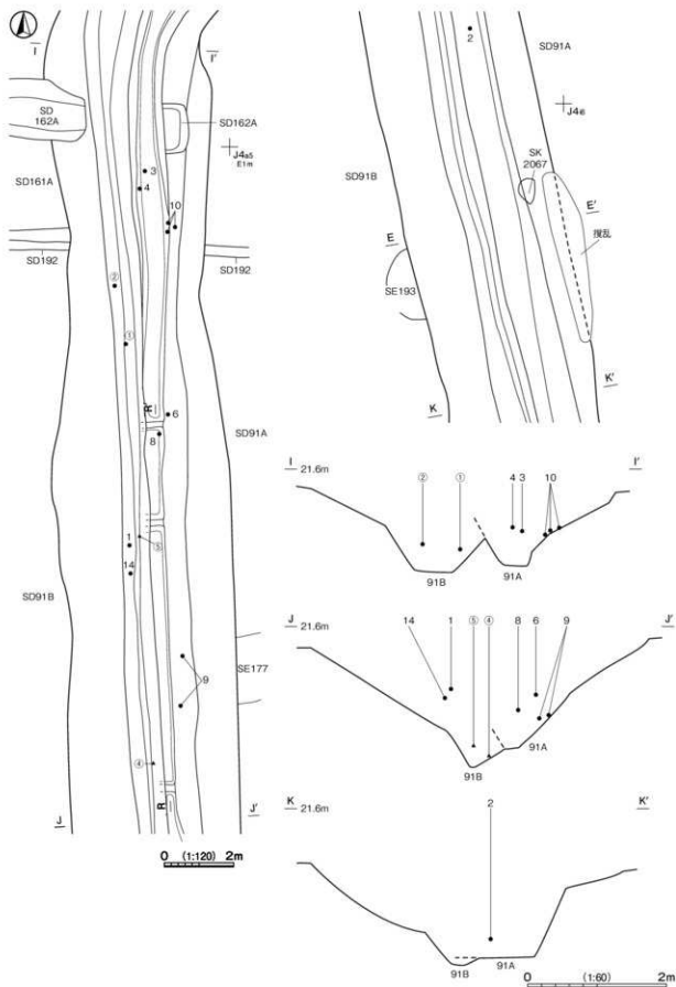
第 321 图 第 91A · B 号堀跡実測图(4)
