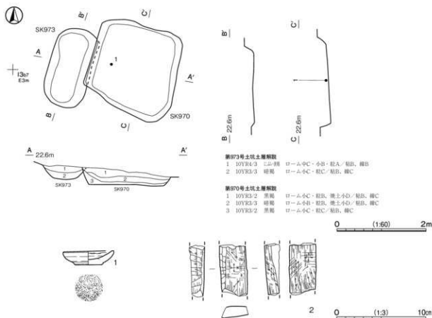
第520図 第970・973号土坑・出土遺物実測図
