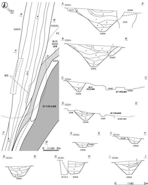
第 291 図 第 63A・B 号溝跡実測図(1)
