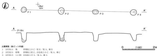
第376図 第7号柱穴列実測図
