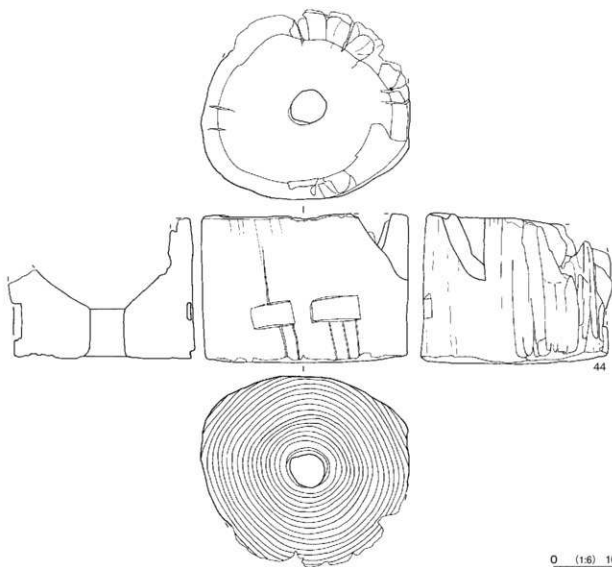
第311図 第73号堀跡出土物実測図(5)
