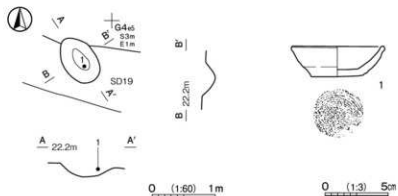
第494図 第42号土坑・出土遺物実測図
