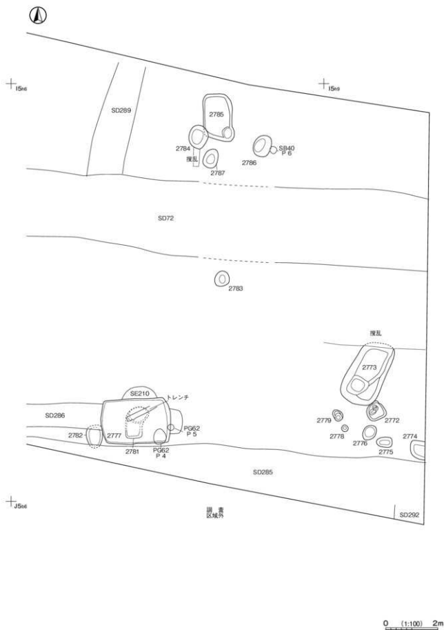
第 450 図 土坑平面図 (44)
