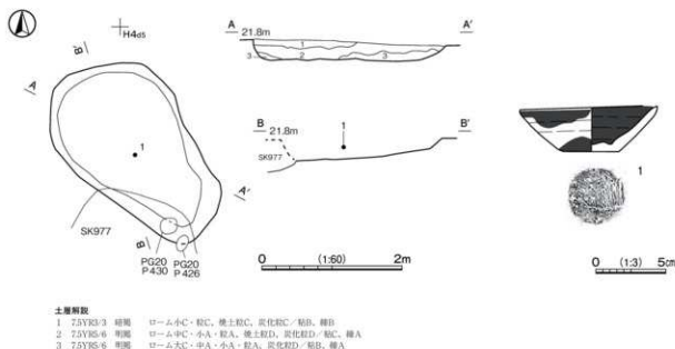
第522図 第987号土坑・出土遺物実測図
