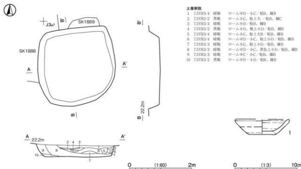
第561図 第1884号土坑・出土遺物実測図
