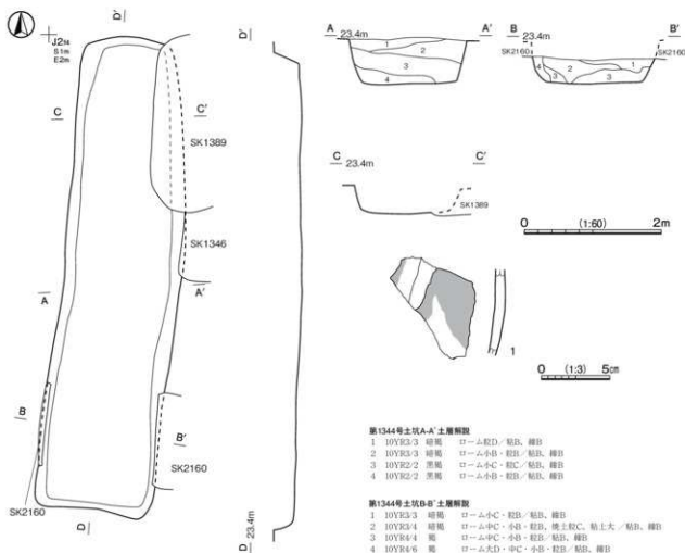
第 539 図 第 1344 号土坑・出土遺物実測図
