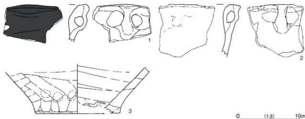
第287図 第16号溝跡出土遺物実測図
