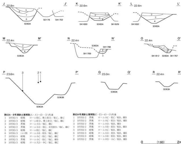
第292図 第63A・B号溝跡実測図(2)
