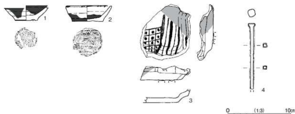
第344図 第169号溝跡出土遺物実測図
