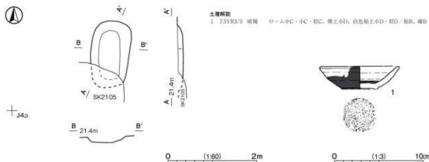
第566図 第2016号土坑・出土遺物実測図
