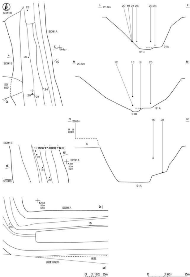
第 322 図 第 91A・B 号堀跡実測図(5)
