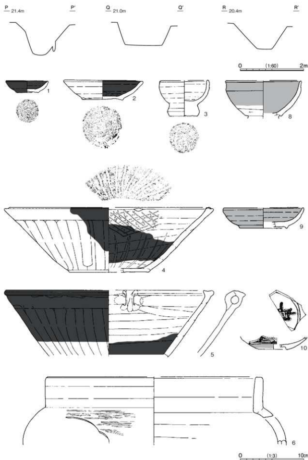
第 351 图 第 217 号沟迹・出土遺物実測図
