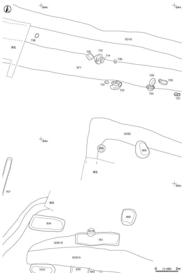
第 417 图 土坑平面图 (11)
