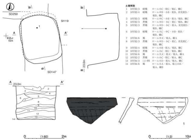
第 577 図 第 2947 号土坑・出土遺物実測図
