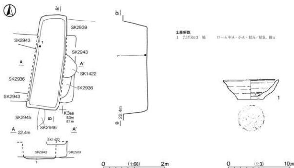
第576図 第2937号土坑・出土遺物実測図
