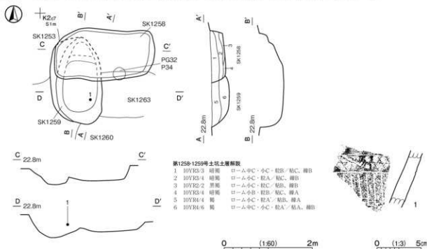
第 534 图 第 1258·1259 号土坑·出土遗物实测图
