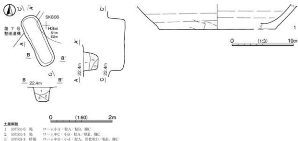
第 500 図 第 749 号土坑・出土遺物実測図
