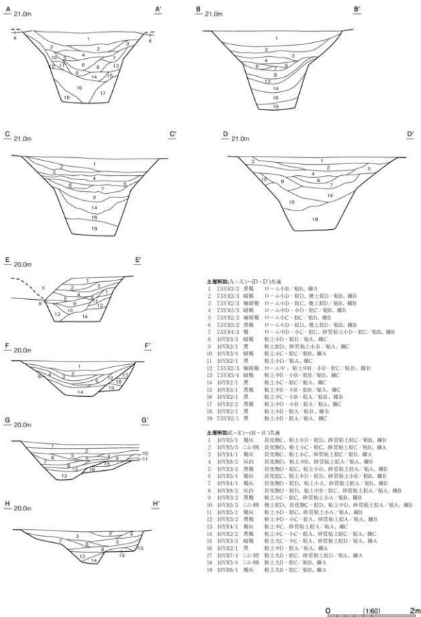
第 295 图 第 72 号掘跡実測図(1)
