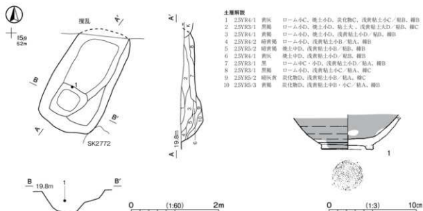
第 573 図 第 2773 号土坑・出土遺物実測図
