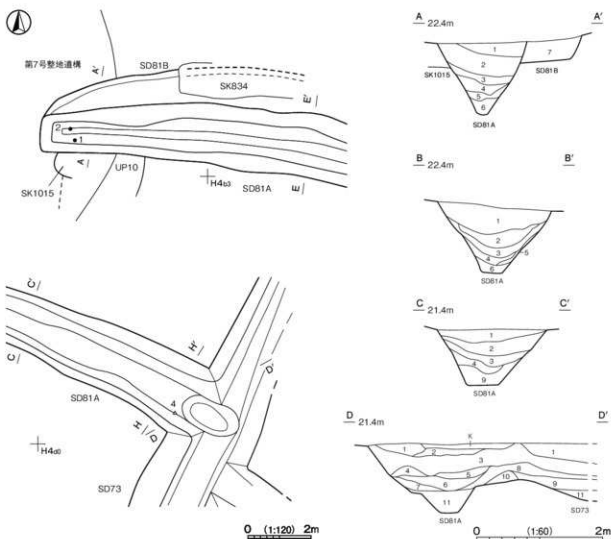
第312図 第81A号堀跡・第81B号溝跡実測図
