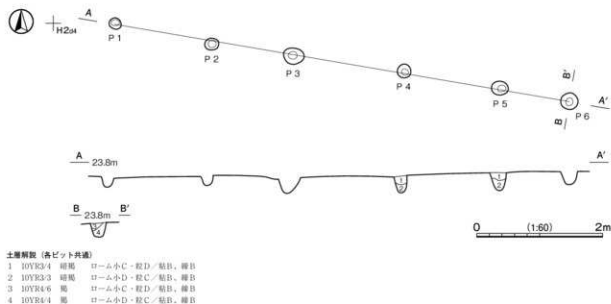
第377図 第19号柱穴列実測図
