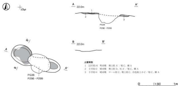
第382図 第8号炉跡実測図
