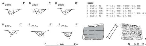
第282図 第2号溝跡・出土遺物実測図
