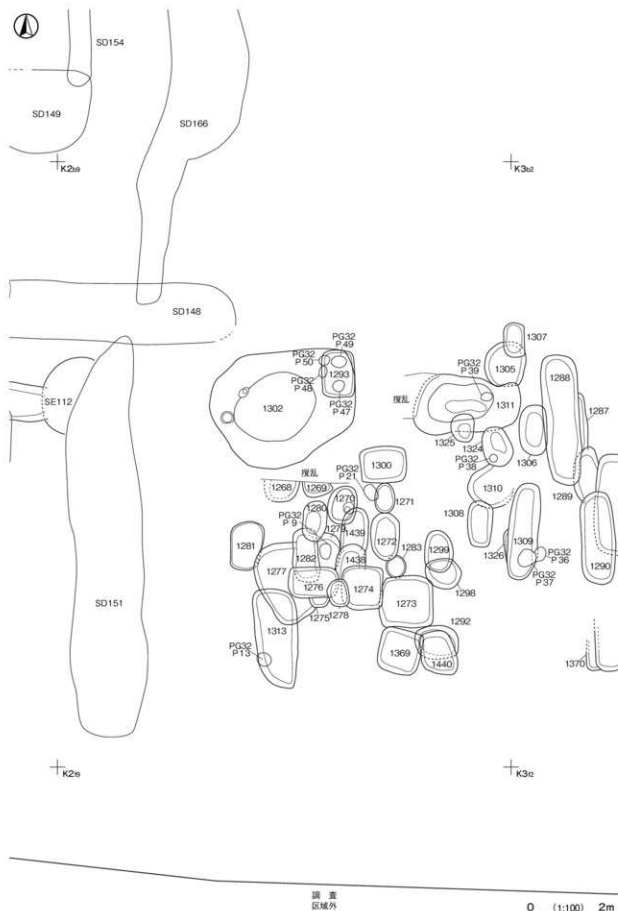
第 484 図 土坑平面図 (78)
