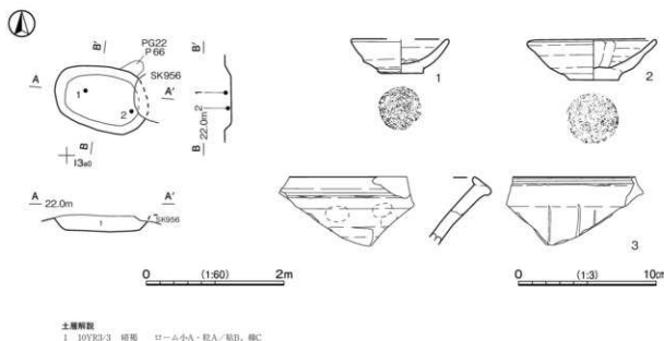
第517図 第916号土坑・出土遺物実測図
