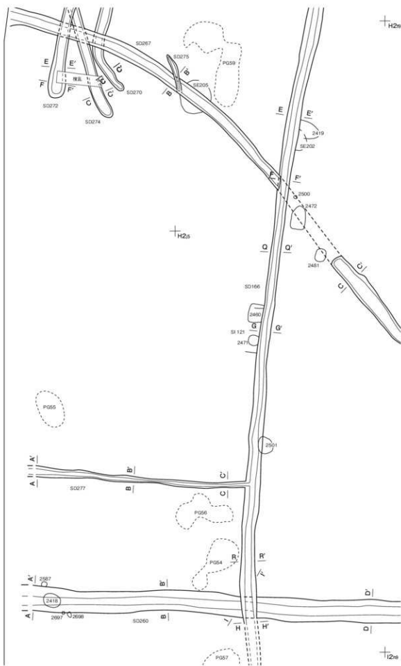
第 279 图 溝跡・堀跡平面図 (21)
