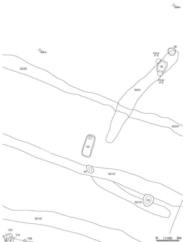
第 411 図 土坑平面図 (5)
