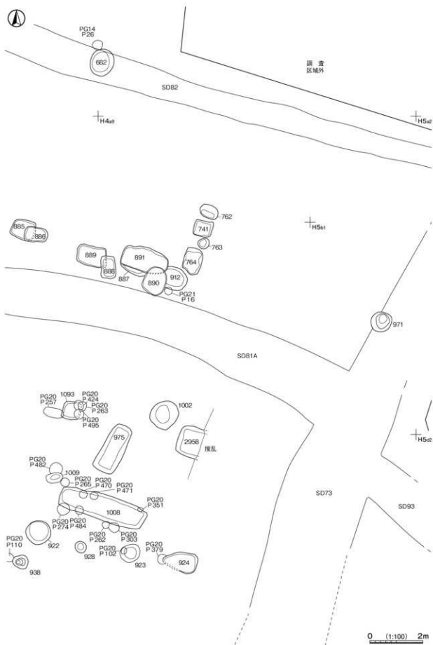
第 419 图 土坑平面图 (13)
