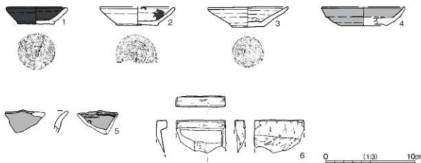
第342図 第162A号堀跡出土遺物実測図
