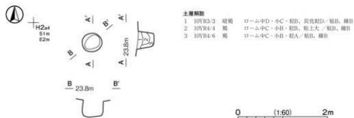
第 575 図 第 2823 号土坑実測図
