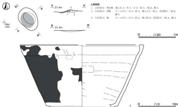
第381図 第2号炉跡・出土遺物実測図
