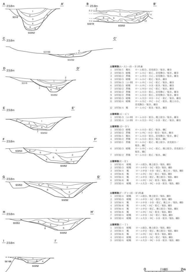
第 354 图 第 252 号清砂迹测图(1)
