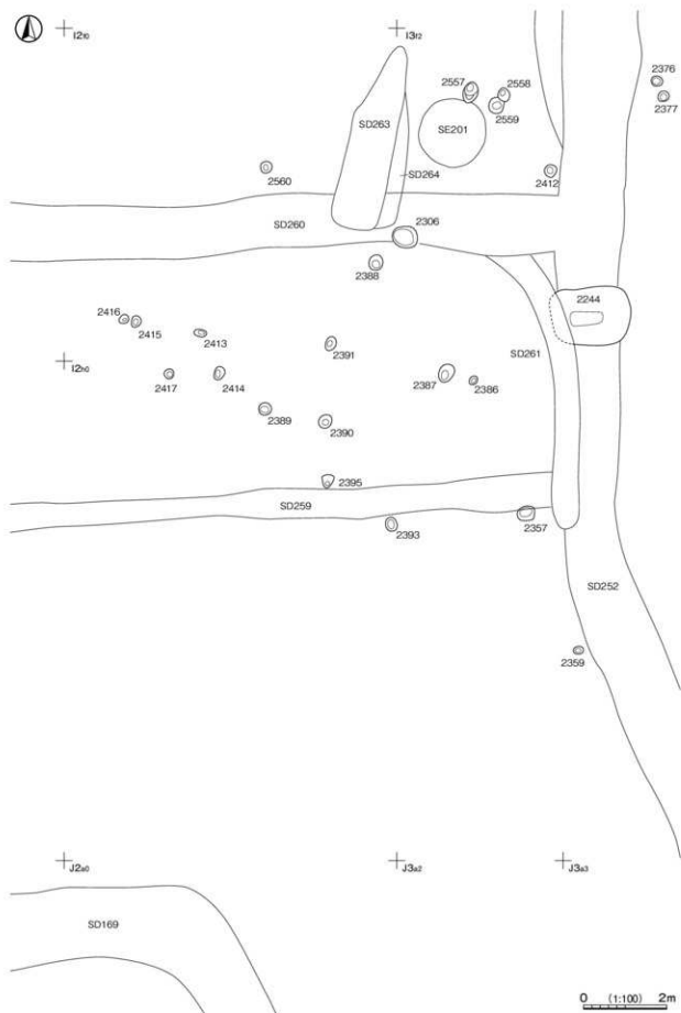
第 454 图 土坑平面图 (48)
