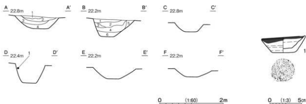
第290図 第19号溝跡・出土遺物実測図
