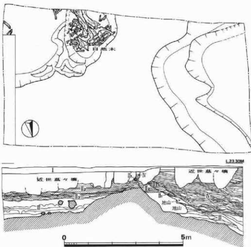
第5図 本調査区実測図 (1/80)
