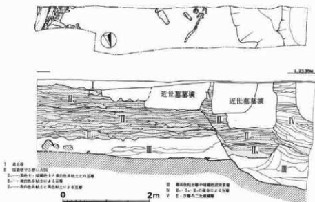
第3図 第1トレンチ実測図 (1/60)
