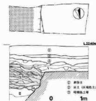
第4図 第2トレンチ実測図 (1/60)
