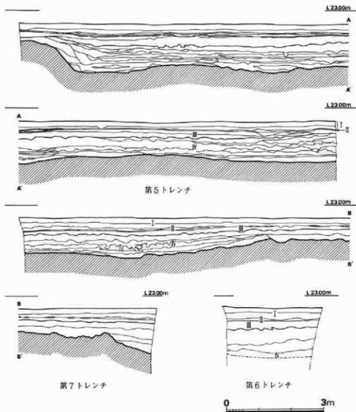
第7図 第5・6・7トレンチ南壁土層図 (1/80)
