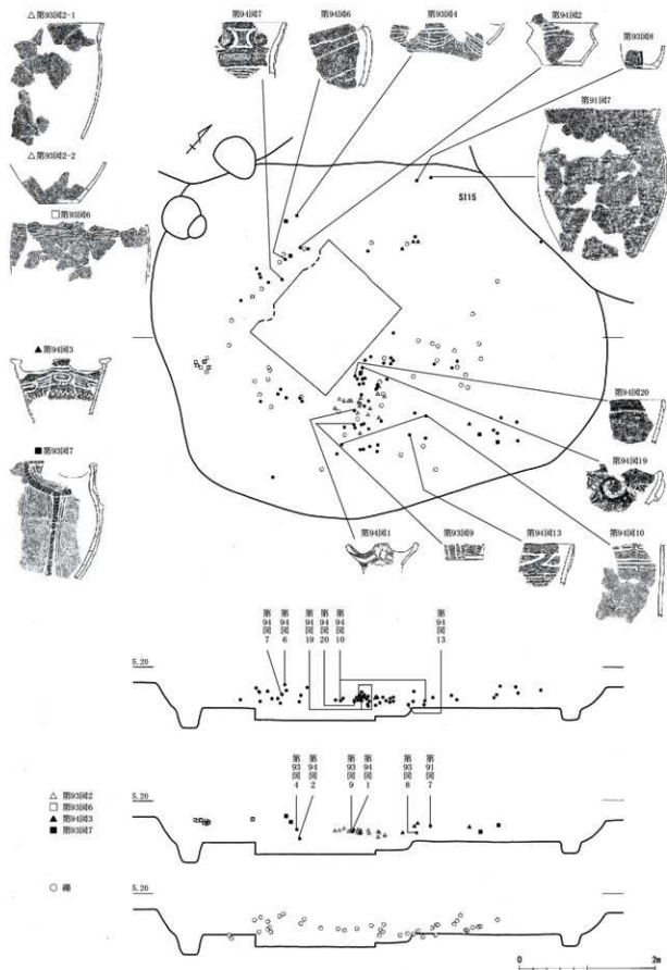
第37図 SI15 遺物出土状況図 (縮尺 1/60)
