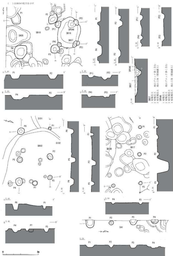
第61図 SB03・17-19, SA1 実測図 (縮尺 1/60)
