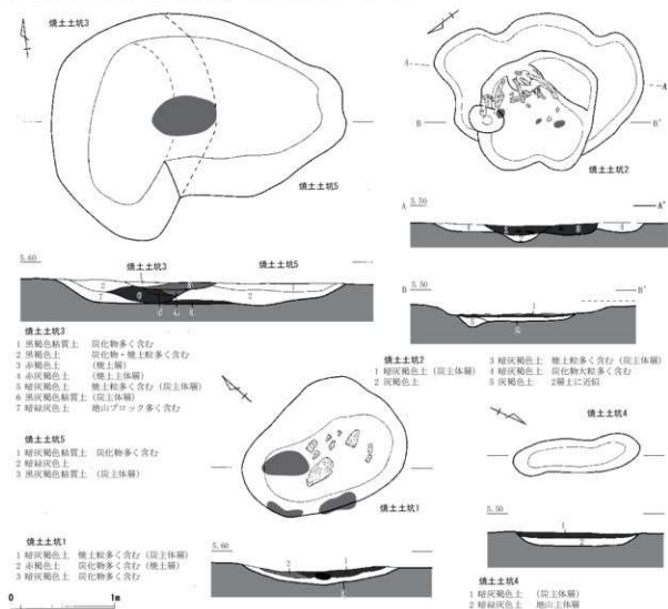
第63図 焼土土坑実測図 (縮尺 1/40)
