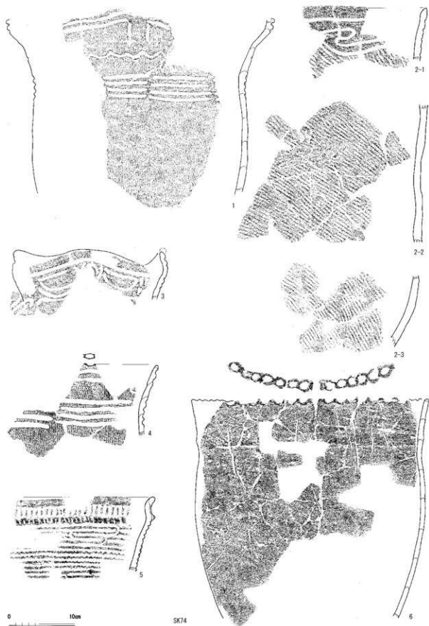
第121図 土坑出土土器実測図8 (縮尺 1/4)
