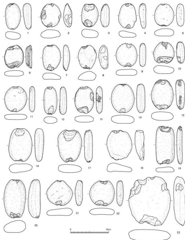
第153図 石錘実測図2 (縮尺 1/3)
