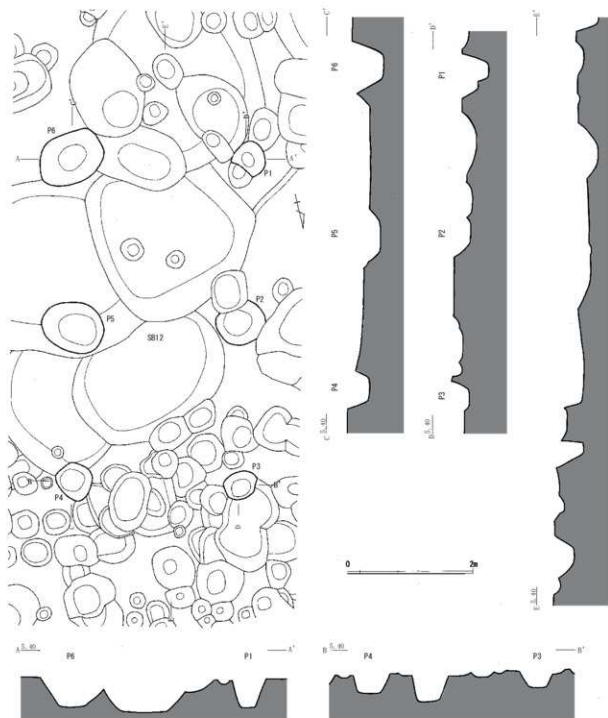
第58図 SB12 実測図 (縮尺 1/60)
