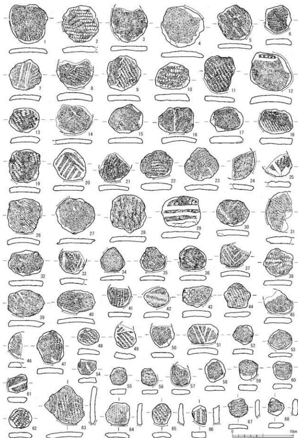
第162図 土製円盤実測図 (縮尺 1/3)
