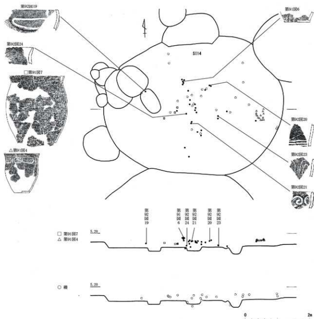
第34図 SI14 遺物出土状況図 (縮尺 1/60)
