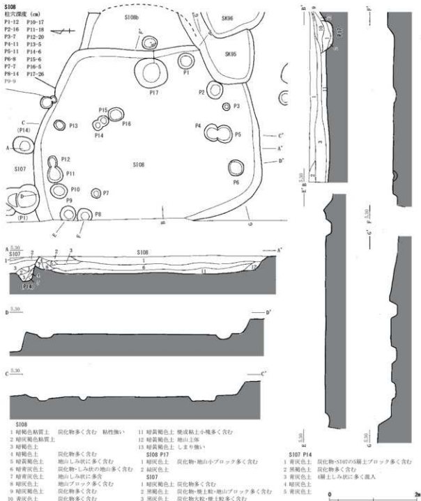
第23図 S108 実測図 (縮尺 1/60)
