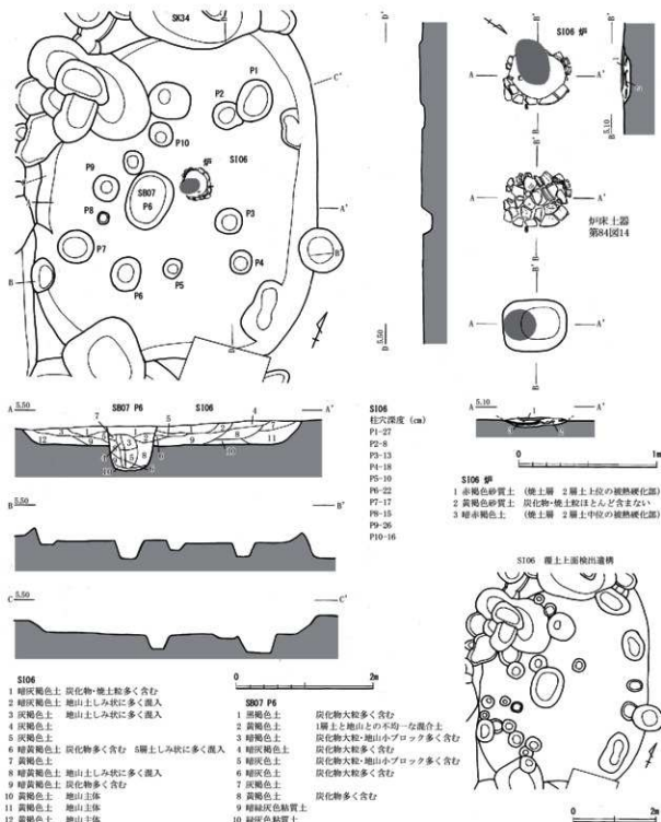
第17図 S106 実測図 (縮尺 1/100・1/60・1/30)
