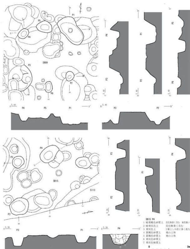
第56図 SB09・15 実測図 (縮尺 1/60)
