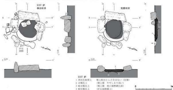
第19図 S107 炉実測図 (縮尺 1/30)
