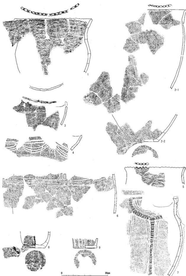
第93図 SI15出土土器実測図1 (縮尺 1/5)
