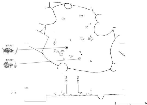
第18図 S106 遺物出土状況図 (縮尺 1/60)
