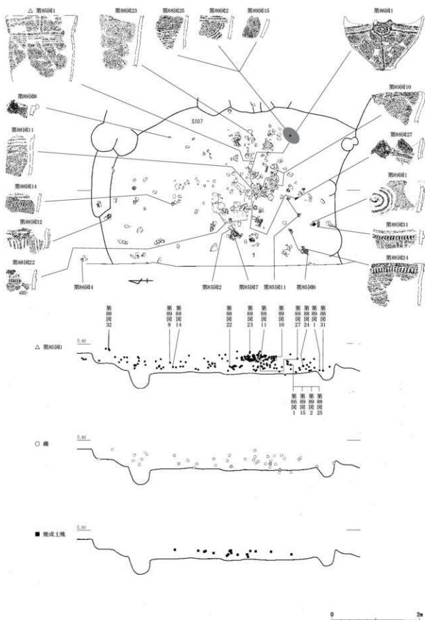
第21図 SI07 遺物出土状況図1 (縮尺 1/60)
