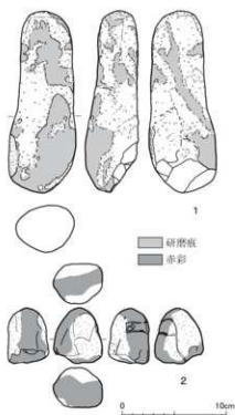
第160図 その他の石製品実測図 (縮尺 2/3)
