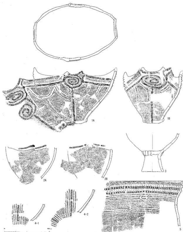
第86図 S107 出土土器実測図2 (縮尺 1/5)
