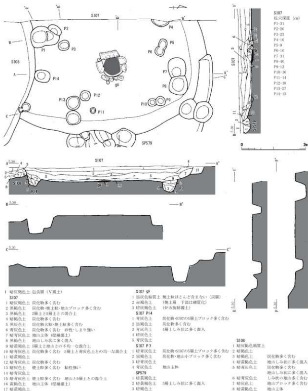
第20図 S107 実測図 (縮尺 1/60)
