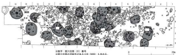
第6図 竪穴住居配置図（縮尺 1/500）
