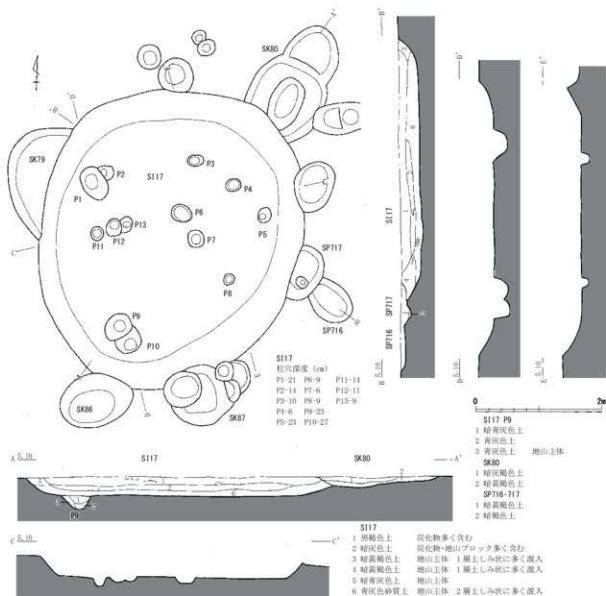
第40図 SI17 実測図 (縮尺 1/60)
