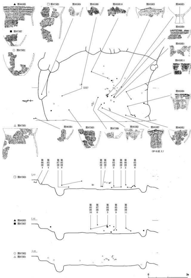
第22図 SI07 遺物出土状況図2 (縮尺 1/60)
