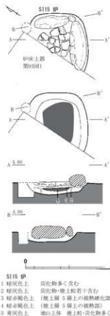
第35図 SI15 炉実測図（縮尺 1/30）
