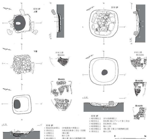
第43図 SI18・19 炉実測図 (縮尺 1/30)
