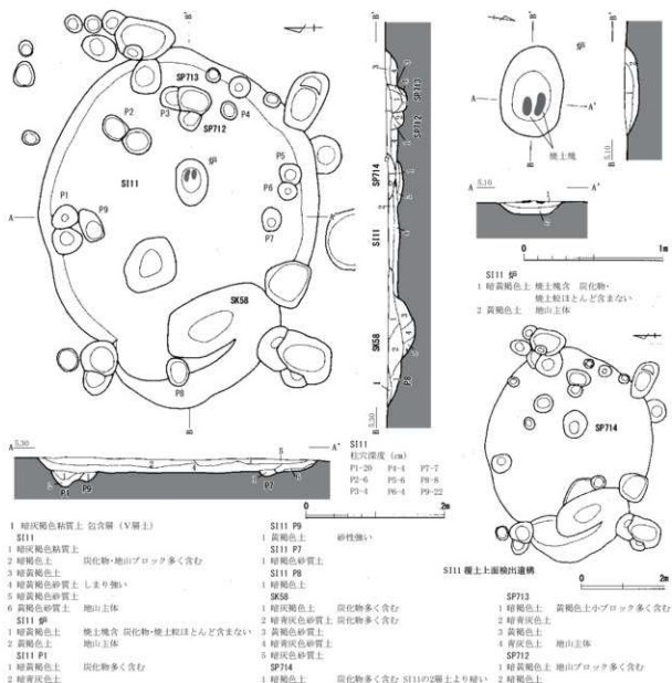
第30図 S111 実測図 (縮尺 1/100・1/60・1/30)
