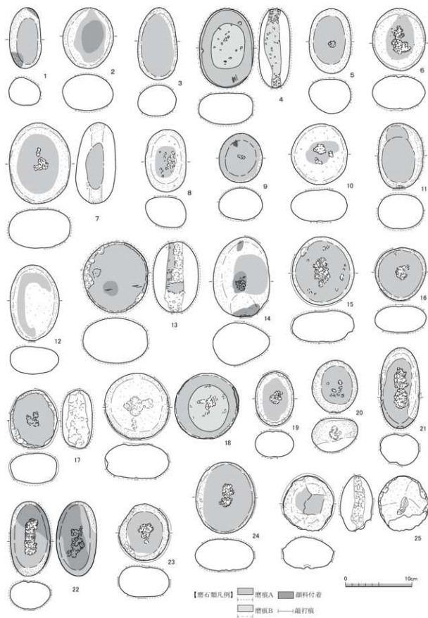
第154図 磨石類実測図1 (縮尺 1/4)
