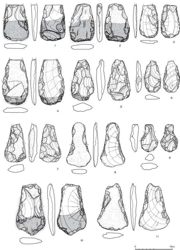
第148図 打製石斧実測圖3 (縮尺 1/3)
