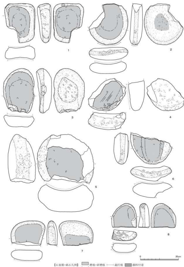
第157図 石皿類実測図（縮尺 1/6）
