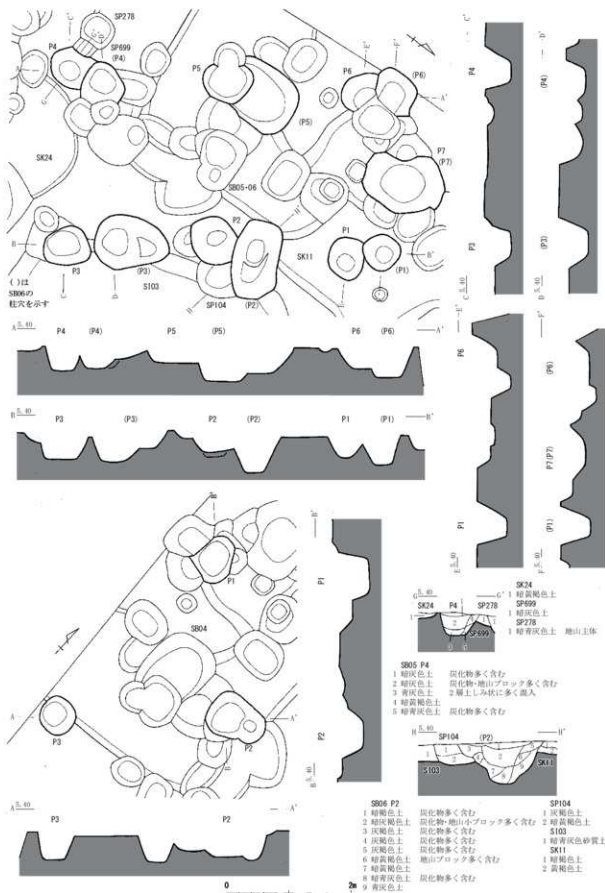
第53図 SB04-06 実測図 (縮尺 1/60)
