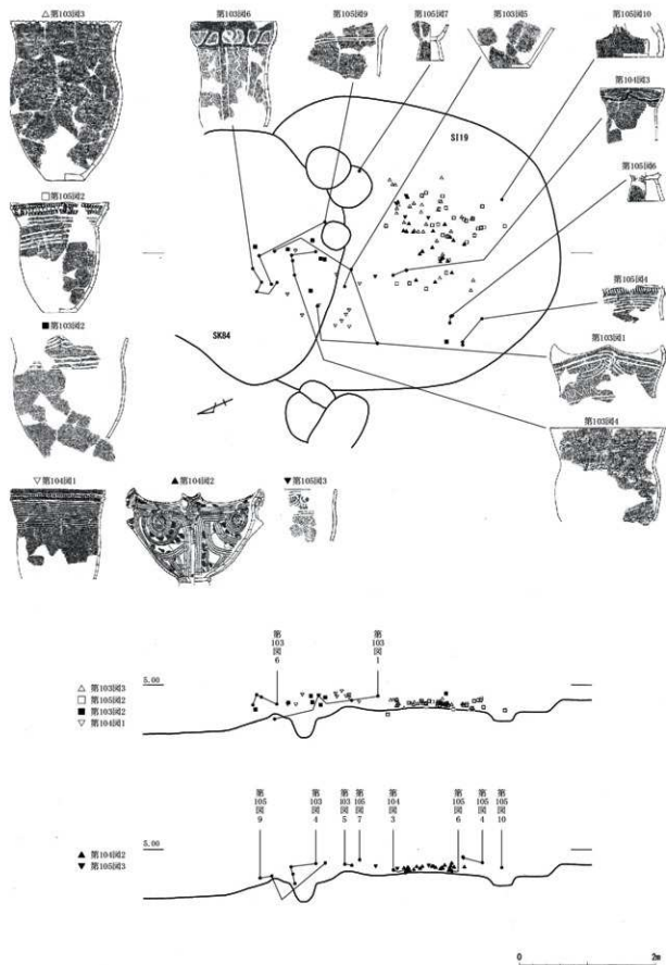
第46図 SI19 遺物出土状況図1 (縮尺 1/60)
