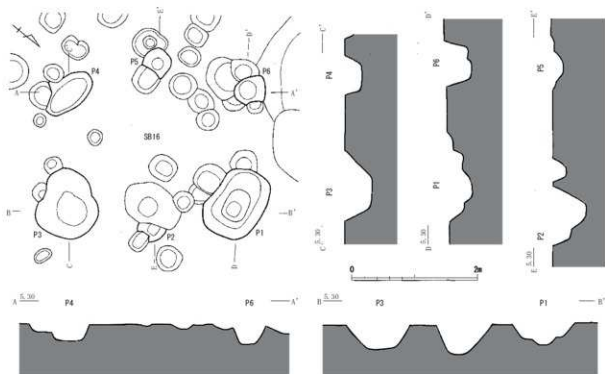
第60図 SB16実測図(縮尺1/60)
