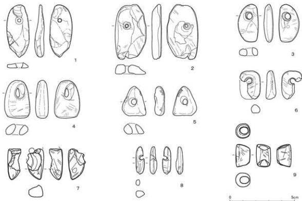
第159図 玉類実測図（縮尺2/3）
