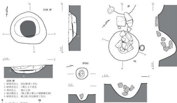
第10図 S104 跡 ・柱穴実測図（縮尺1/30）
