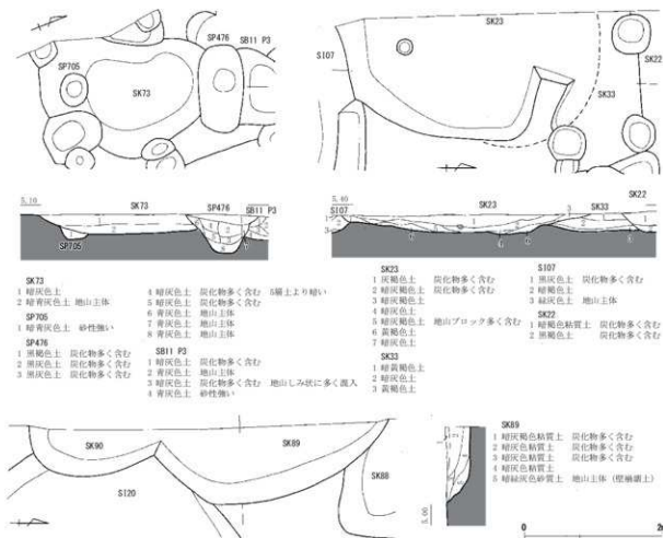
第65図 土坑実測図2 (縮尺 1/60)
