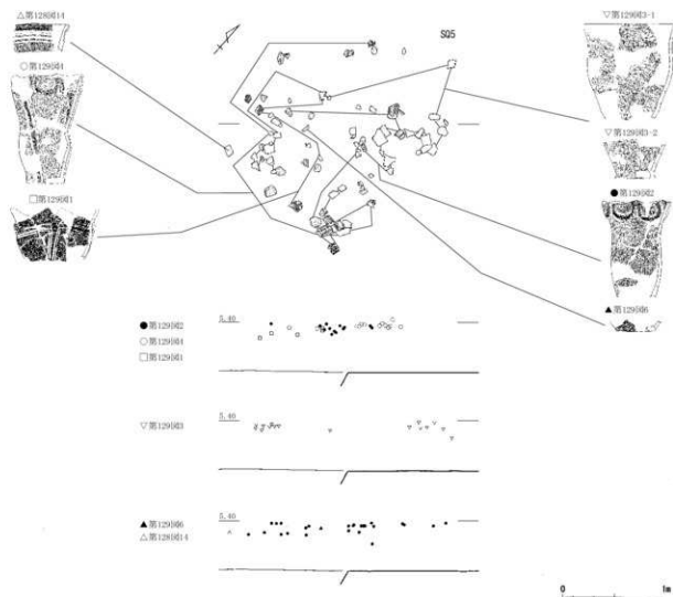
第75図 SQ 5 遺物出土状況図 (縮尺 1/40)
