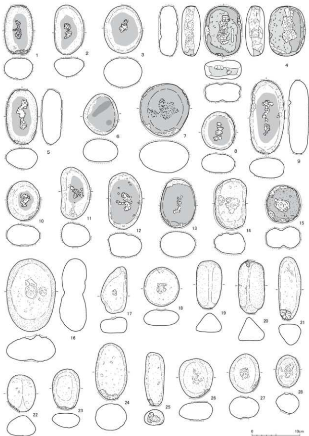
第155図 磨石類実測図2 (縮尺 1/4)
