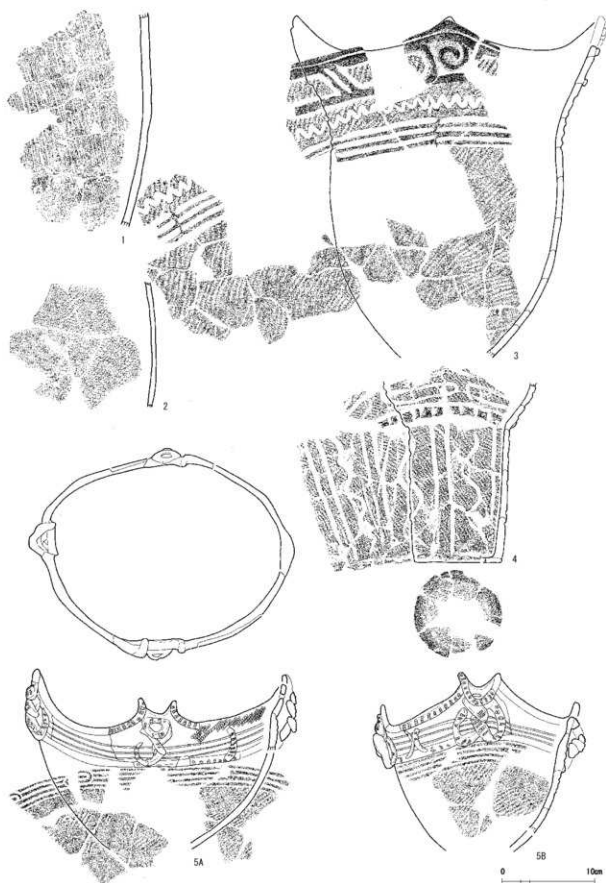
第83図 S105出土土器実測図（縮尺1/4）
