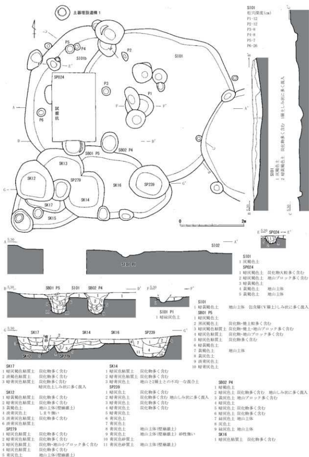
第7図 SI01 実測図(縮尺 1/60)
