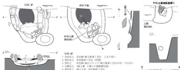
第15図 S105 炉・柱穴実測図（縮尺 1/30）
