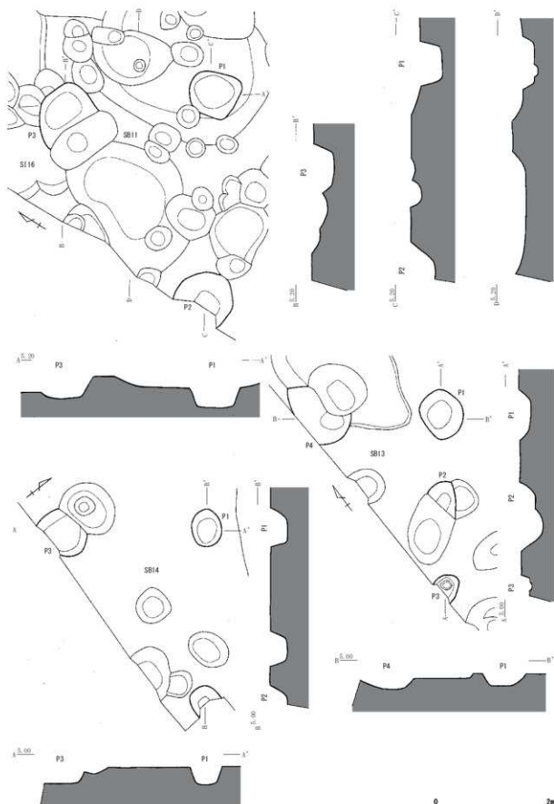
第59図 SB11・13・14実測図(縮尺1/60)
