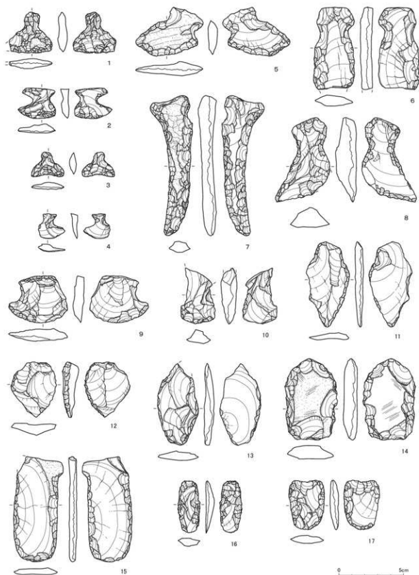
第144図 石匙・スクレイパー類実測図（縮尺1/2）
