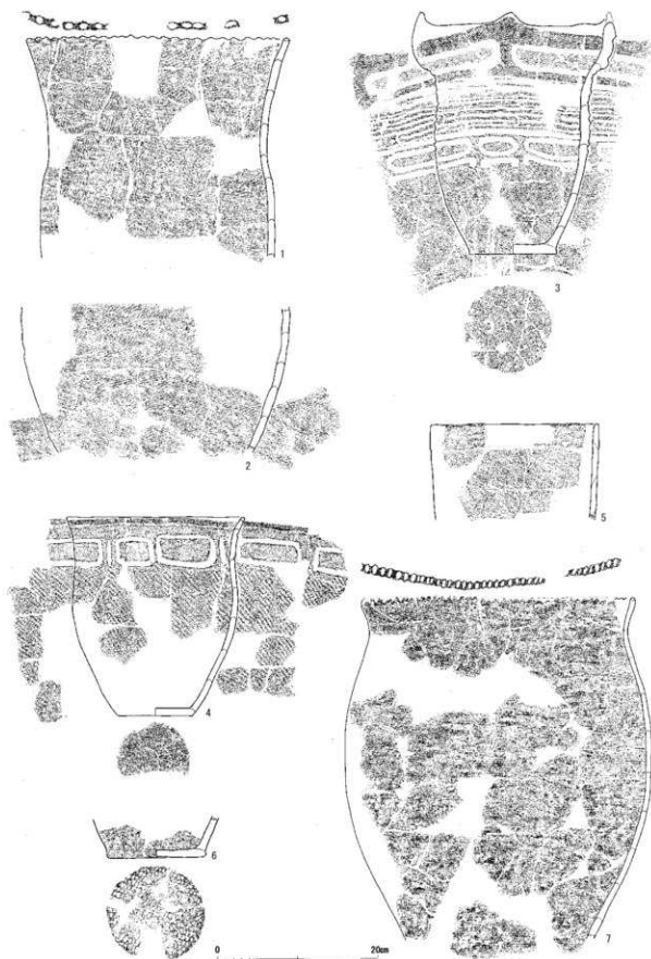
第91図 SI14出土土器実測図（縮尺 1/5）
