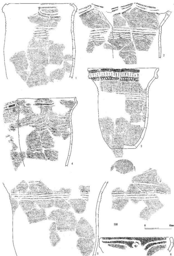
第130図 遺物集中域出土土器実測図4 (縮尺 1/4)
