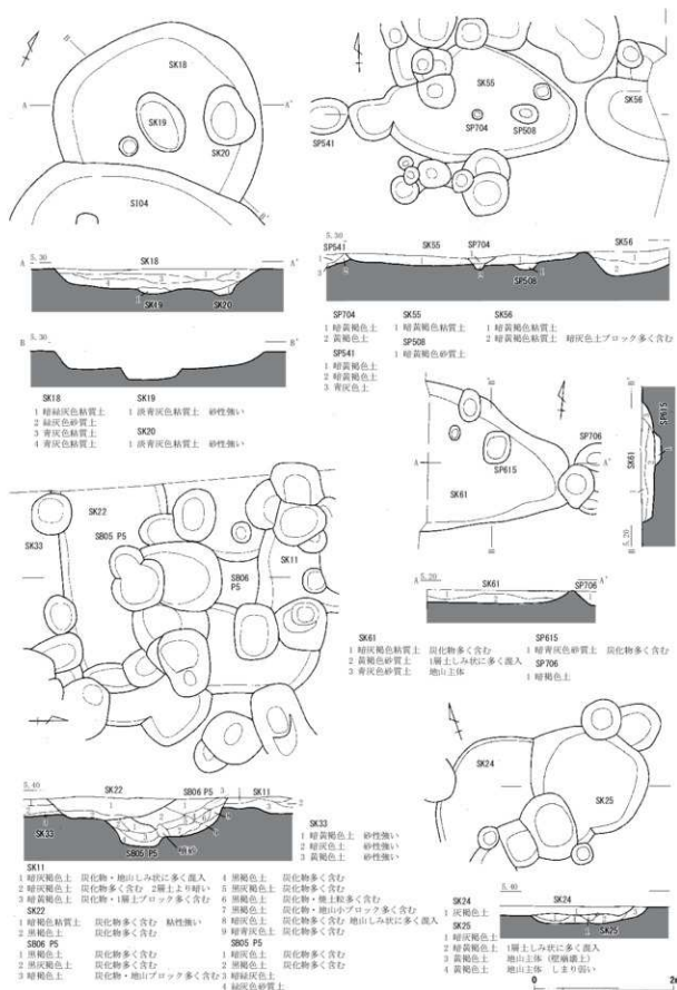
第66圖 土坑実測図3 (縮尺 1/60)
