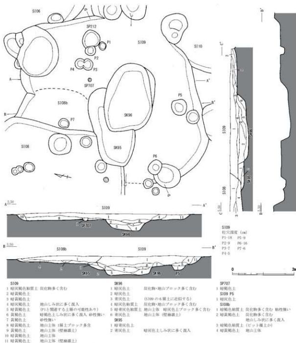
第25図 S109 実測図 (縮尺 1/60)
