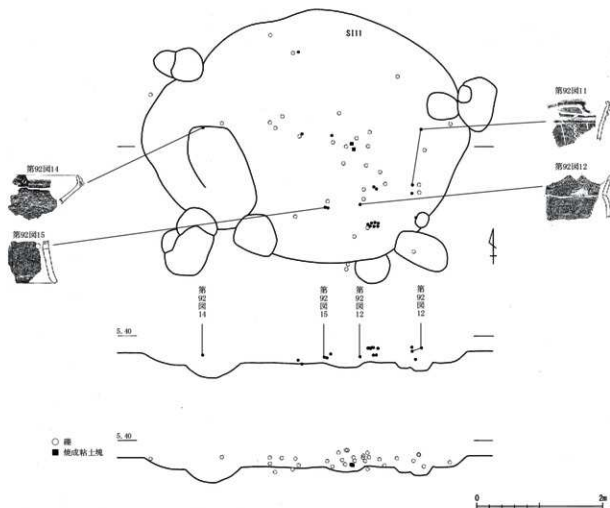
第31図 SI11 遺物出土状況図(縮尺1/60)
