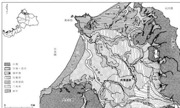
第2図 周辺の地形図（縮尺 1/200,000）
