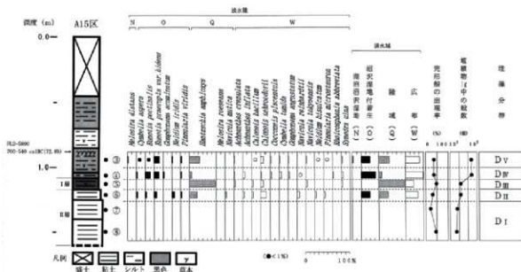
第169図 A15区における珪藻化石分布図 (2%以上の分類群を表示)
