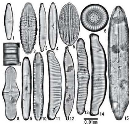
第169図 A15区における珪藻化石分布図 (2%以上の分類群を表示)
