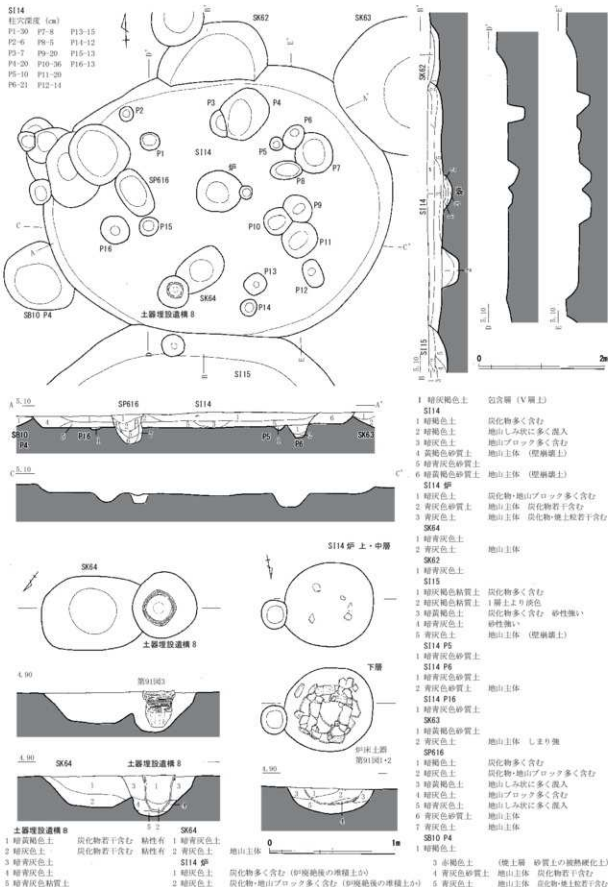
第33図 SI14 実測図 (縮尺 1/60・1/30)
