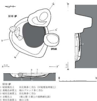
第27図 S110 炉実測図 (縮尺 1/30)
