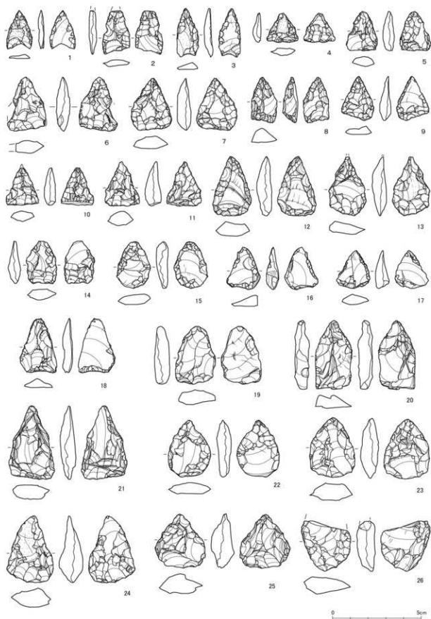
第142図 石鑑実測図4 (縮尺 2/3)
