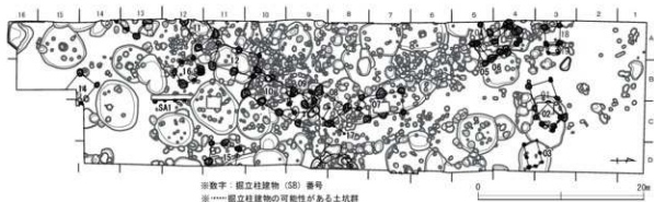
第51図 掘立柱建物・柱穴列配置図（縮尺 1/500）
