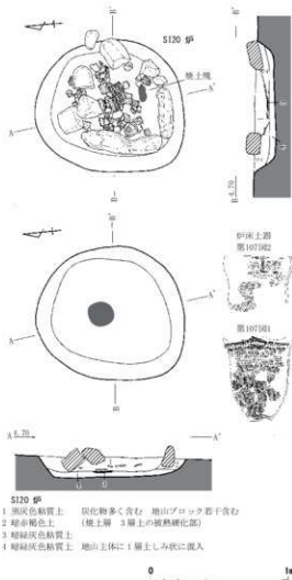
第49図 SI20 炉実測図(縮尺1/30)
