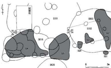
第72図 落ち込み実測図(縮尺1/60)
