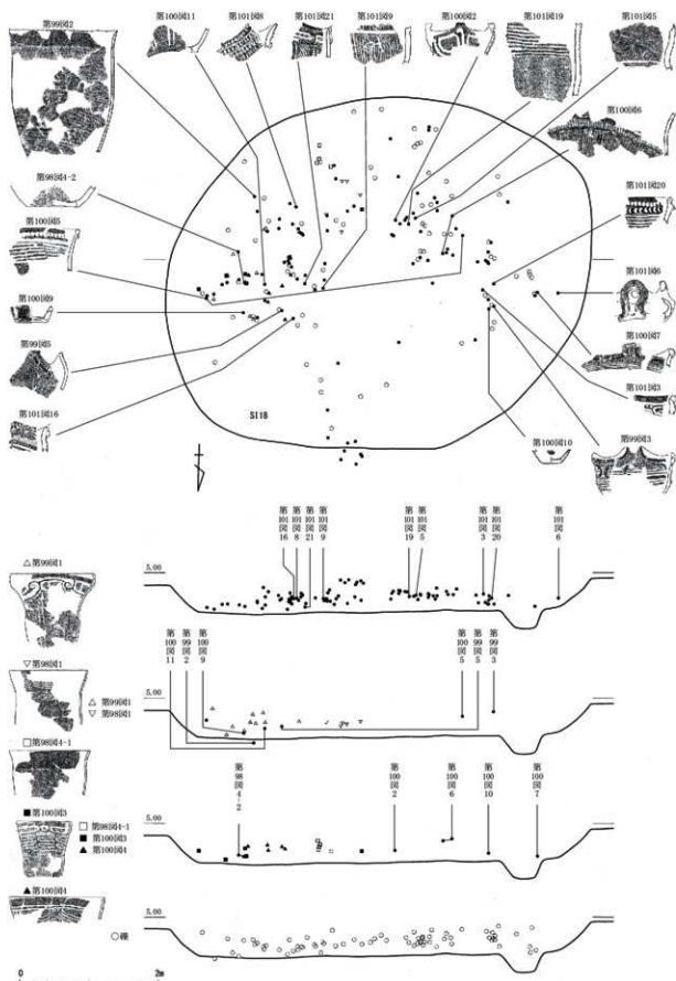
第44図 S118 遺物出土状況図 (縮尺 1/60)
