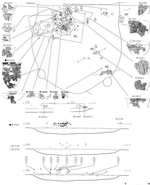
第74図 SQ 1～4 遺物出土状況図（縮尺 1/40）
