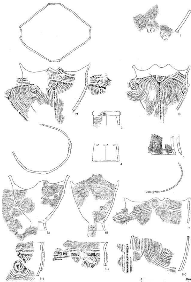
第80図 S104出土土器実測図2 (縮尺 1/5)
