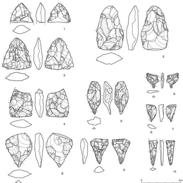
第143図 石鏃・石錐実測図（縮尺2/3）
