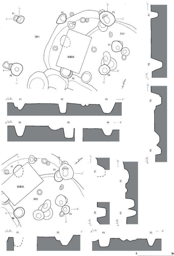
第52図 SB01・02 実測図 (縮尺 1/60)
