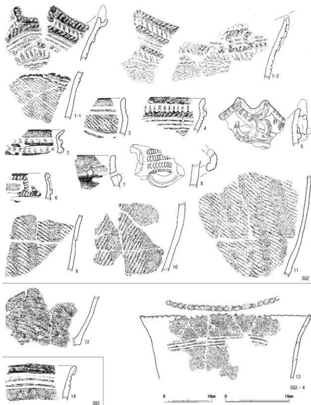
第128図 遺物集中城出土土器実測図2 (縮尺 1/4 : 12・13 1/3 : その他)
