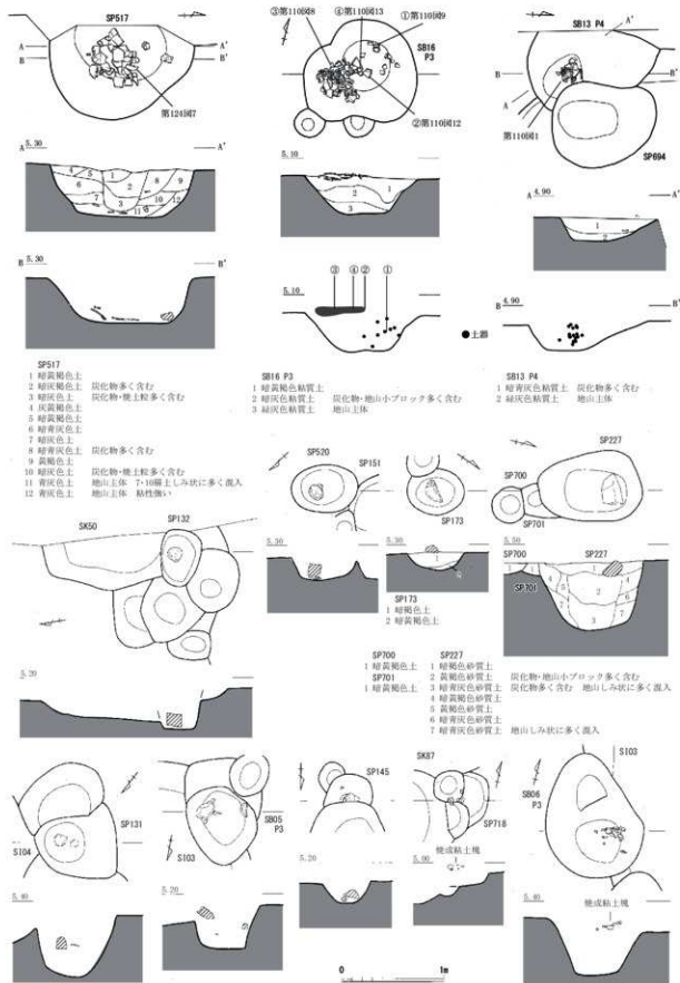
第71圖 柱穴実測図2 (縮尺 1/40)
