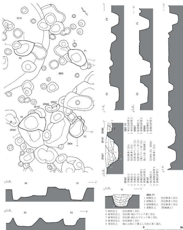
第55図 SB08 実測図 (縮尺 1/60)
