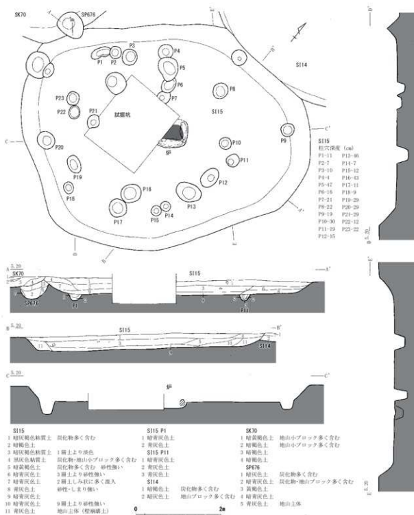
第36図 SI15 実測図 (縮尺 1/60)
