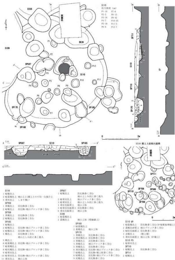
第28図 SI10 実測図 (縮尺 1/100・1/60)
