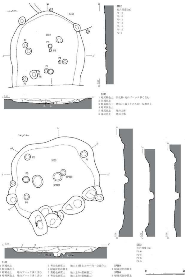
第8図 S102・03 実測図 (縮尺 1/60)
