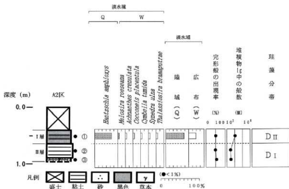
第168図 A2区における珪藻化石分布図（4%以上の分類群を表示）
