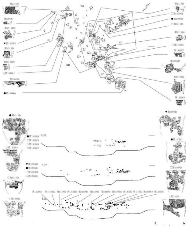
第76図 SQ 6 遺物出土状況図 (縮尺 1/40)
