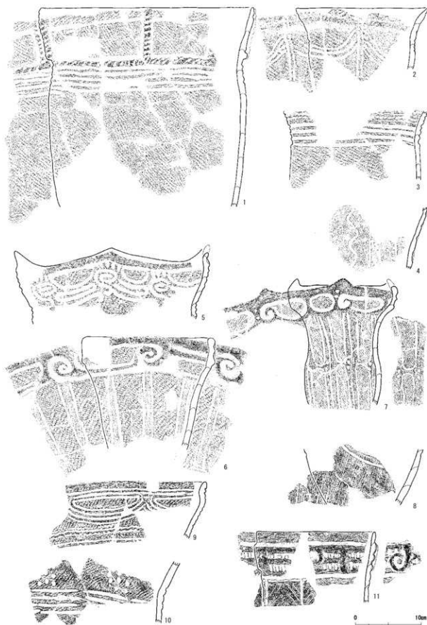
第85図 S107出土土器実測図1 (縮尺1/4)
