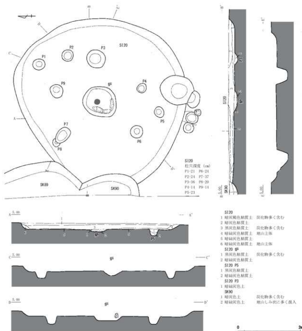
第48図 S120 実測図 (縮尺 1/60)
