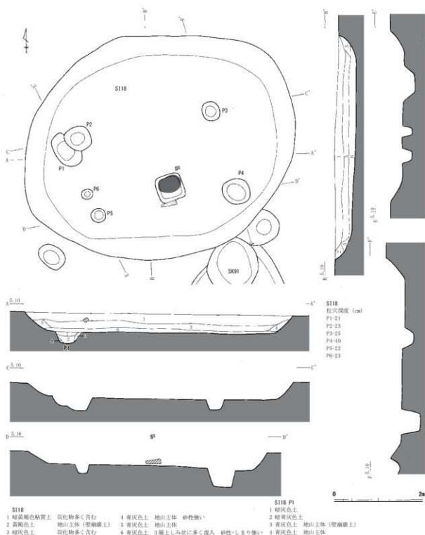
第42図 S118 実測図（縮尺 1/60）
