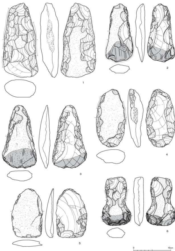
第150図 打製石斧実測図5 (縮尺 1/3)
