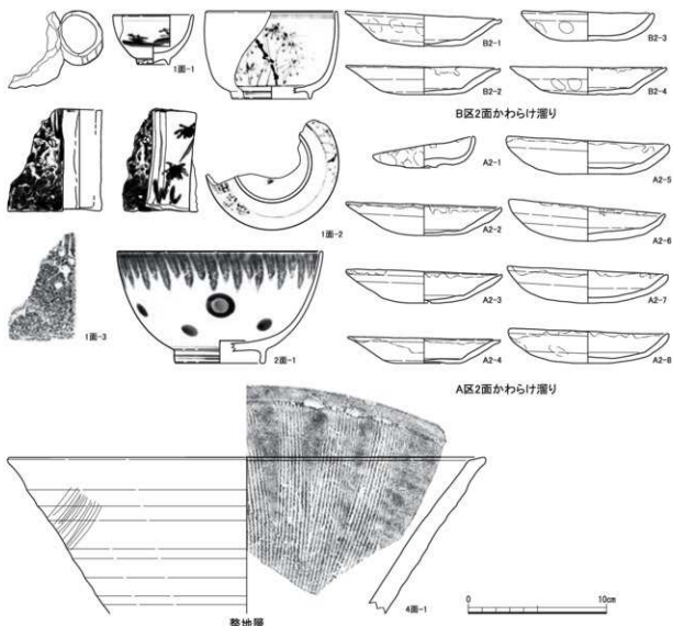
第19図 土器・陶磁器実測図3 (縮尺1/3)
