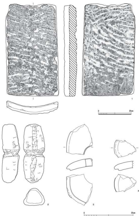
第22図 石製品実測図(2～4：縮尺1/4 1：縮尺1/6)
