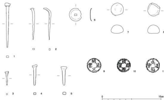
第23図 金属製品実測図(縮尺1/2)
