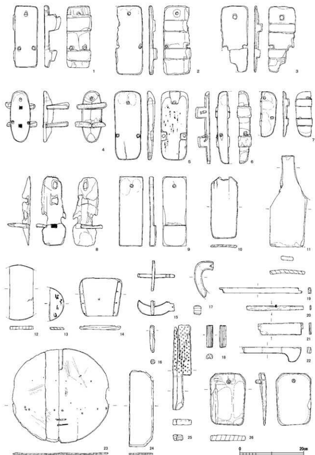
第21図 木製品実測図2 (縮尺1/6)
