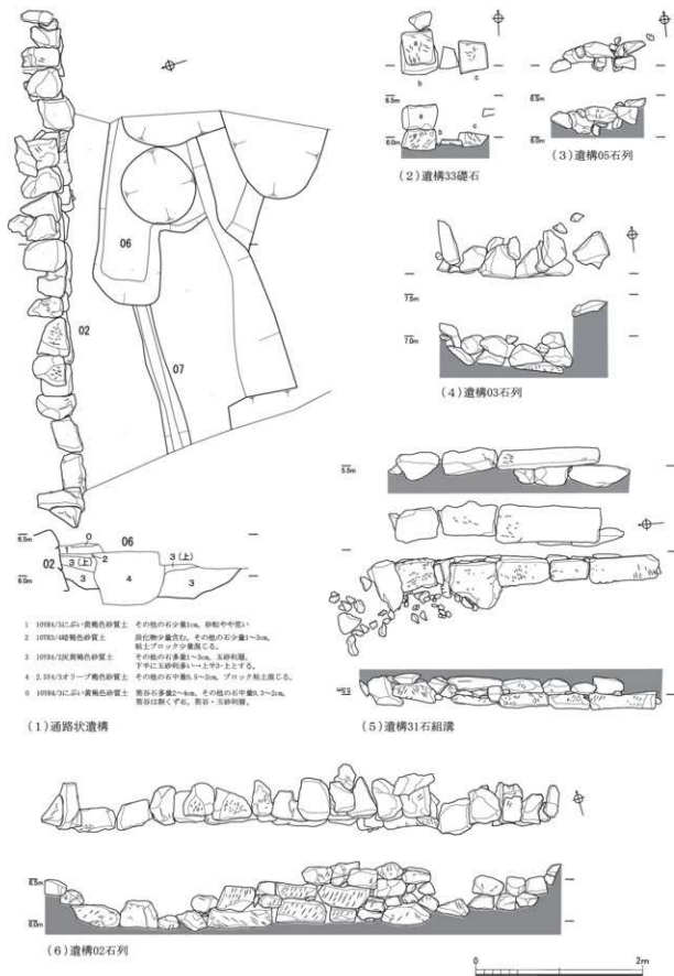
第12図 A区遺構図(縮尺1/50)
