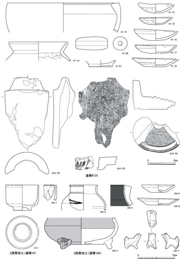
第18図 土器・陶磁器実測図2 (縮尺1/3 ☆印: 縮尺1/4)
