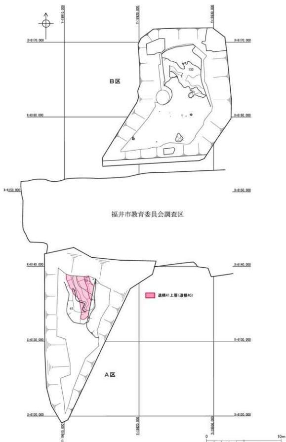
第9圖 6面遺構配置図(縮尺1/250)
