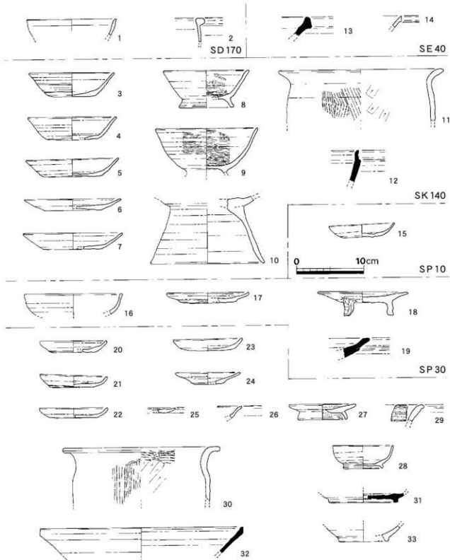
第19図 出土遺物実測図 (1/4)
