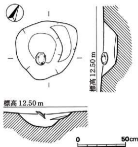
第18図 SP 30実測図 (1/20)
