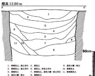
第13図 SE 40土層断面図(1/20)
