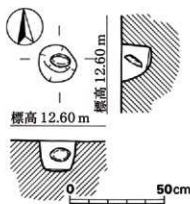
第15図 SP 10実測図 (1/20)
