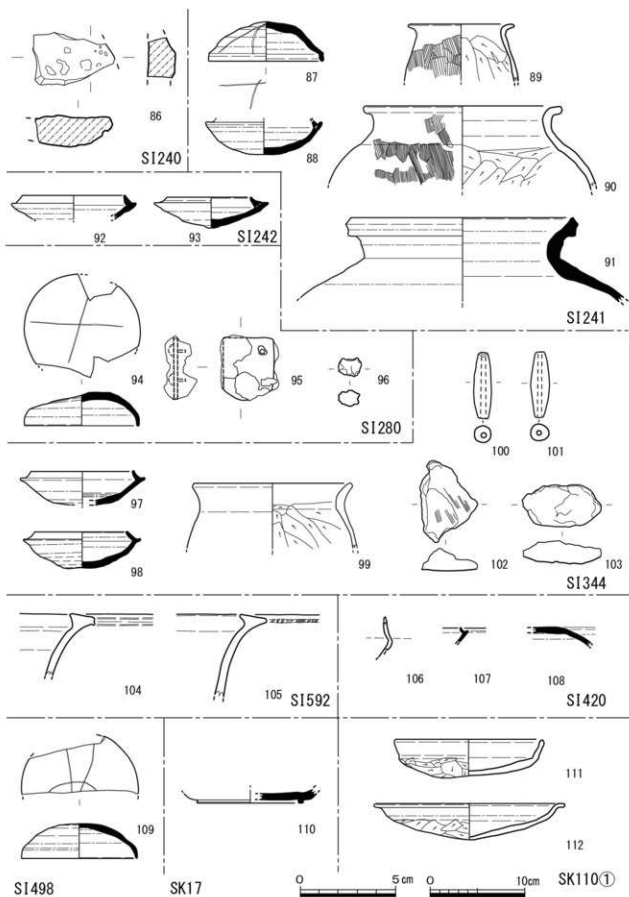
第22図 出土遺物実測図 (1/2・1/4)
