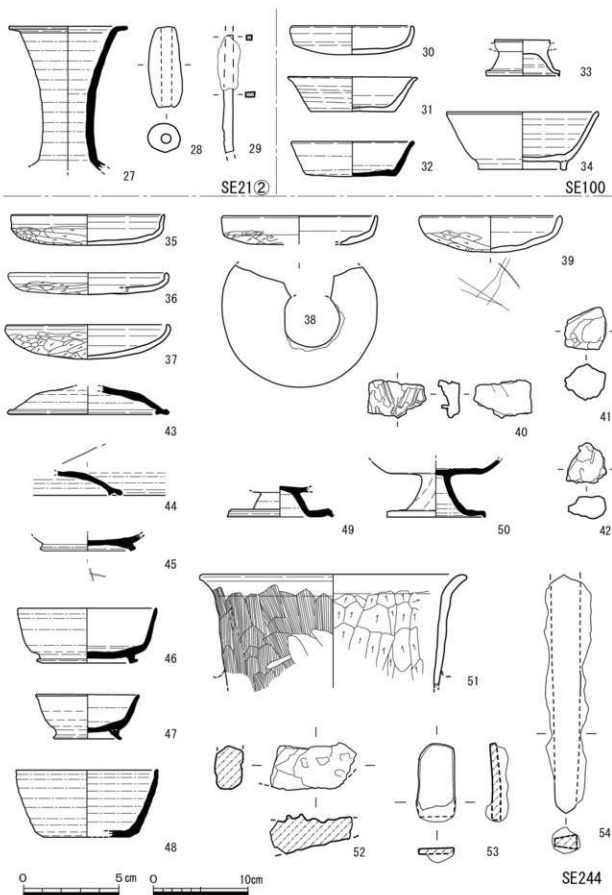
第20図 出土遺物実測図 (1/2・1/4)
