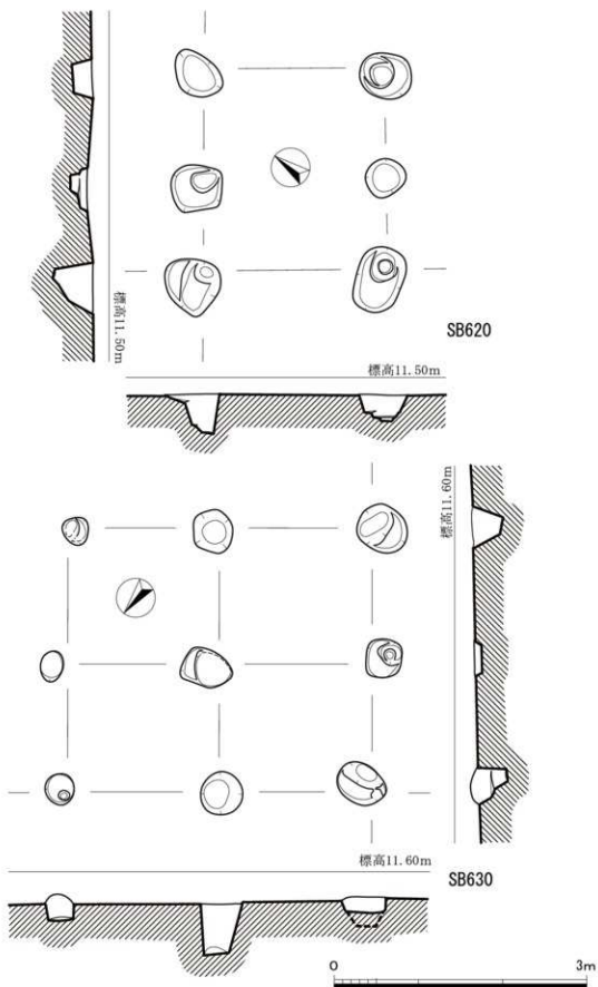
第6図 SB620・SB630実測図 (1/50)
