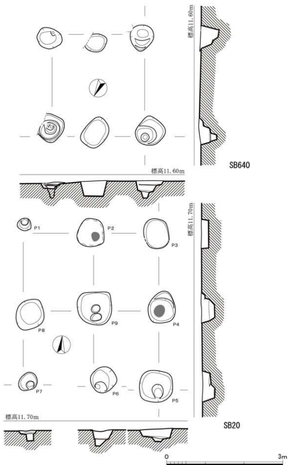
第7圖 SB640・SB20実測図 (1/50)
