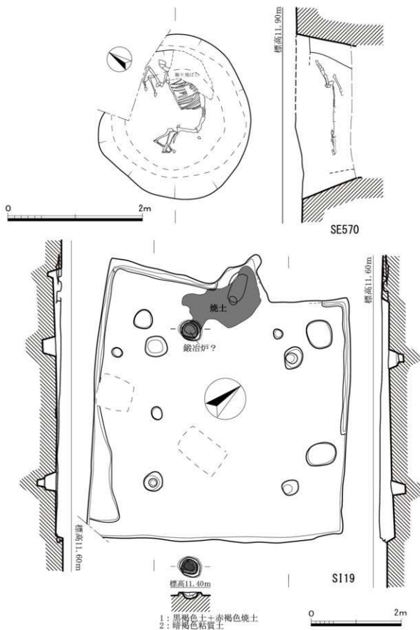
第13図 SE570・SE582・S119実測図 (1/40・1/60)
