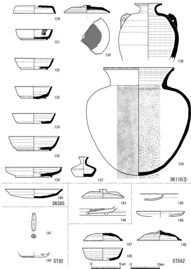
第24図 出土遺物実測図 (1/2・1/4)
