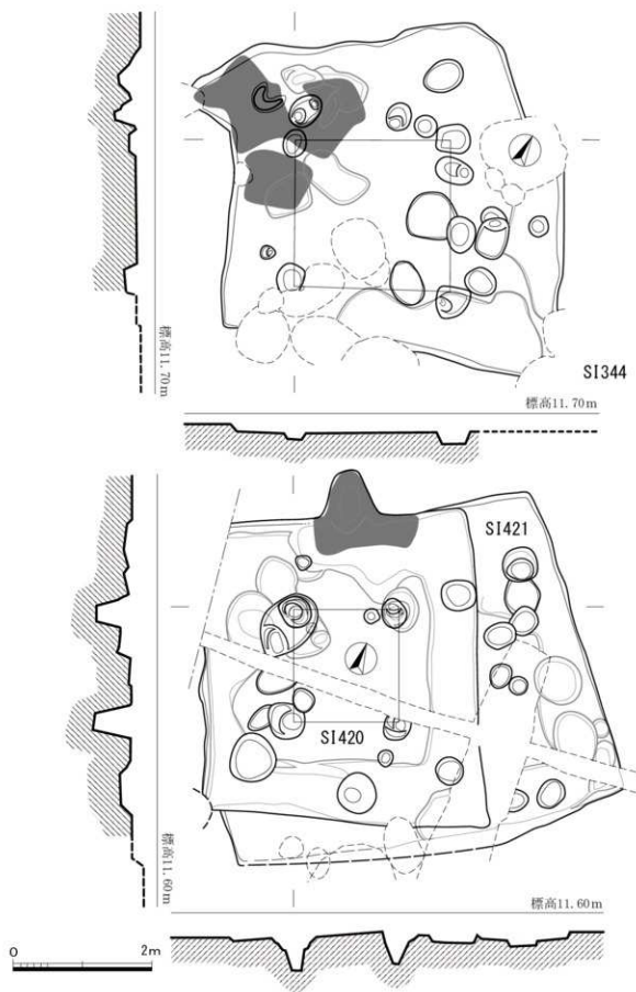
第15図 SI344・SI420・SI421実測図 (1/60)
