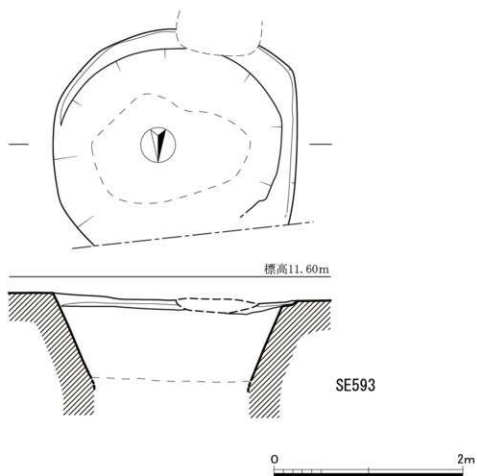
第8圖 SD13 · SD244 · SE593実測図 (1/20 · 1/40)
