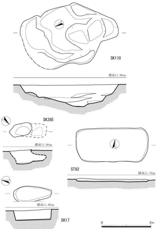
第17圖 SK110・SK385・SK17・ST92実測図 (1/40)
