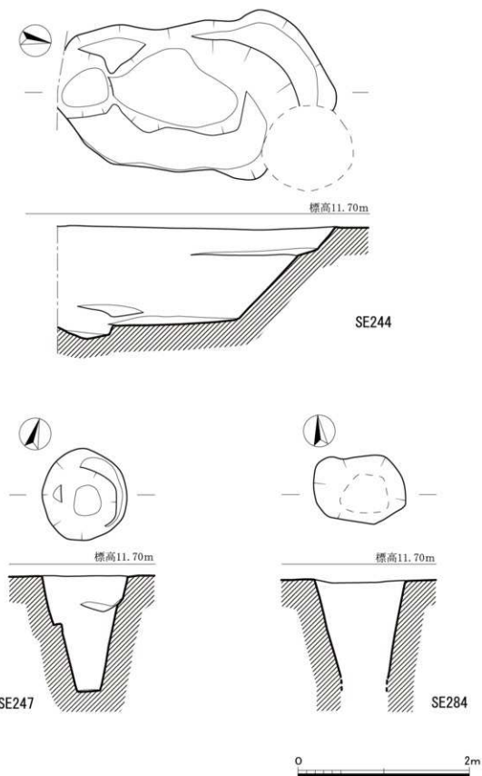
第10圖 SE244・SE247実測図 (1/40)
