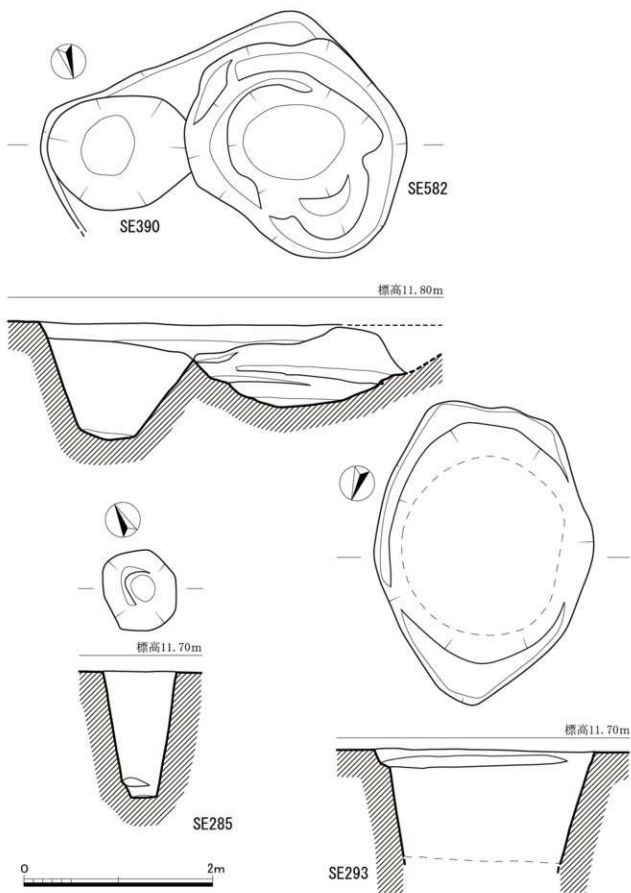
第11圖 SE390・SE582・SE285・SE293実測図 (1/40)
