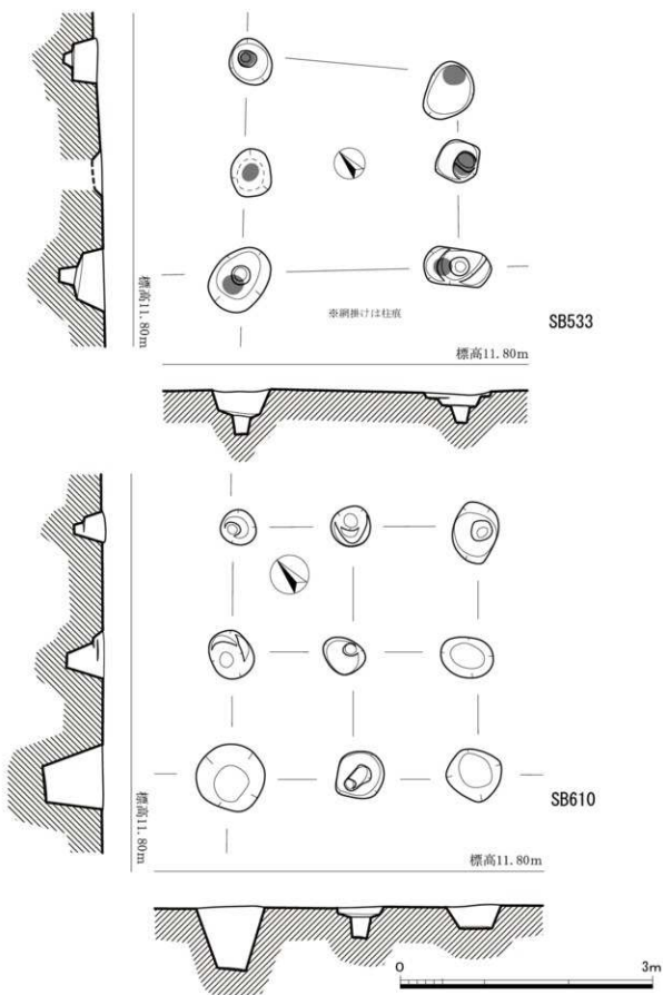
第5図 SB533・SB610実測図 (1/50)
