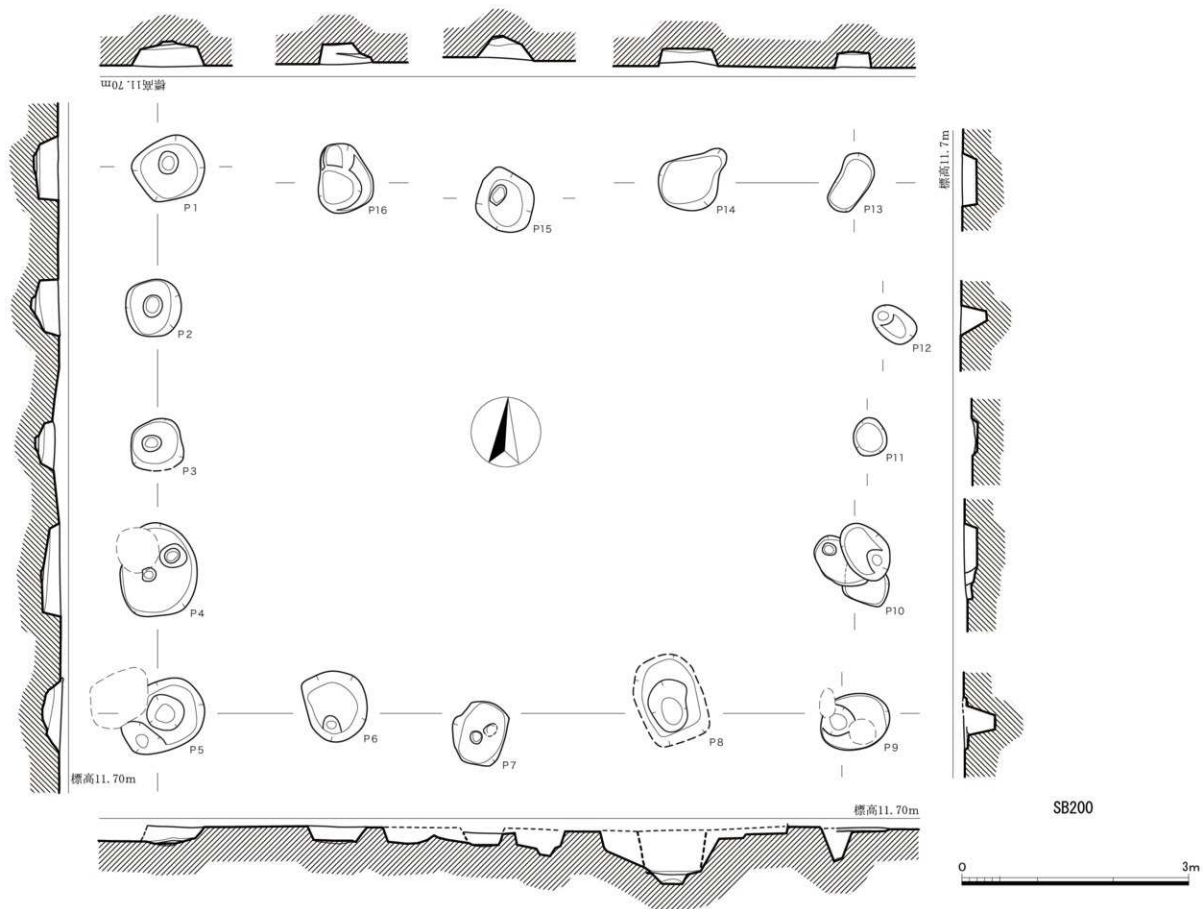
第12図 SB200実測図 (1/50)
