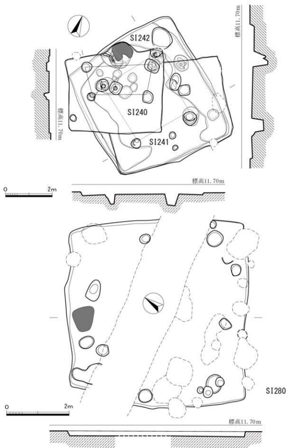
第14図 S1240・S1242・S1280実測図 (1/80・1/60)
