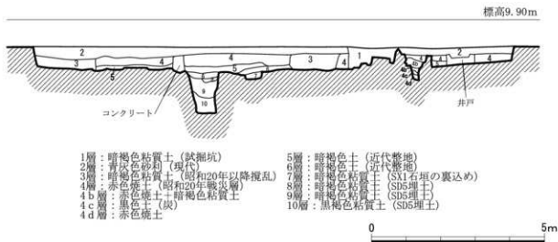
第7図 調査区南壁基本土層図（1/100）
