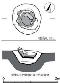
第5図 SX11実測図 (1/20)
