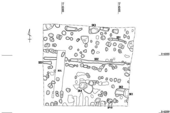
第3図 I区 遺構配置図 (S=1/100)
