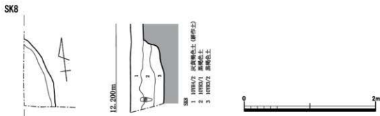
第 12 図 6・8号土坑 平・断面図 (S=1/40)
