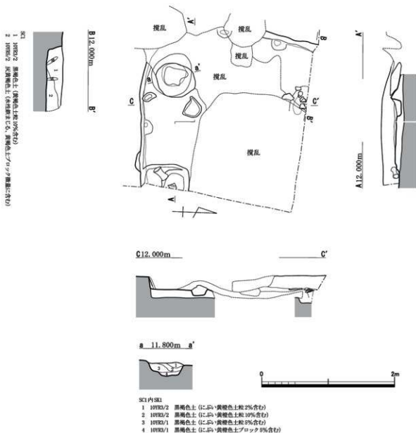
第 6 図 1 号住居 平・断面図 (S=1/40)
