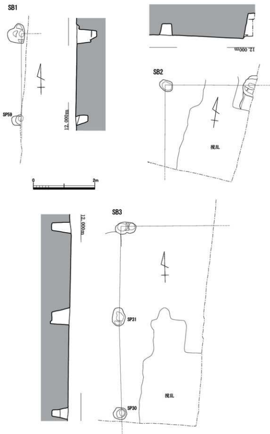
第9図 1～3号掘立柱建物 平・断面図 (S=1/60)
