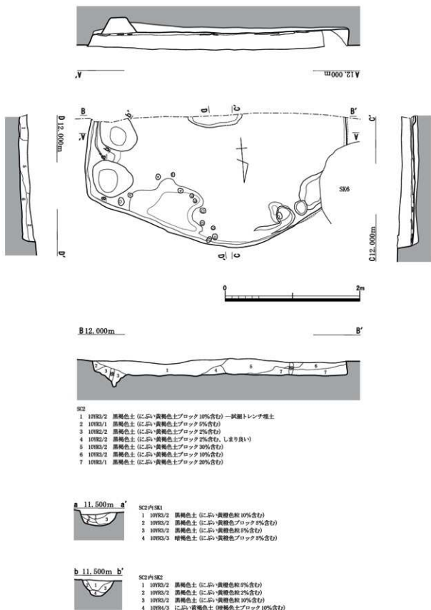
第7図 2号住居 平・断面図 (S=1/40)
