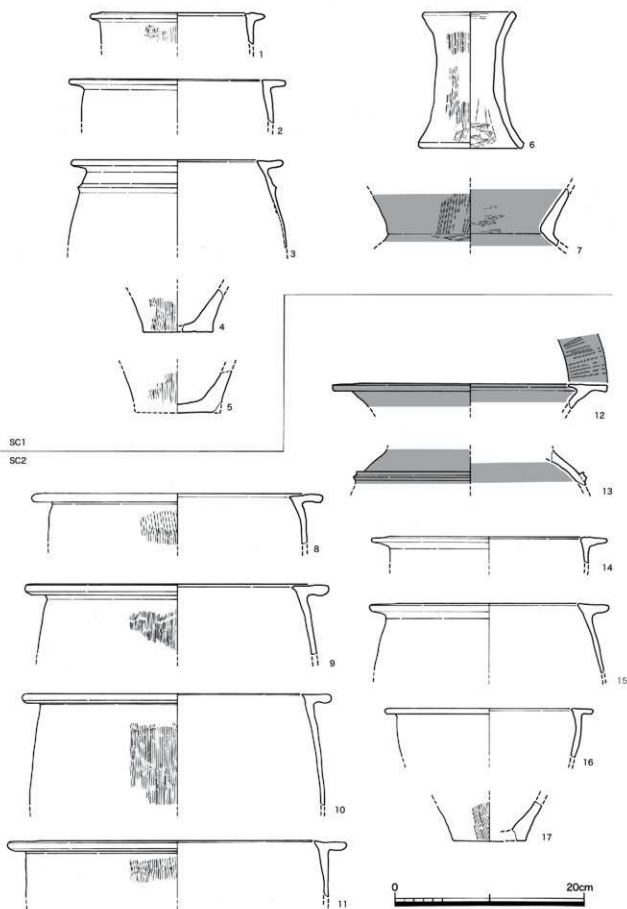
第8图 1·2号住居 出土遺物 (S=1/4)
