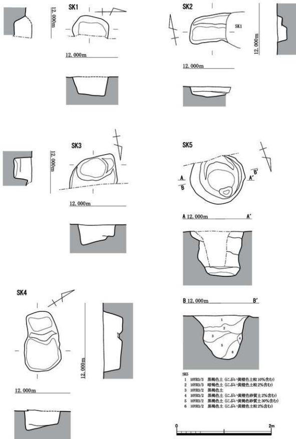
第 11 図 1～5 号土坑 平・断面図 (S=1/40)
