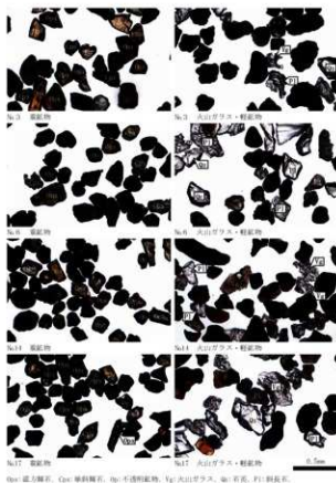
写真3 テフラ試料の顕微鏡写真(1)
