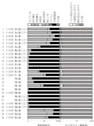
第26図 テフラ組成分析結果
