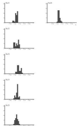
第 32 図 斜方輝石の屈折率測定結果 (3)
