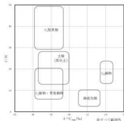
第40図 炭素安定同位体比とC/N比の関係 (1) [吉田・西田 (2009) に基づく]
