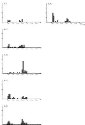
第 29 図 火山ガラスの屈折率測定結果 (3)
