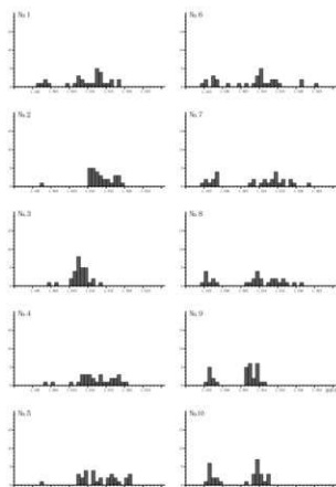
第27図 火山ガラスの屈折率測定結果(1)
