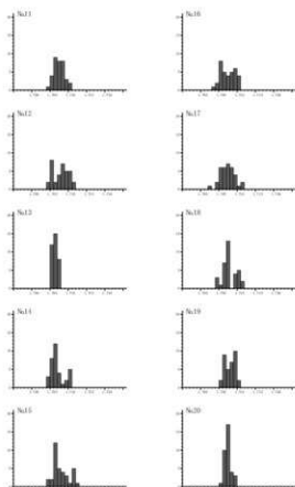
第 31 図 斜方輝石の屈折率測定結果 (2)
