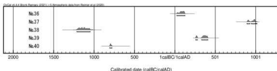
第37図 暦年校正年代マルチプロット図(2)
