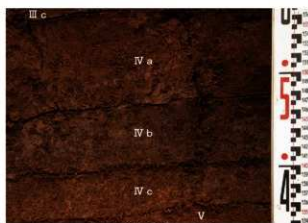
IV層の細分 (②のアップ)
