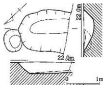
第94図 1号土坑実測図(1/60)
