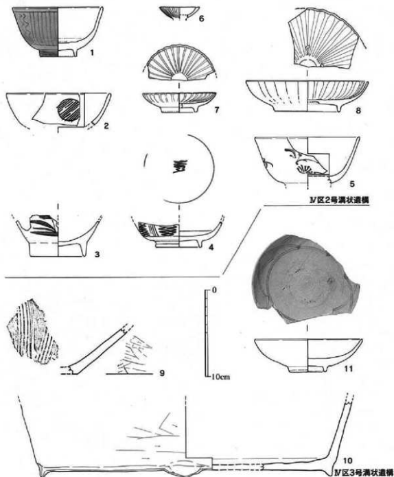
第64図 IV区2・3号溝状遺構出土物実測図(1/3)
