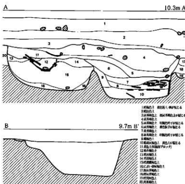
第26図 Ⅱ区5～8号土坑実測図(1/30)
