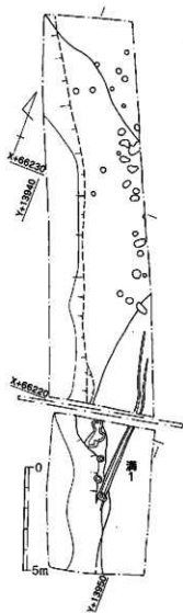
第96図 六郎神田遺跡 遺構配置図(1/200)
