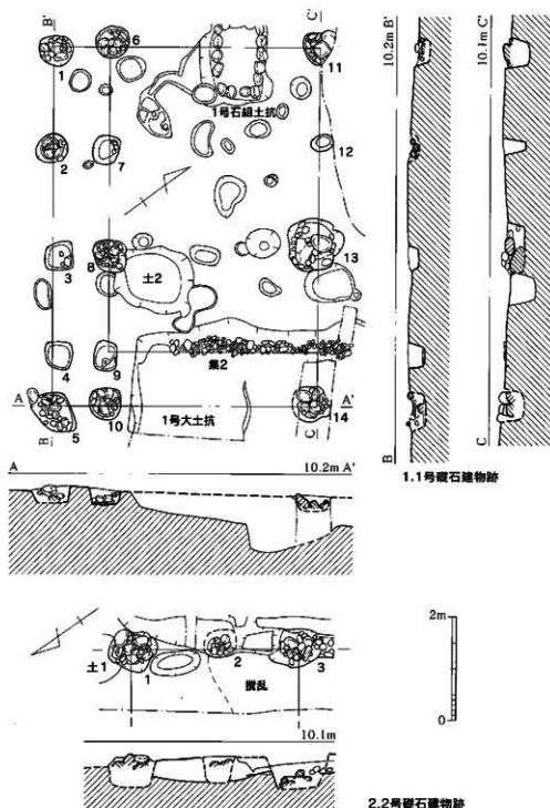
第4図 I区1・2号礎石建物跡実測図(1/80)
