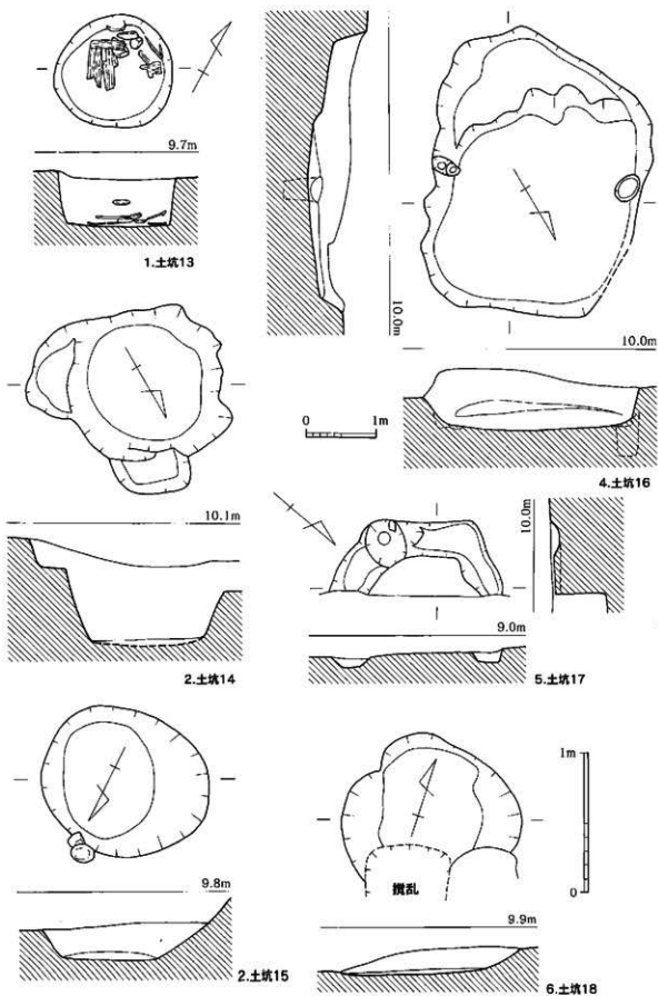
第54图 IV区13~18号土坑实测图(4是1/60, 他1/30)
