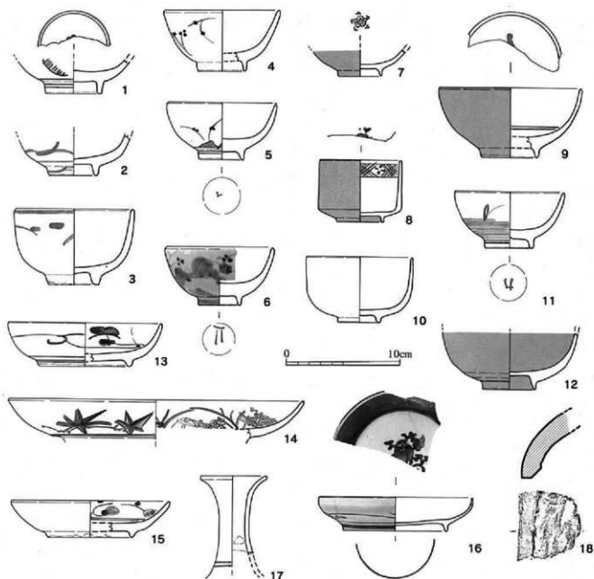
第37図 II区1号溝状遺構出土磁器・瓦実測図(1/3)
