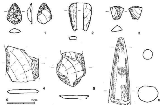
第100図 六郎坂木遺跡出土石製品実測図(1/2)
