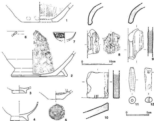
第13図 Ⅰ区1・2号大上坑出土陶磁器・瓦実測図(11・12は1/2、他は1/3)
