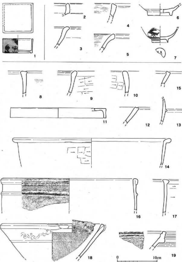
第66図 IV区6・7・9号溝状遺構出土物実測図(1/3)
