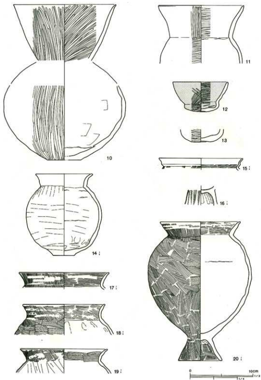
第32図 18号土坑出土遺物(2)
