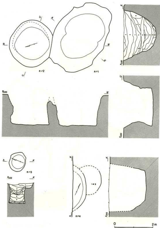
第20圖 中近世(I):井戸跡実測図
