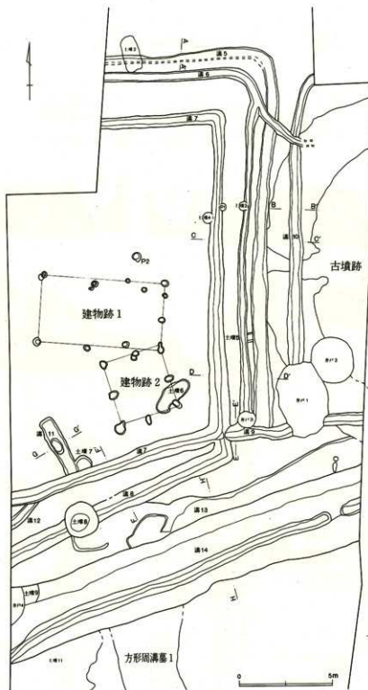
第12図 C区全測図・部分(2)
