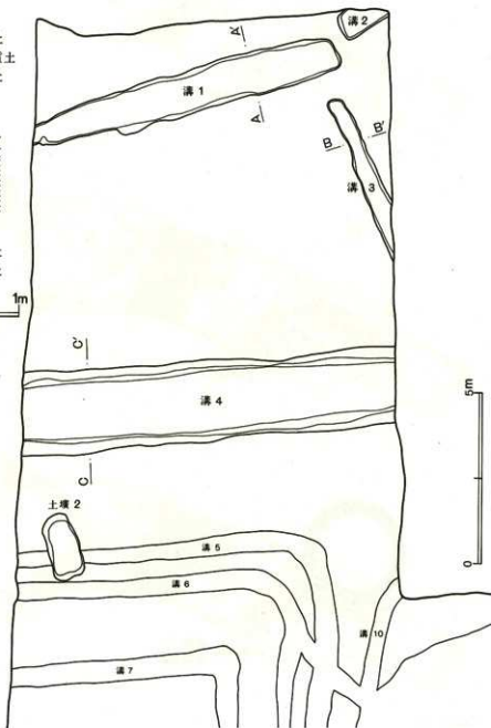
第11图 C区全测图・部分(1)
