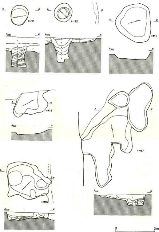
第19図 井戸跡・土城実測図：平安時代
