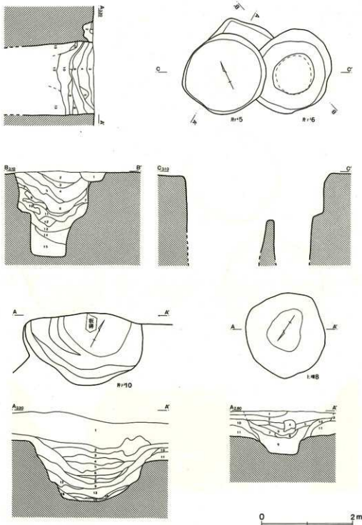
第21図 中近世(2)：井戸跡・土坑実測図
