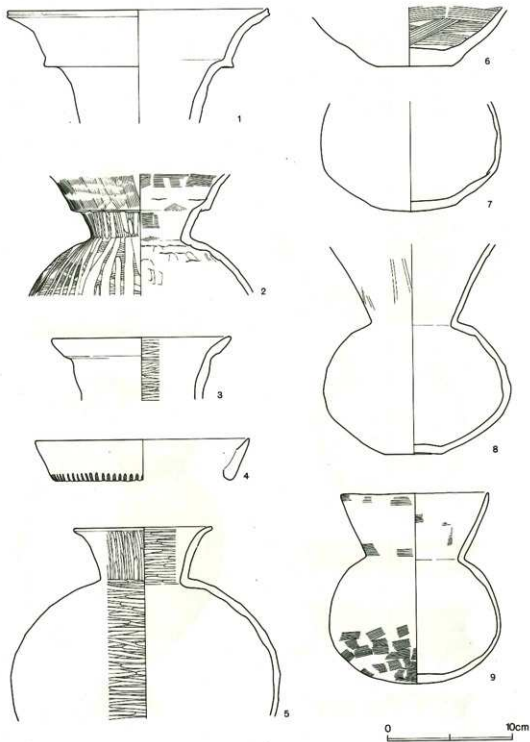
第31圖 18号土壙出土遺物(1)
