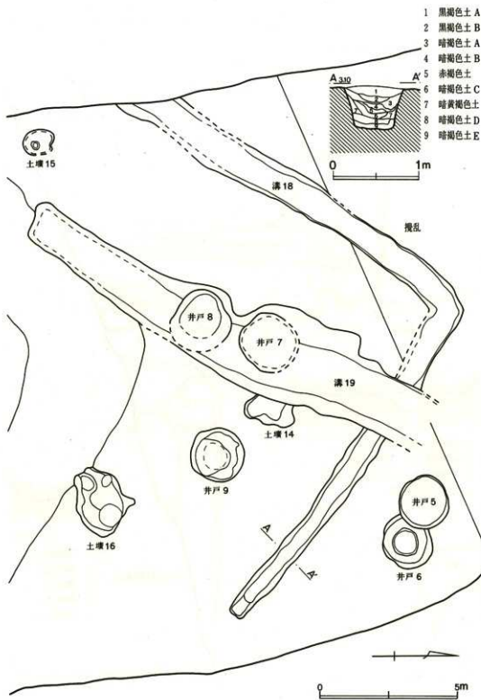
第15图 C区全测图・部分(4)
