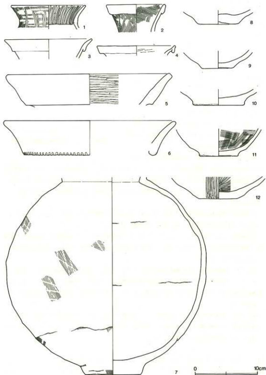
第29图 3号方形周葬墓出土遗物(1)
