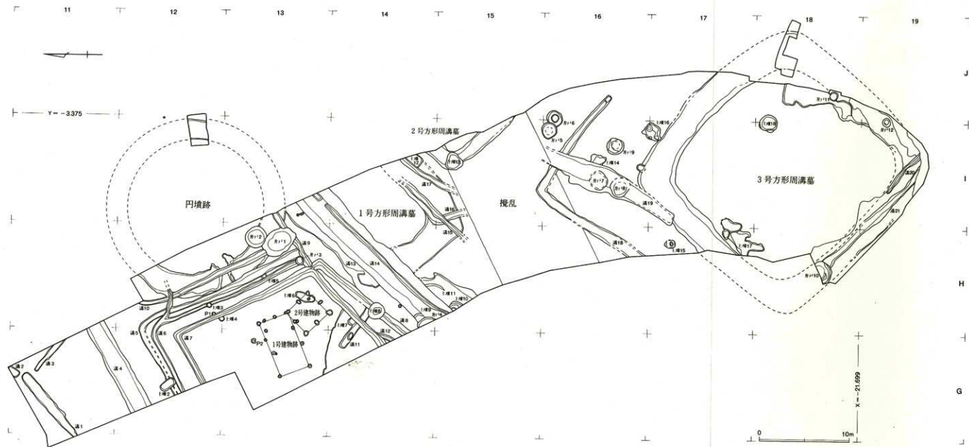
第5图 C区全测图
