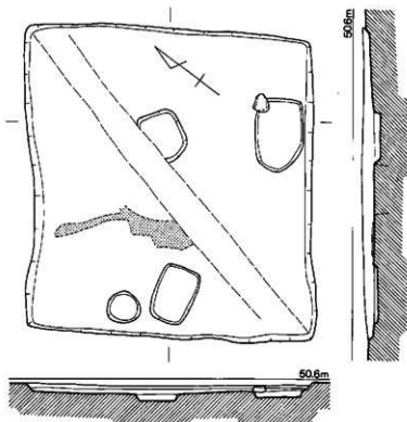
第26図 10号住居跡実測図 (1/60)
