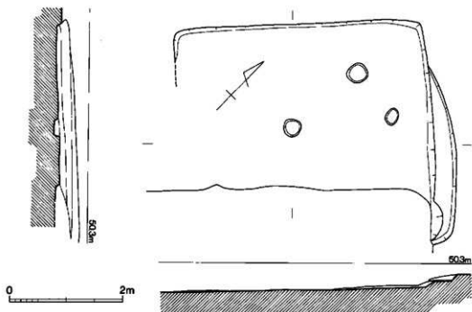
第32図 17号住居跡実測図 (1/60)
