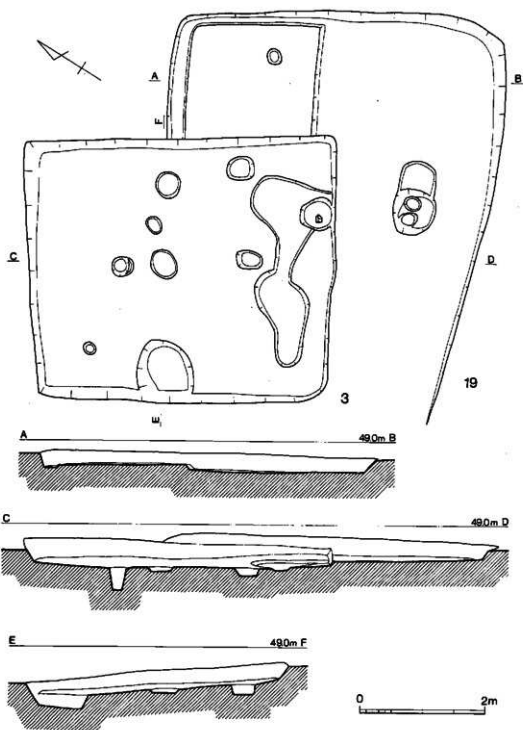
第20図 3・19号住居跡実測図 (1/60)
