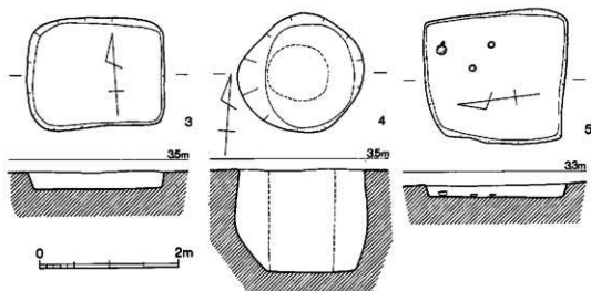
第4図 3・4・5号土坑実測図(1/60)
