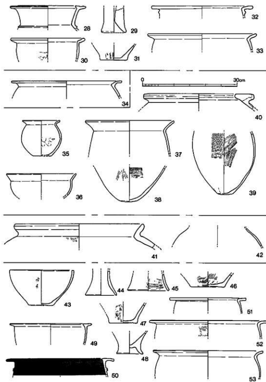
第36图 三船山遺跡6・7・8・10・11号住居跡出土土器実測図(1/6)
