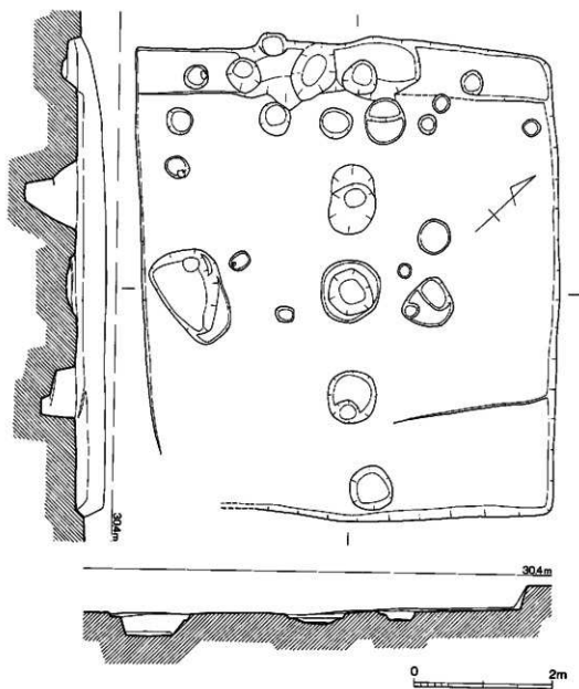
第31図 16号住居跡実測図 (1/60)
