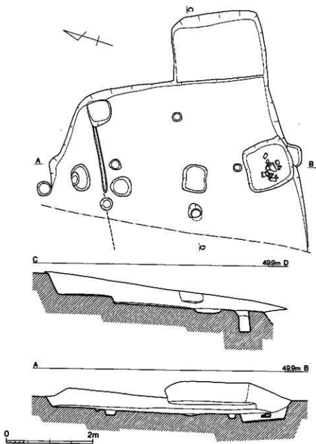
第33図 23号住居跡実測図 (1/60)
