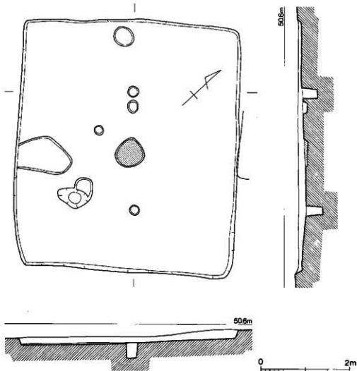
第28図 12号住居跡実測図 (1/60)
