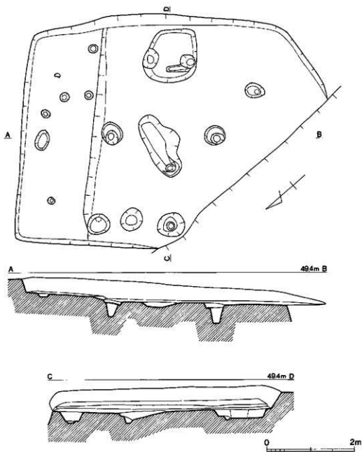
第23図 7号住居跡実測図 (1/60)
