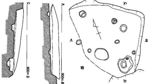
第27图 11・18号住居跡実測図 (1/60)
