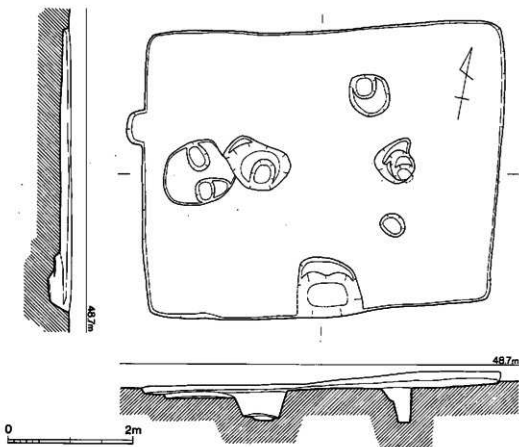
第18図 1号住居跡実測図 (1/60)
