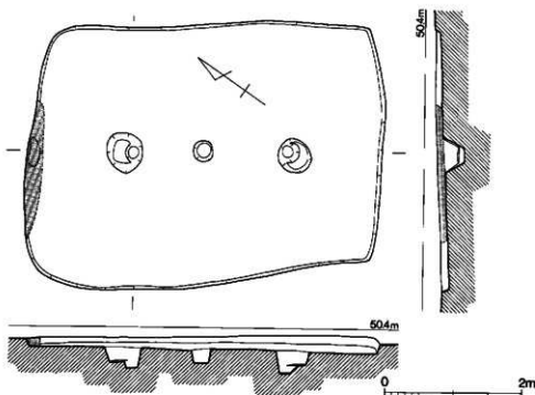
第29図 14号住居跡実測図 (1/60)
