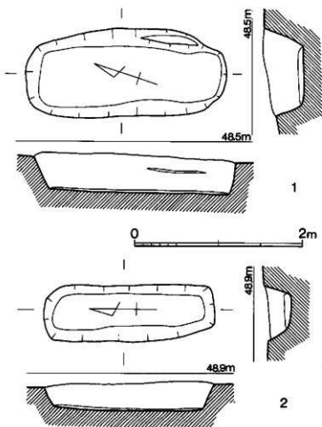
第34図 1・2号土墳墓実測図 (1/40)
