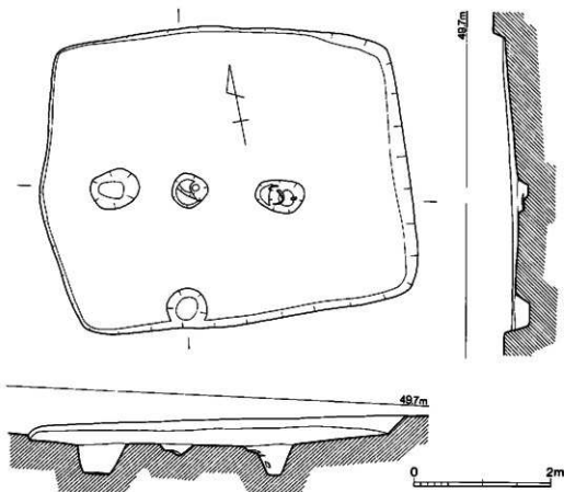
第24図 8号住居跡実測図 (1/60)
