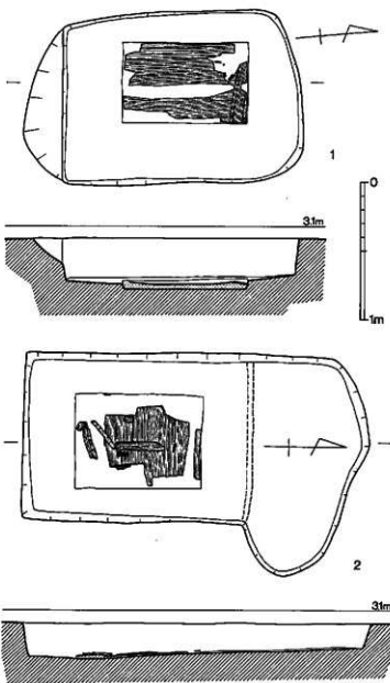
第3図 1・2号木棺墓実測図（1/30）
