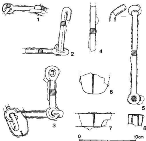
第12図 向野1・2号墳出土鉄器実測図(1/2)
