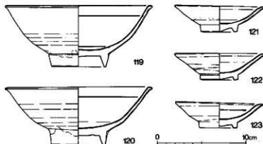
第41図 三船山遺跡出土白磁実測図（1/3）
