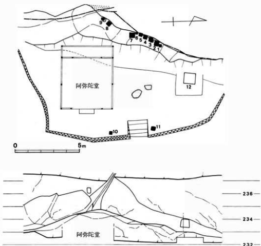
第1図 阿弥陀堂遺跡地形測量図
