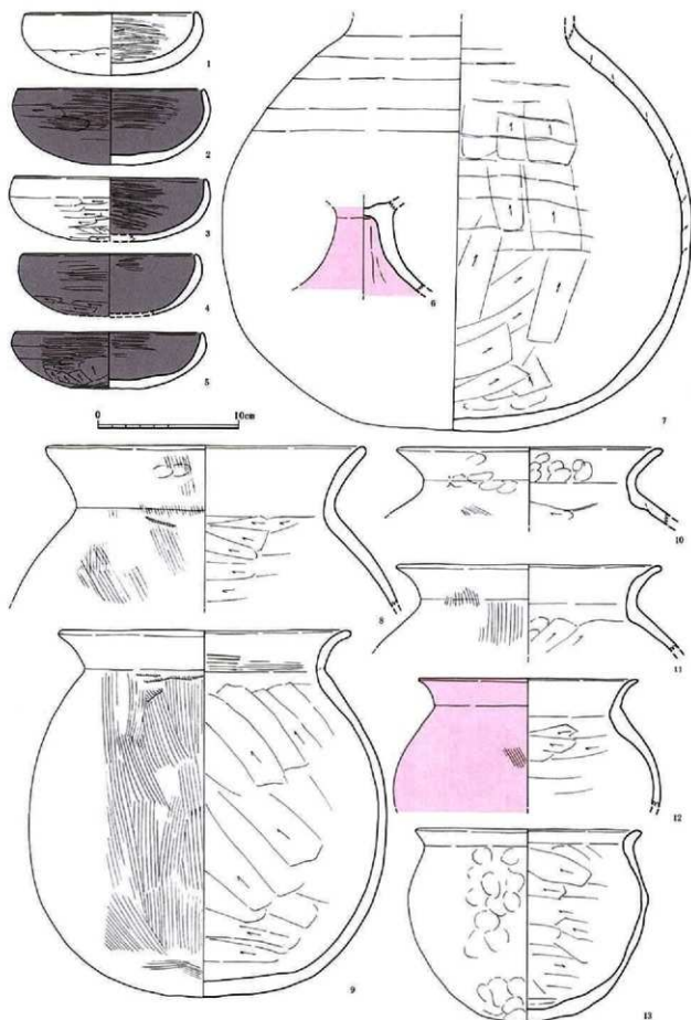
第 50 图 26 号竖穴住居跡出土土器実測图 (1) (1/3)
