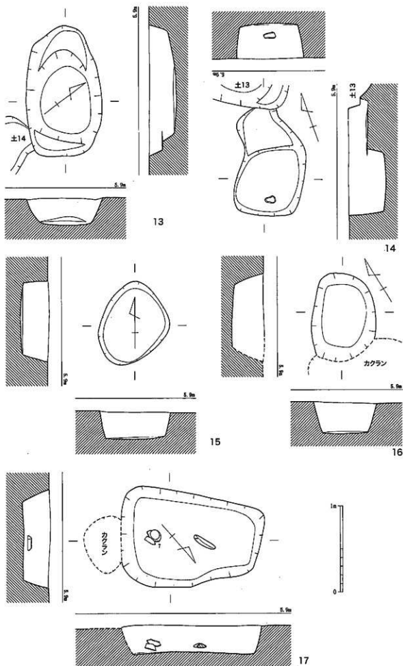
第77図 13～17号土坑実測図 (1/30)
