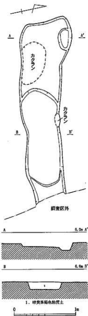
第84図 5号溝実測図 (1/30)
