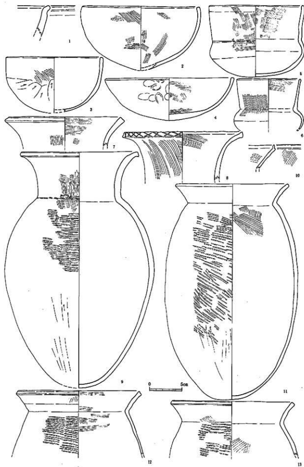
第 18 图 8 号竖穴住居跡出土土器実測図 (1) (1/3)
