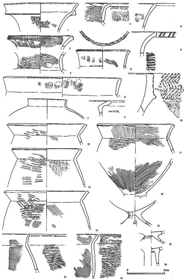
第41图 21号竖穴住居跡出土土器実測图(1)(1/3)
