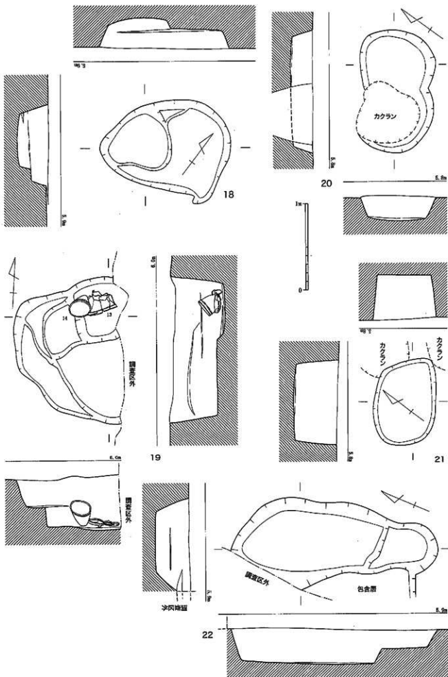
第 79 図 18～22 号土坑実測図 (1/30)
