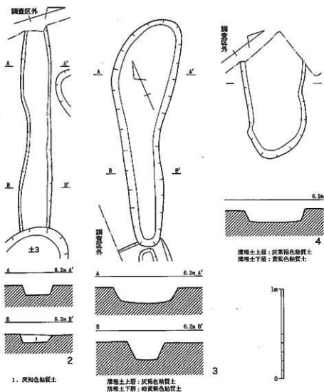
第70図 2~4号溝実測図(1/30)
