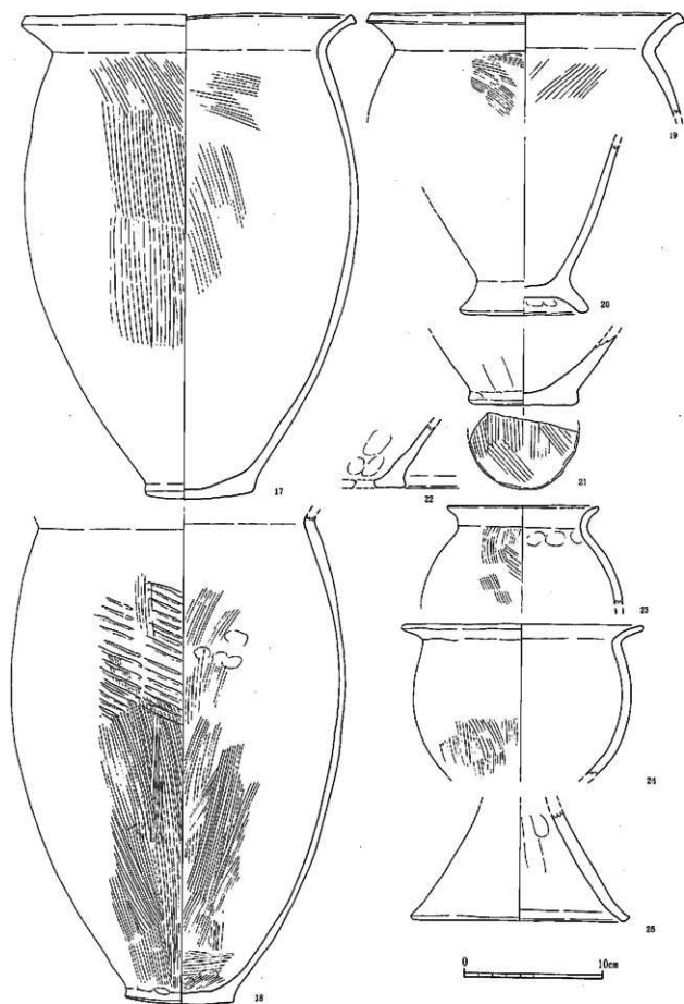
第30图 13号竖穴住居跡出土土器実測図(3)(1/3)
