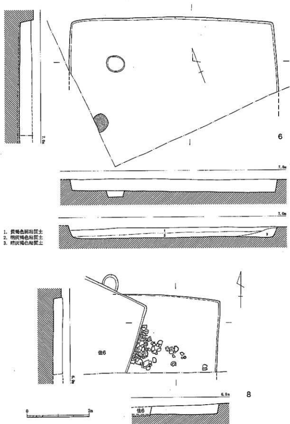
第17图 6・8号竖穴住居跡実測図 (1/60)
