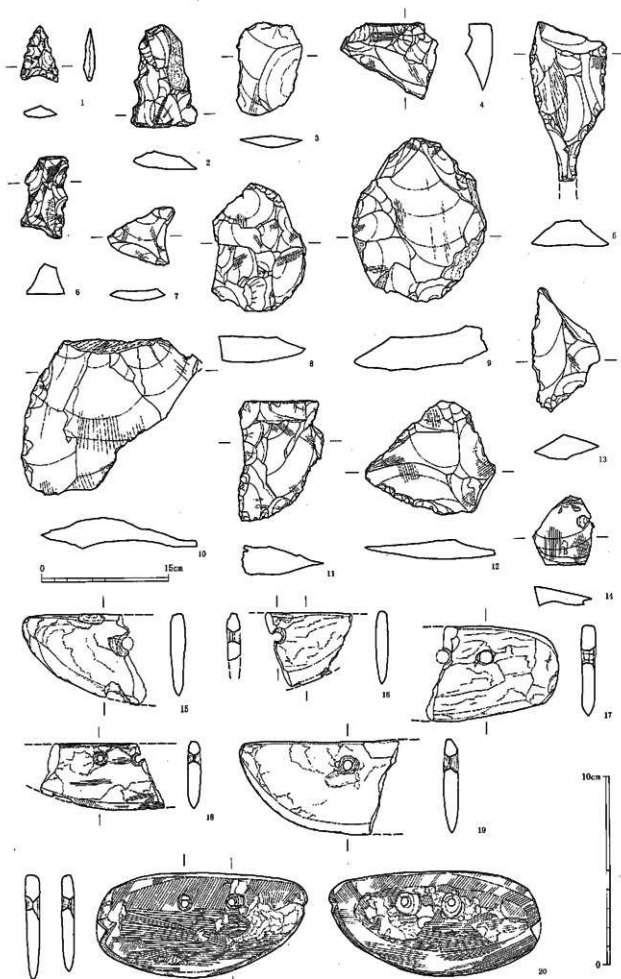
第91図 石器・石製品実測図(1) (1~14は2/3、15~20は1/2)
