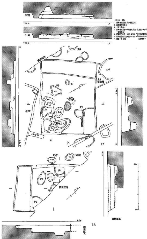
第35図 17・18号竪穴住居跡実測図 (1/60)
