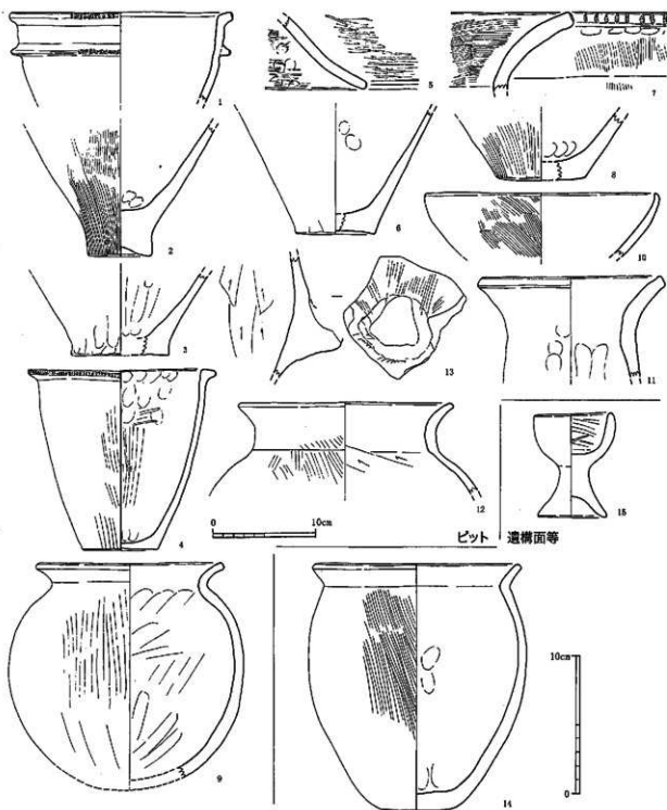
第72図 7区第1面ビット、遺構面等出土土器実測図（1～5は1/4、他は1/3） はナデ調整を行う。外面には黒斑があり、色は灰黄色。
