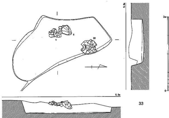
第 86 図 32・33 号土坑実測図 (1/40・1/30)
