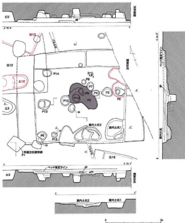
第33図 15号竪穴住居跡実測図 (1/60)
