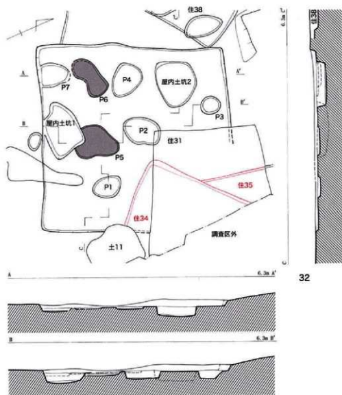
第60図 31・32号竪穴住居跡実測図 (1/60)
