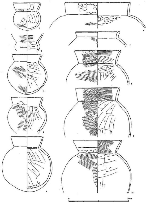
第 55 图 29 号竖穴住居跡出土土器実測図 (1) (1/3)
