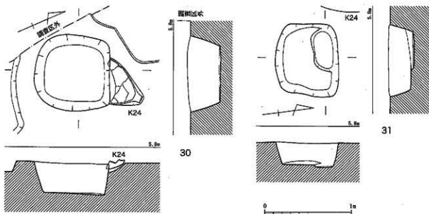
第 83 図 30・31 号土坑実測図 (1/30)
