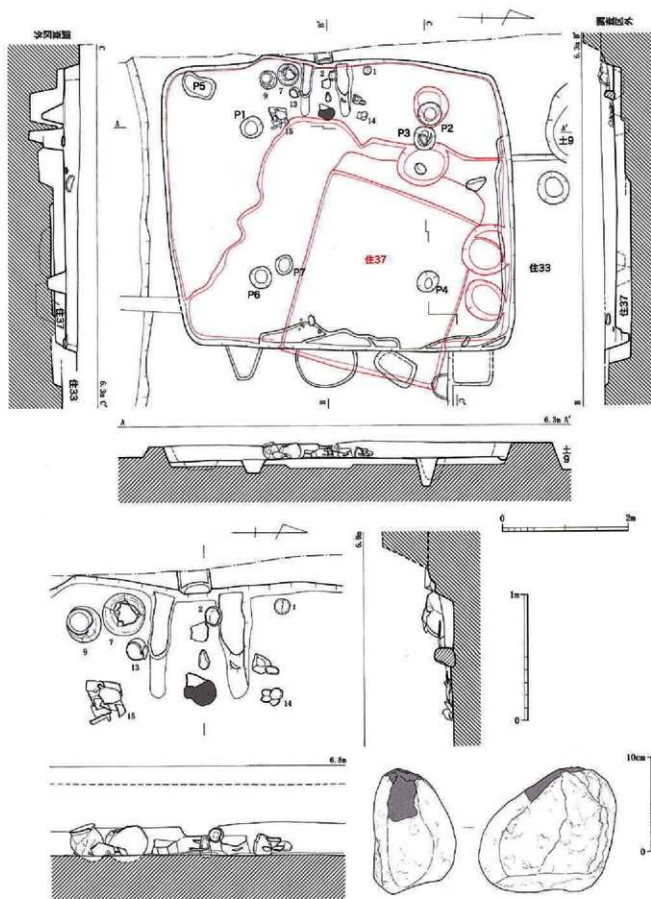
第49図 26号竪穴住居跡・カマド・カマド支脚実測図 (1/60・1/30・1/4)
