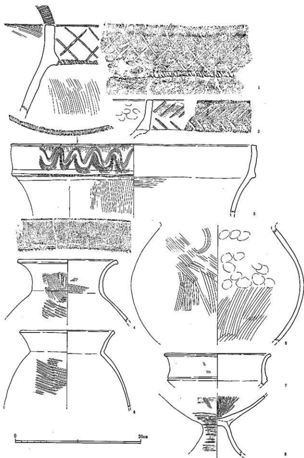
第 45 图 23 号竖穴住居跡出土土器実測図 (1) (1/3)
