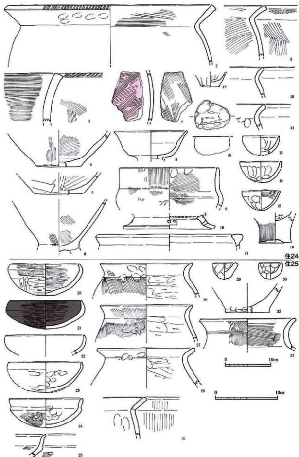
第47図 24・25号竪穴住居跡出土土器実測図 (17・18・33は1/4、他は1/3)
