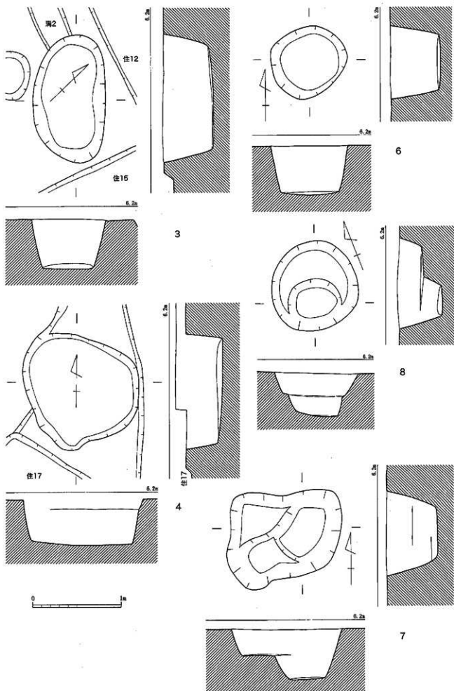
第 67 图 3·4·6~8号土坑实测图 (1/30)
