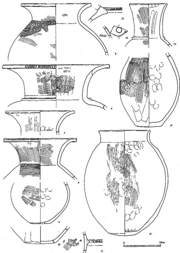
第29图 13号竖穴住居跡出土土器実測図(2)(1/3)
