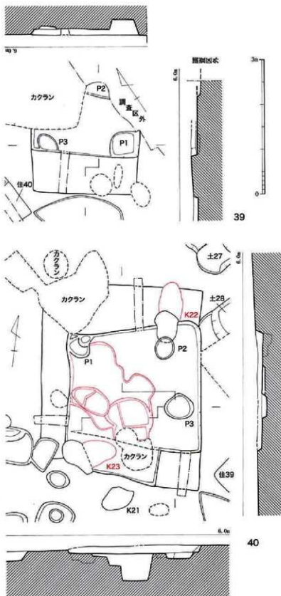
第73図 39・40号竪穴住居跡実測図 (1/60)
