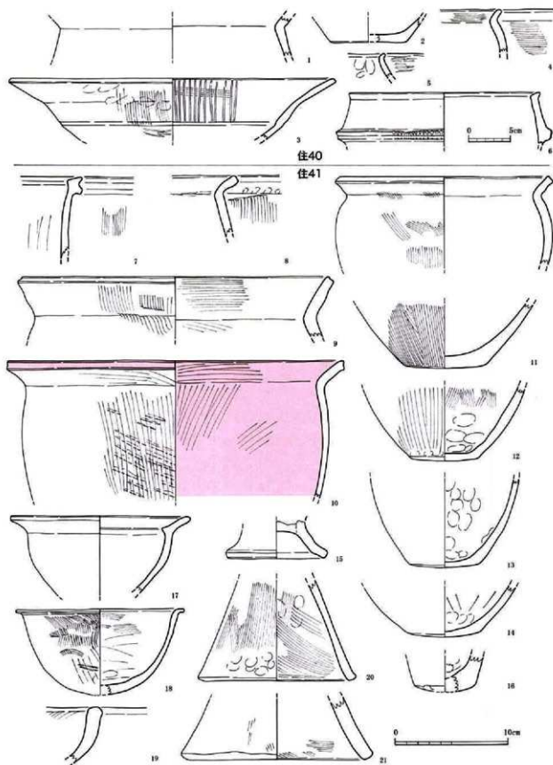
第75図 40・41号竪穴住居跡出土土器実測図（5・6は1/4、他は1/3）
