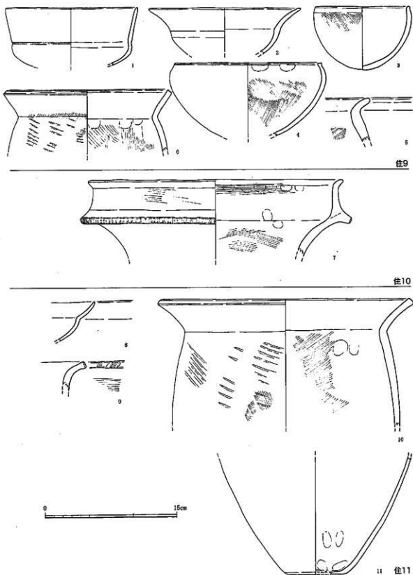
第 21 图 9 ~ 11 号竖穴住居跡出土土器実測図 (1/3)
