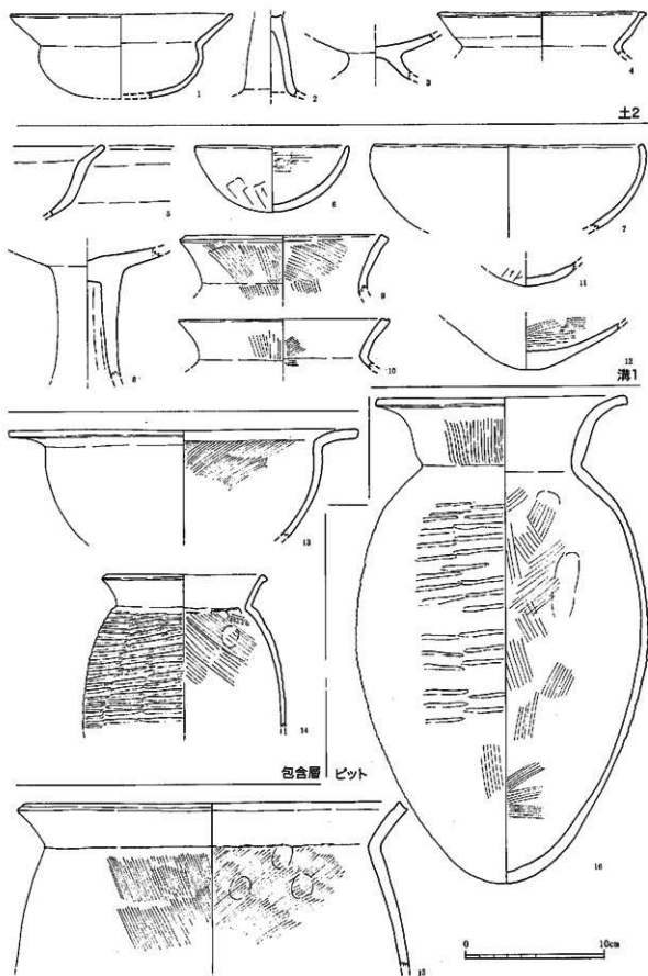
第23図 2号土坑、1号溝、ビット、包含層出土土器実測図 (1/3)
