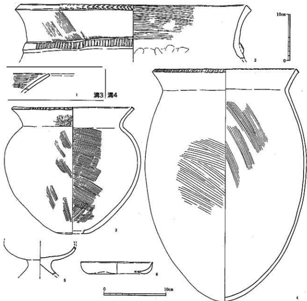
第71図 3・4号溝出土土器実測図(2は1/4、他は1/3)
