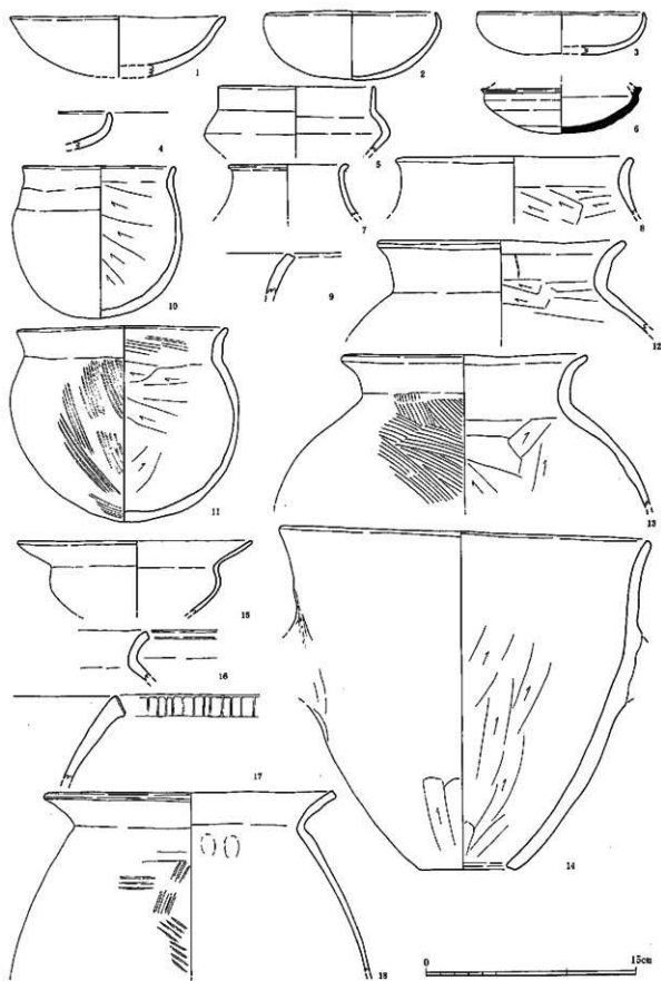
第13图 1号竖穴住居跡出土土器実測図 (1/3)
