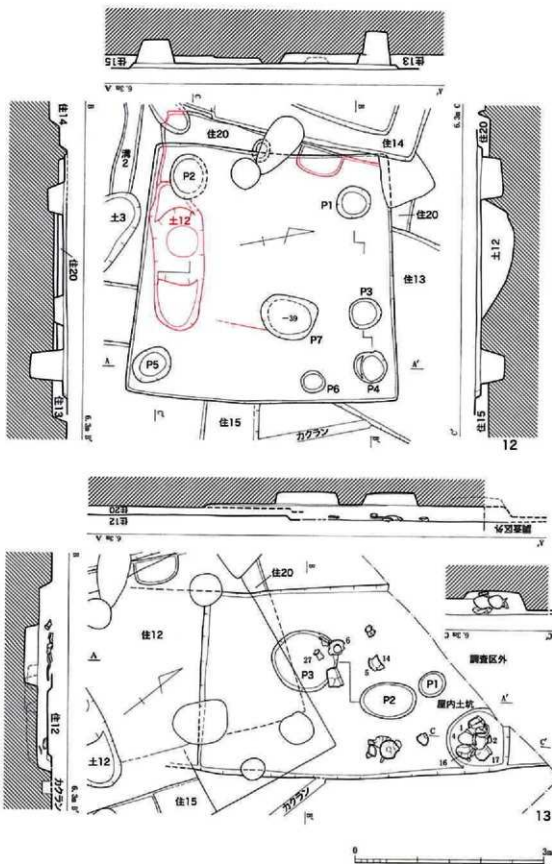
第26図 12・13号竪穴住居跡実測図 (1/60)
