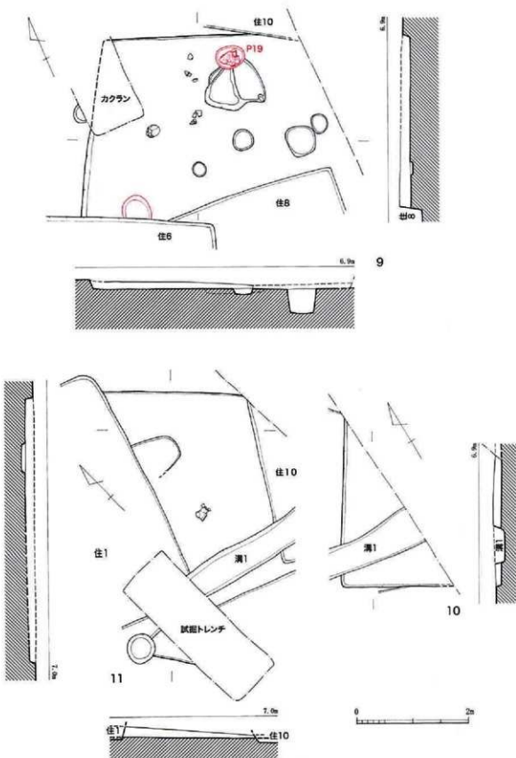
第20図 9～11号竪穴住居跡実測図 (1/60)
