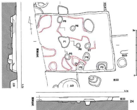
第44図 23・24号竪穴住居跡実測図 (1/60)
