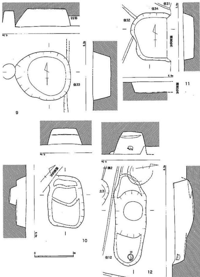
第69图 9~12号土坑实测图 (1/30)
