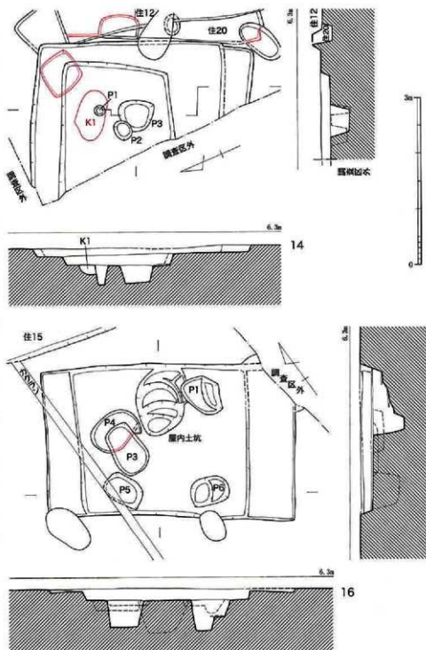
第32図 14・16号竪穴住居跡実測図 (1/60)
