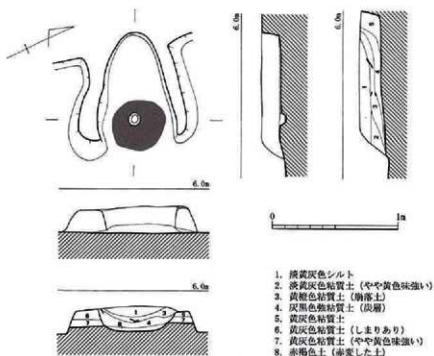
第12図 1号竪穴住居跡実測図 (1/60、カマドは1/30)
