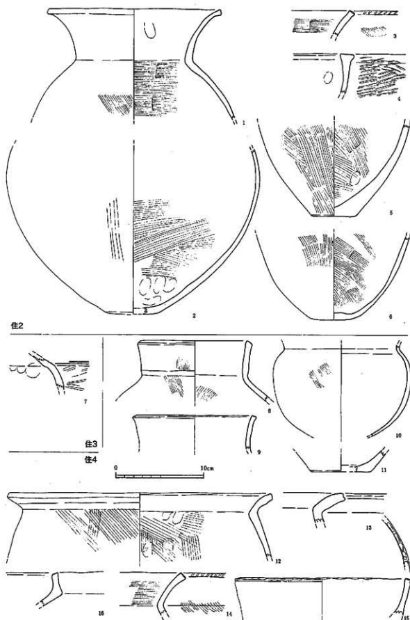
第 15 图 2～4 号竖穴住居跡出土土器実測図 (1/3)
