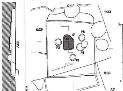
第63図 36・37号竪穴住居跡実測図(1/60)
