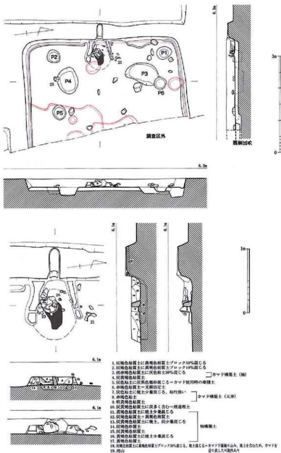
第52図 27号竪穴住居跡・カマド実測図（1/60・1/30）
