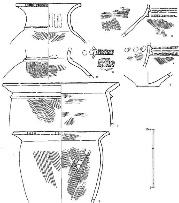
第54図 28号竪穴住居跡出土土器実測図 (1/3)
