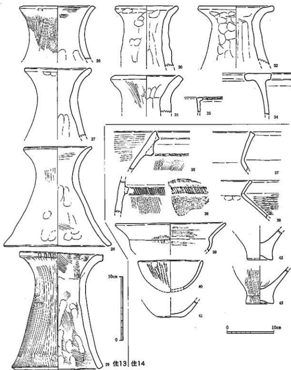
第31図 13(4)・14号堅穴住居跡出土土器実測図 (33・34・42・43は1/4、他は1/3)
