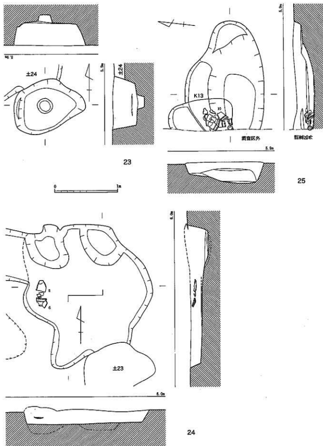
第 81 図 23 ～ 25 号土坑実測図 (1/30)
