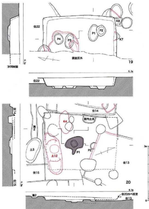
第38図 19・20号竪穴住居跡実測図 (1/60)
