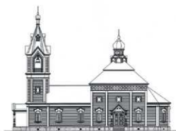
図13 京都聖堂南側立面図（現状）
