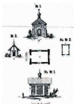
図1 「教会外観及び正面の設計図」 No.1～2
