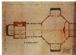
図10 仙台聖堂平面図（原設計図）
