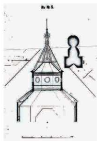
図12 同No.5屋根詳細図
