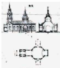
図11 「教会外観及び正面の設計図」No.5
