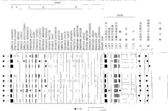
第3図 珪藻化石分布図
