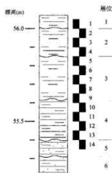
第2図 峰高前遺跡低地セクションにおける柱状図
