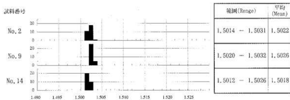
第5図 峰前遺跡における火山灰ガラスの屈折率
