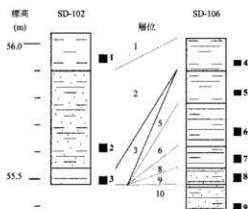
第2図 峰前遺跡 SD-102・106 の柱状図
