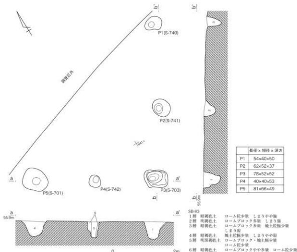
第271図 SB-83 掘立柱建物跡
