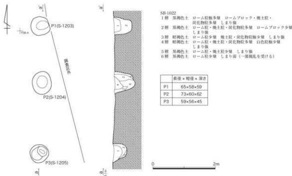
第281図 SB-1022 掘立柱建物跡
