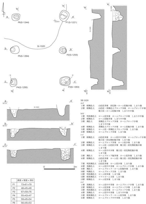
第284図 SB-1028 掘立柱建物跡
