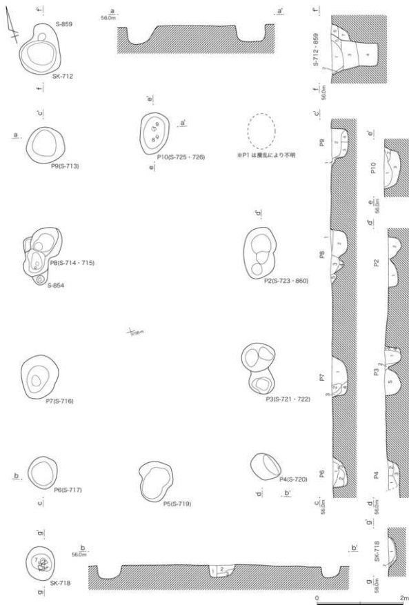
第 276 圖 SB-98 掘立柱建物跡
