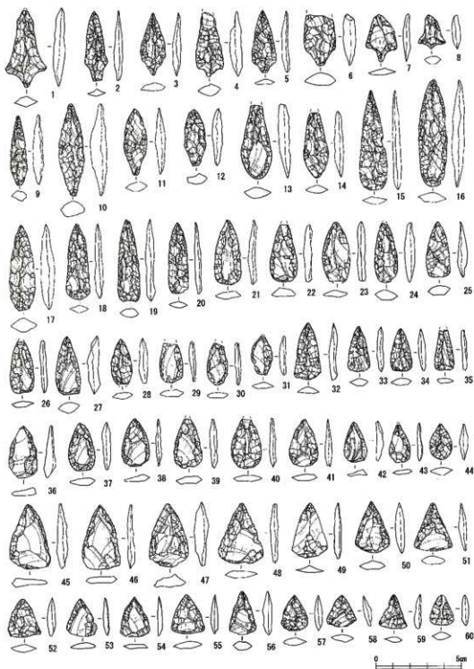
第120圖 石器実測圖2(縮尺1/2)
