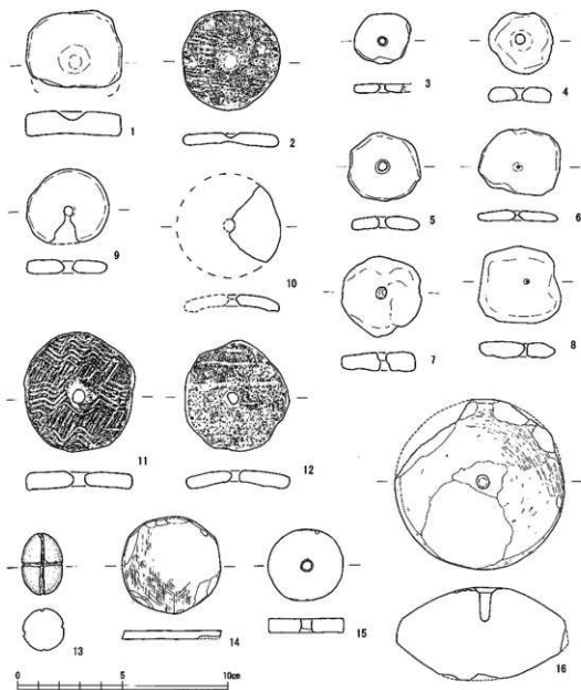
第132圖 土製品・石製品実測図(縮尺1/2)
