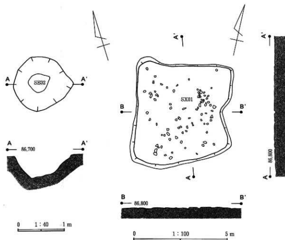
図8 1区SXD01実測図
