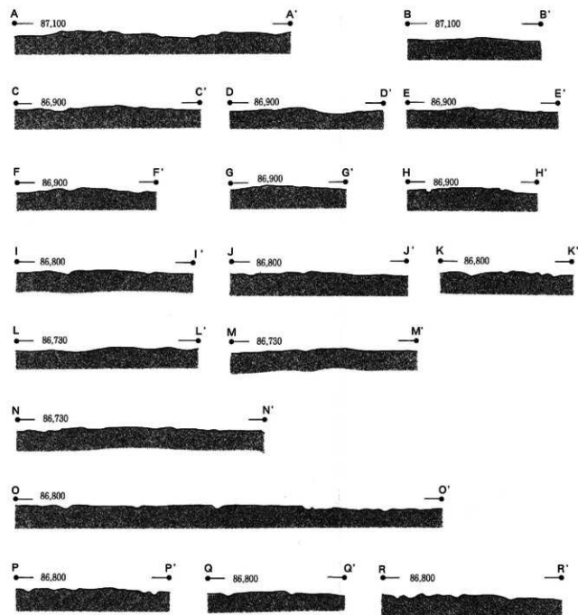
図9 1・3～5区 (A-B直下) 実測図
