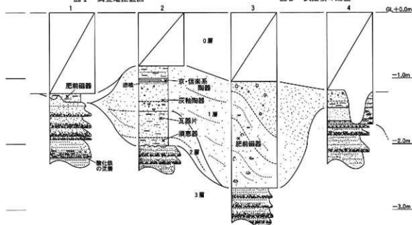
図3 各試掘坑の地質柱状図
