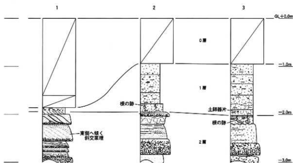
図3 各試掘壕の地質柱状図
