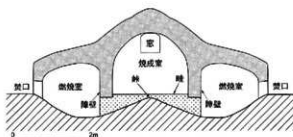
図9 連磨窯の構造(連磨窯の基本形[藤原学2001]に加筆)
