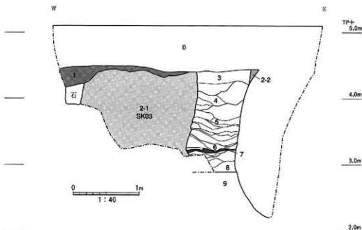
図3 北壁断面図
