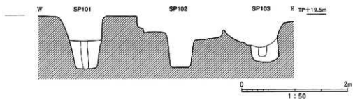
図6 SA101断面図
