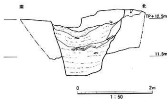
図4 SE101断面図
