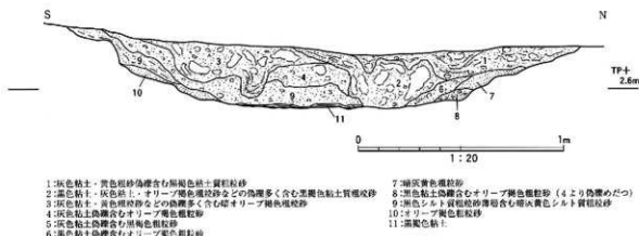
図3 SD01断面図
