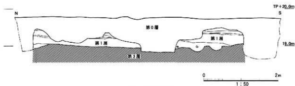
図3 東壁断面図
