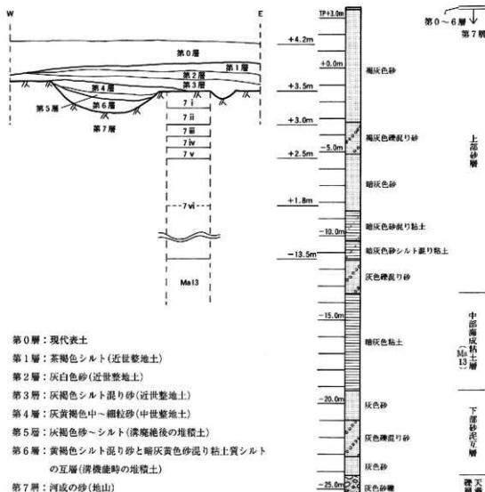
図3 層序模式図
