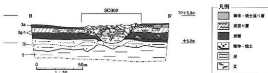
図20 暗渠SD302断面図
