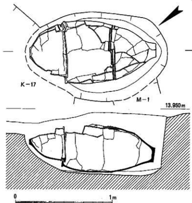
Fig.24 19号壺棺墓実測図 (1/20)
