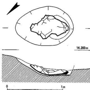
Fig.9 3号雙棺墓実測図 (1/20)
