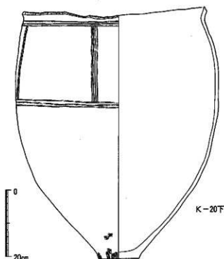
Fig.49 20号壺棺墓上・下甕実測図 (1/8)
