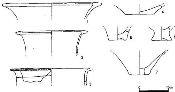
Fig.54 1号土墳出土土器実測図 (1/4)
