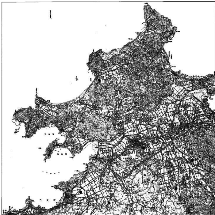
第1図 分析に用いた遺跡 (1/100,000)
