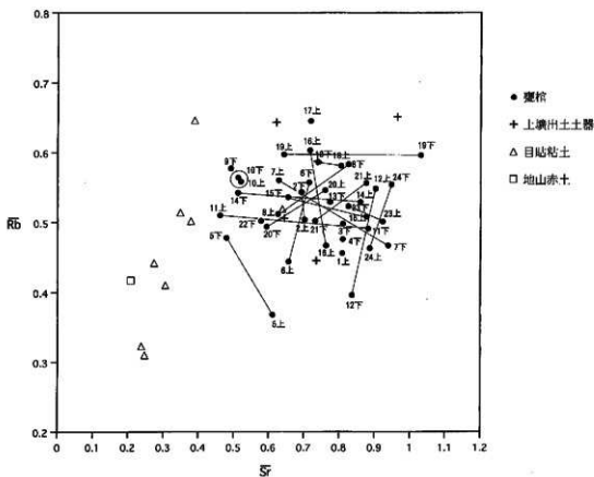
第3圖 久米遺跡試料のK-Ca(上)、Rb-Sr(下) 分布図
