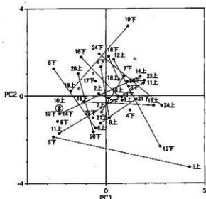
第4図 久米遺跡墓棺・土壌出土土器の主成分分析結果
