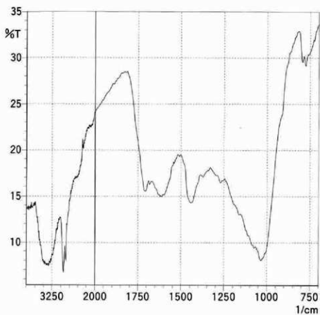
図244 試料の赤外吸収スペクトル
