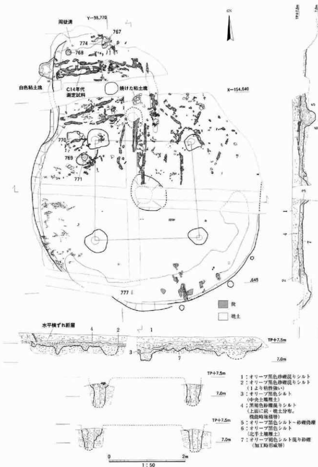
図139 SB015平・断面図
