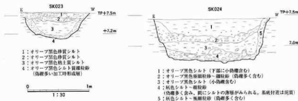
図22 SK023・024断面図
