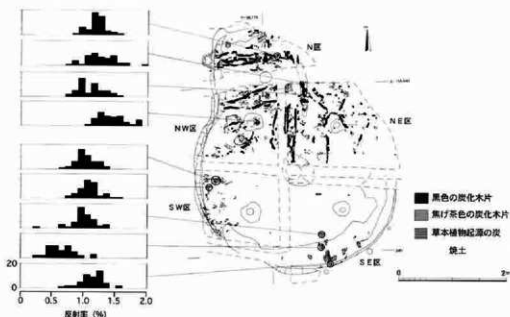
図238 焼失住居SB015における炭の分布と反射率ヒストグラム
