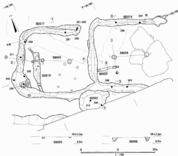
図78 SB005・006、SE002平面図
