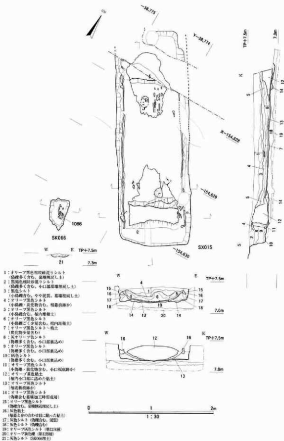
図189 SX015・SK066平・断面図
