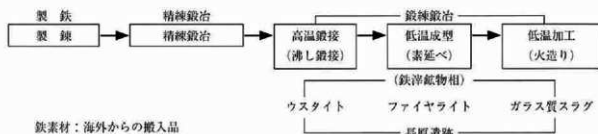
図245 鉄器製作工程の流れ一覧(鉱石)
