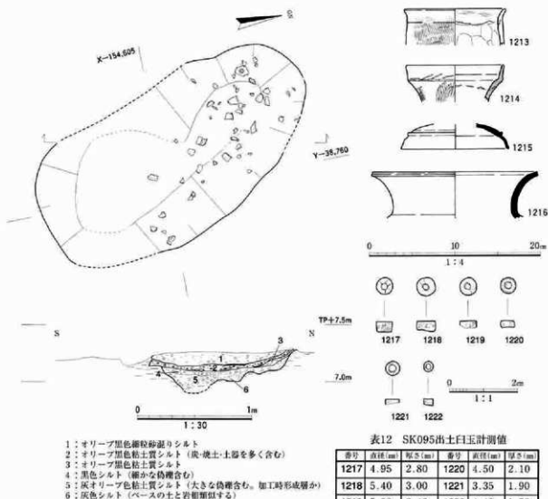
図218 SK095平・断面図および出土遺物
