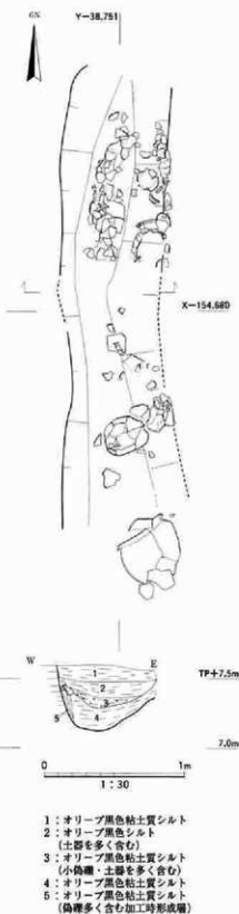
図31 SD006平・断面図
