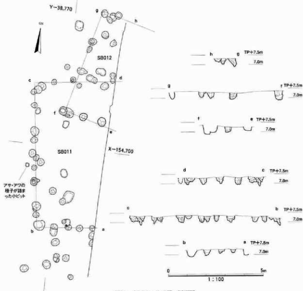
図85 SB011・012平・断面図
