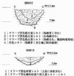
図43 SD010～013断面図
