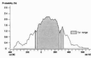
図239 MethodBによる校正年代の確率分布
