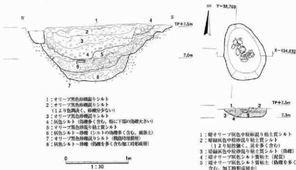
図148 SK058断面図およびSK061平・断面図
