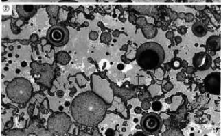
写真31 ガラス滓小片の顕微鏡組織
