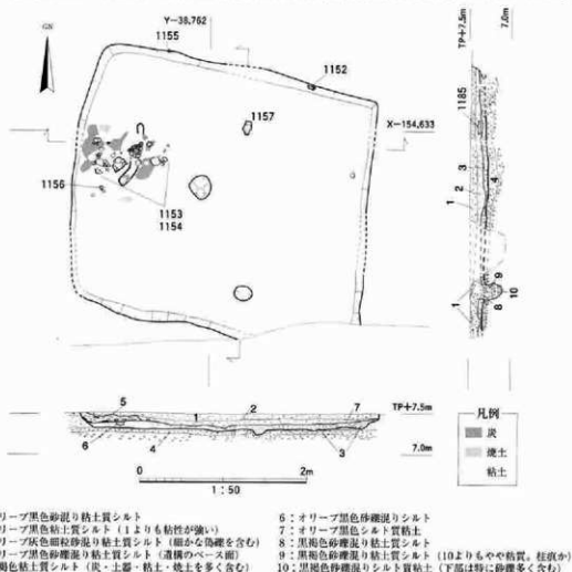
図203 SB020平・断面図
