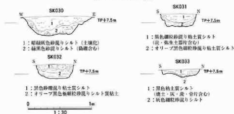
図28 SK030～033断面図
