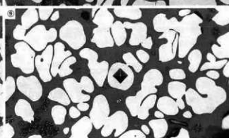
写真32 小型碗形鍛冶滓の顕微鏡組織
