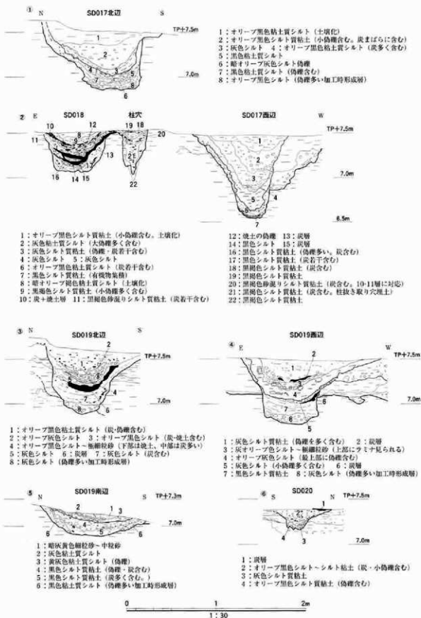
図79 SD017～020断面図
