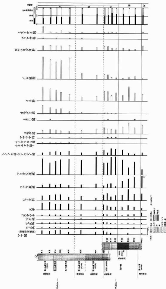
図248 NG02-8 次調査地D地点花部ダイアグラム
