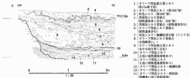
図82 SE002断面図
