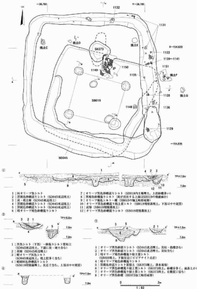
図200 SB019・SD045平・断面図
