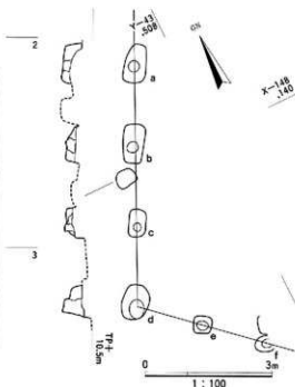
図17 東調査区SA54平面・断面図
