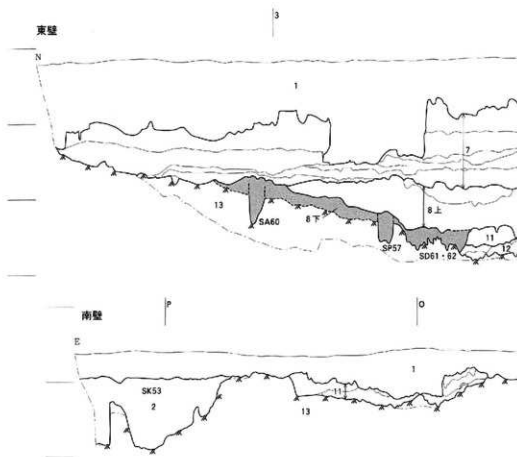
図6 東調査区東・南壁地層断面図(1)
