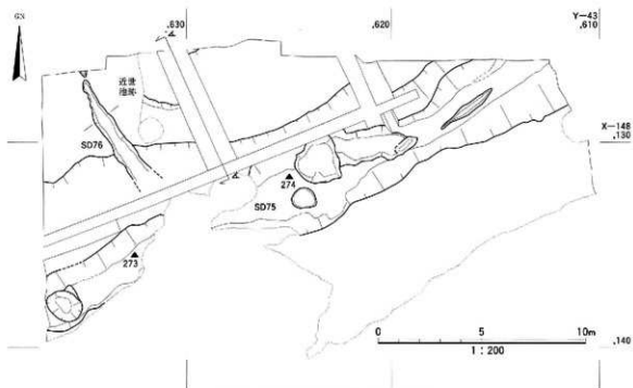
図29 西調査区飛鳥時代の遺構平面図
