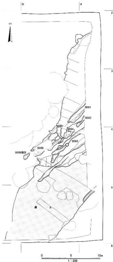
図12 東調査区谷平面図(古墳～飛鳥時代)
