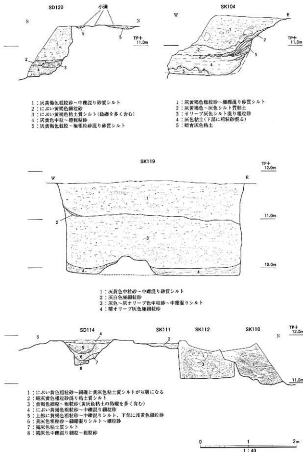
図49 西調全区江戸時代の遺構断面図
