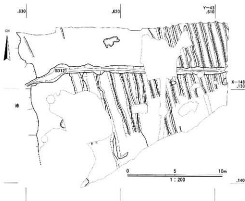
図50 西調査区江戸時代の遺構平面図(2)
