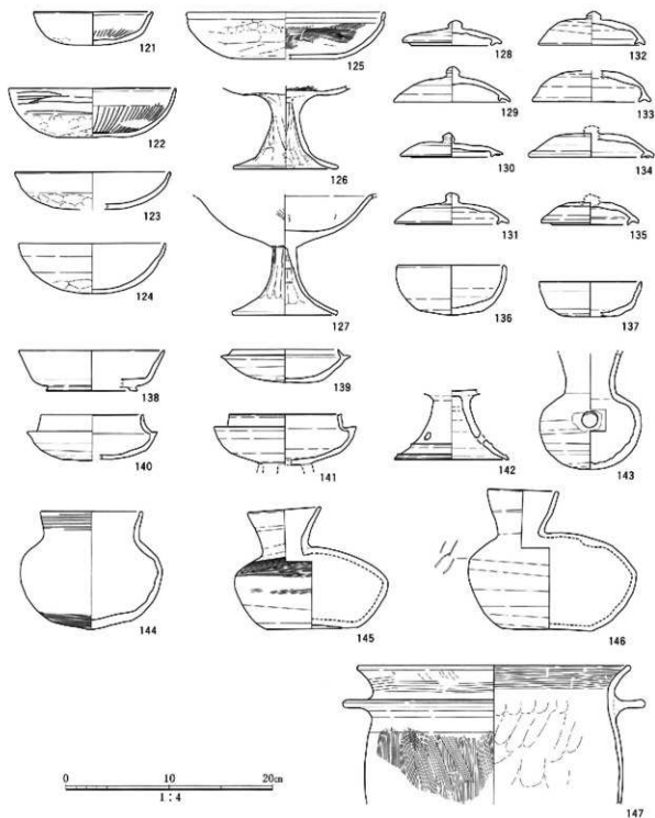
図30 西調査区SD75出土土器
