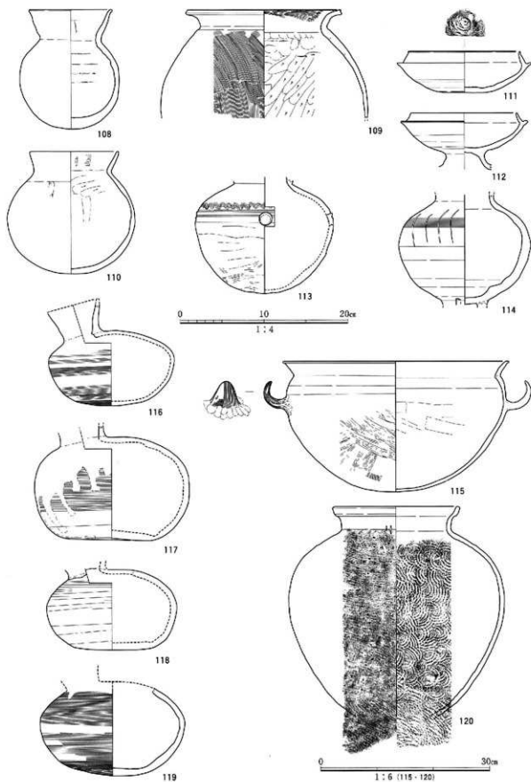
图28 西洞全區SD71·SX72·SD73·土器集中部出土土器
