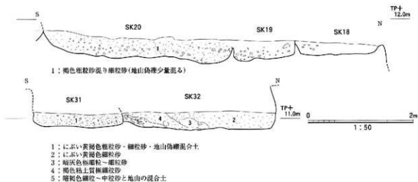
図21 東調査区近世の遺構断面図(2)
