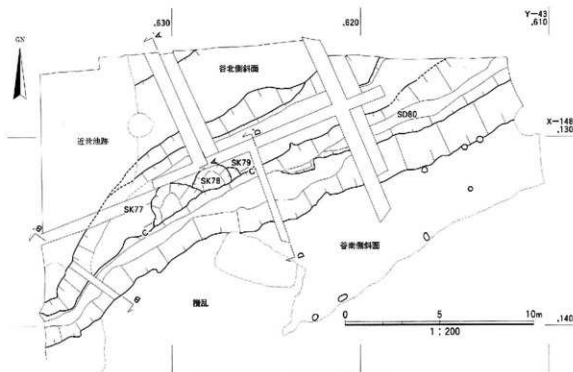
図32 西洞査区奈良時代の遺構平面図
