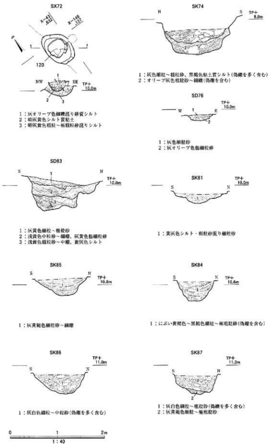
図27 西調査区古墳～平安時代の遺構
