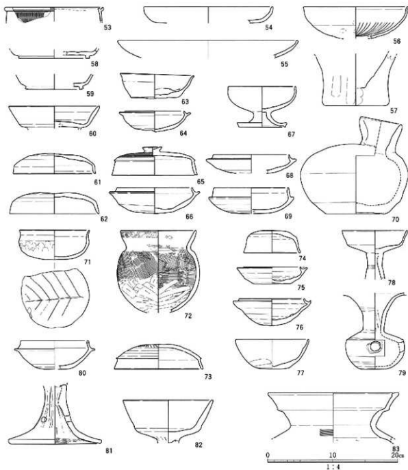
図23 東洞査区各地層出土の遺物実測図 第2層(53)、第7層(54~70)、第8層上・下部(71~79)、第11層(80~83)
