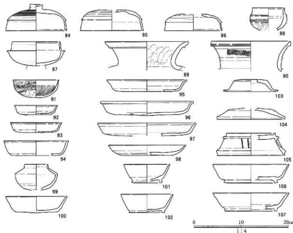
図24 東調査区近世遺構出土の古代以前の遺物実測図
