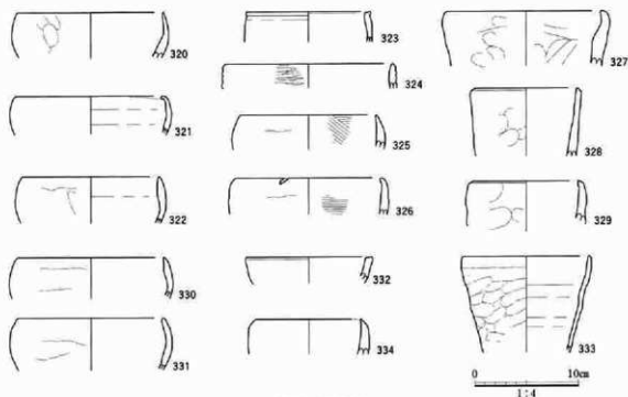
図83 製塩土器
