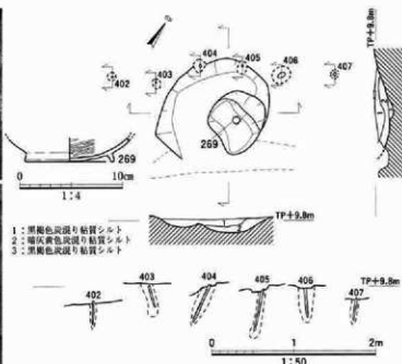
図66 SK401実測図
