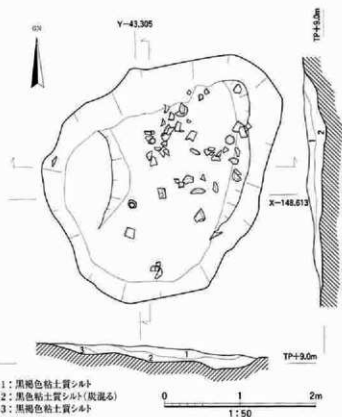
図49 SK504実測図
