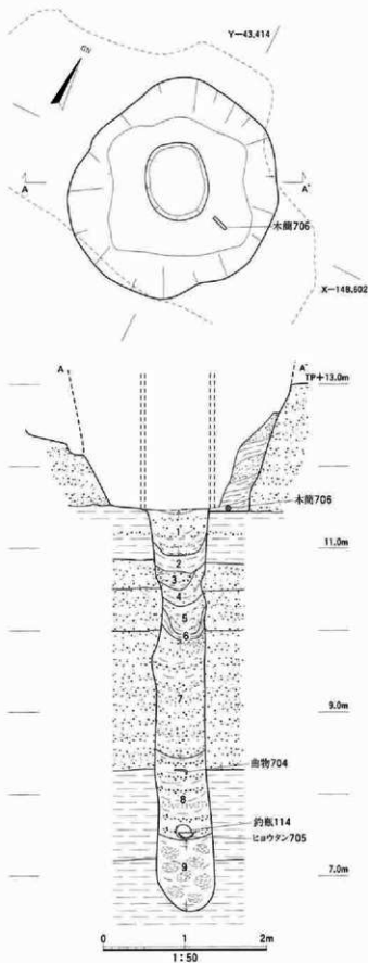
図26 SE606実測図
