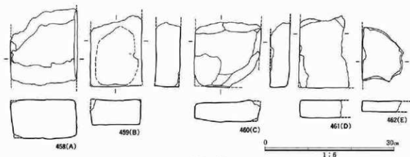
図81 塼
