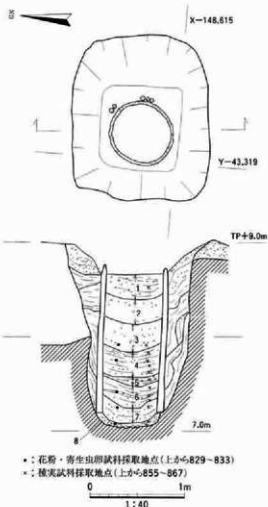
図51 SE505実測図
