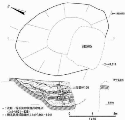
図24 SK605実測図
