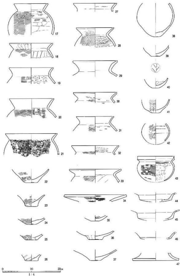
图12 SK66出土遗物实测图(2)
