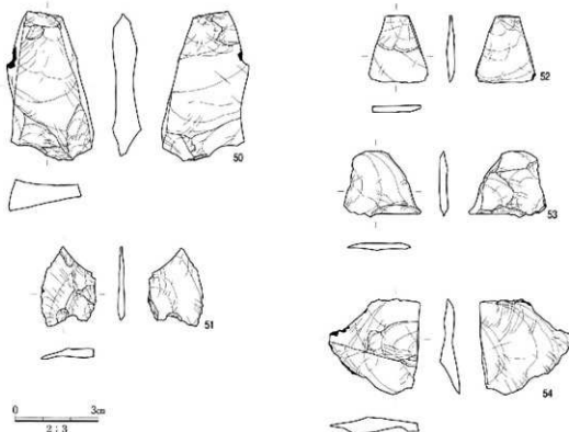
図15 SX59および周辺出土遺物実測図
