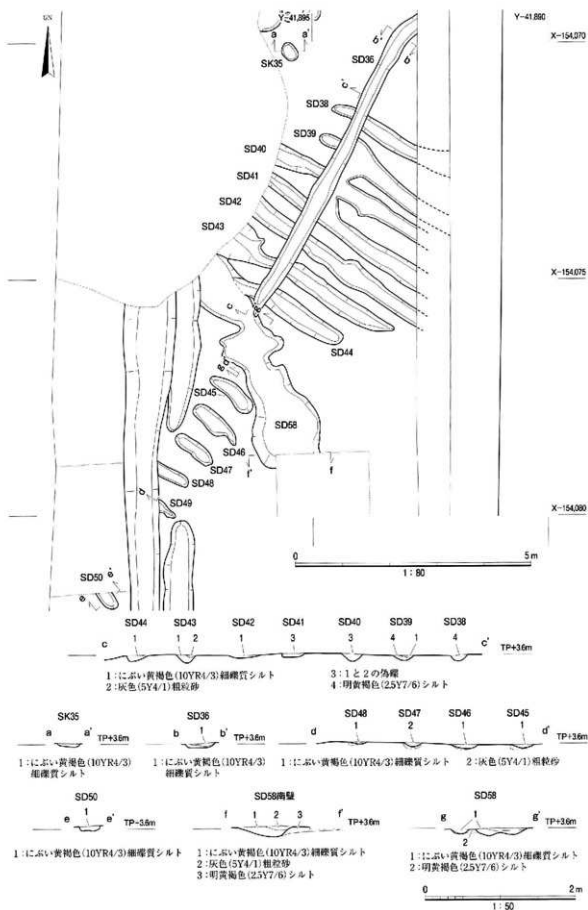
図27 SK35・SD58・扇溝群平面・断面図
