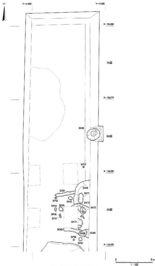
图8 第6层上面结构配置图(1)
