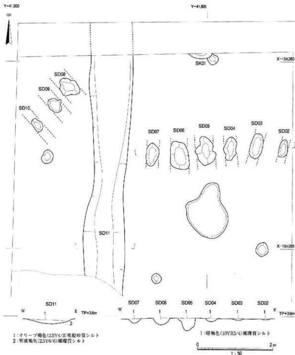
図26 SD11・鋤溝群平面・断面図
