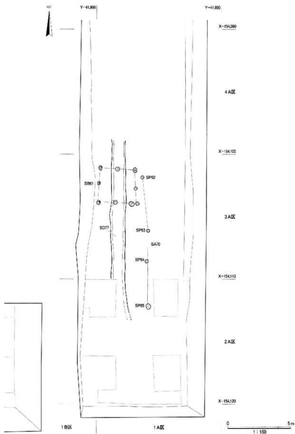
図24 第4層下面および第5層上面連携配置図(2)
