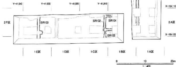
図29 第2層上面遺構配置図
