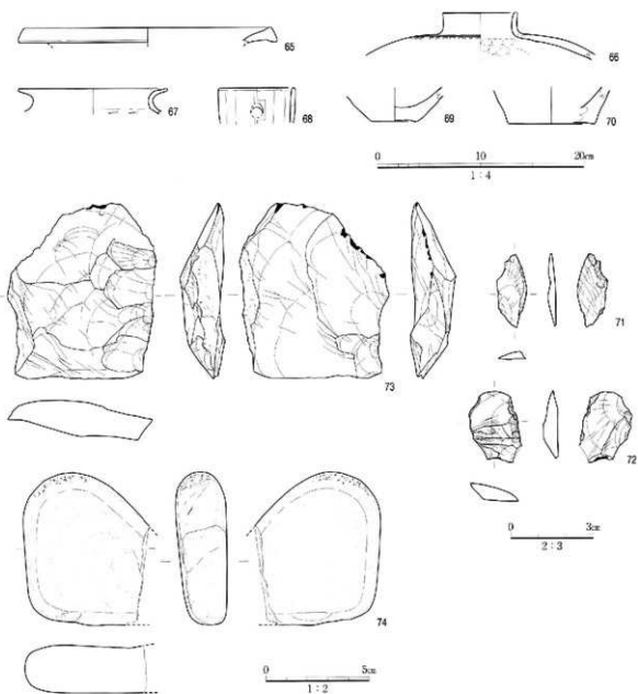
图22 SX75北周溝出土遺物実測図
