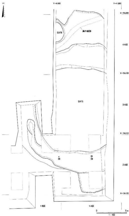
図9 第6祠上面遺構配置図(2)
