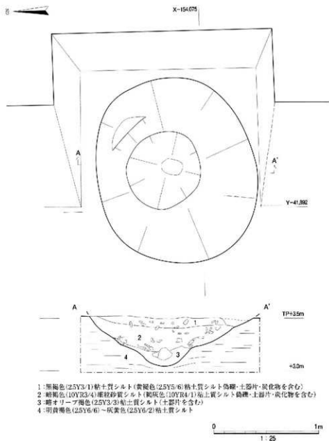
図10 SK66平面・断面図
