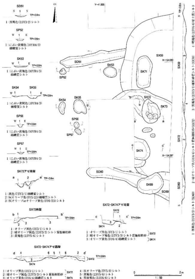
図14 第6層上面遺構平面・断面図
