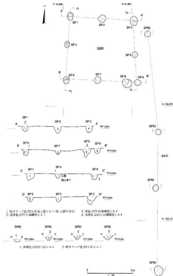
図25 SB61・SA70平面・断面図
