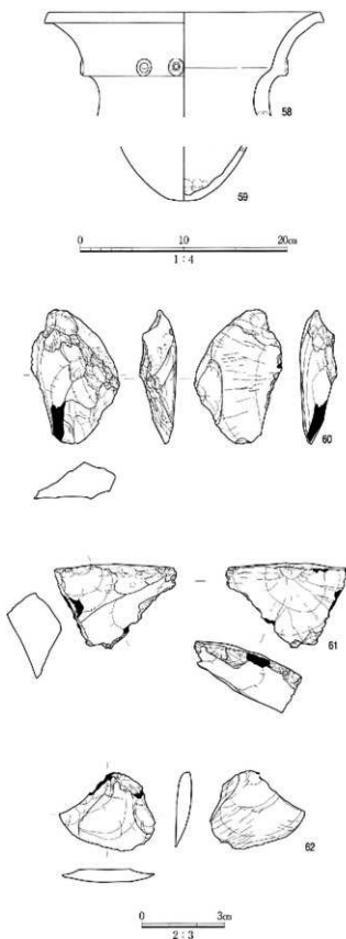
図20 SX75南周溝出土遺物実測図
