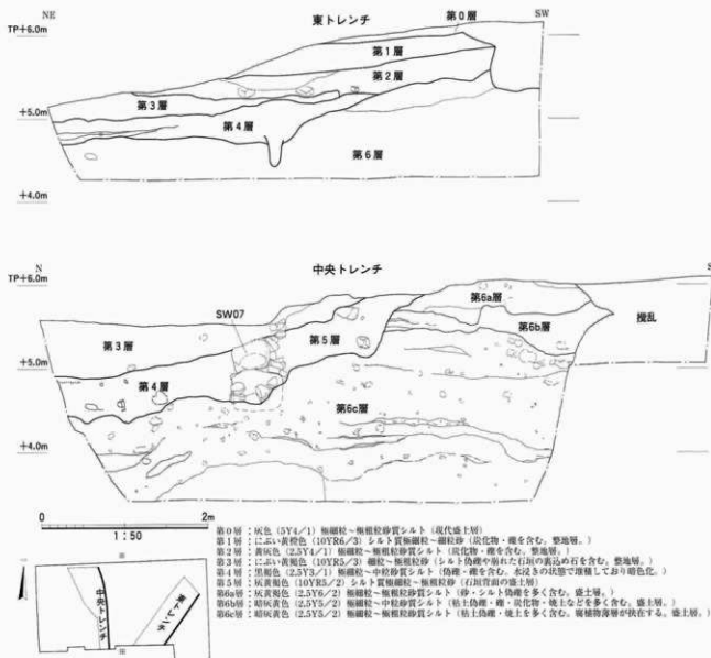
図4 東・中央トレンチ地層断面図
