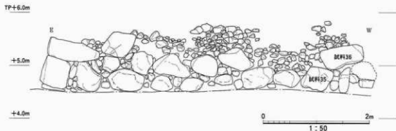
図6 SW07東半立面図
