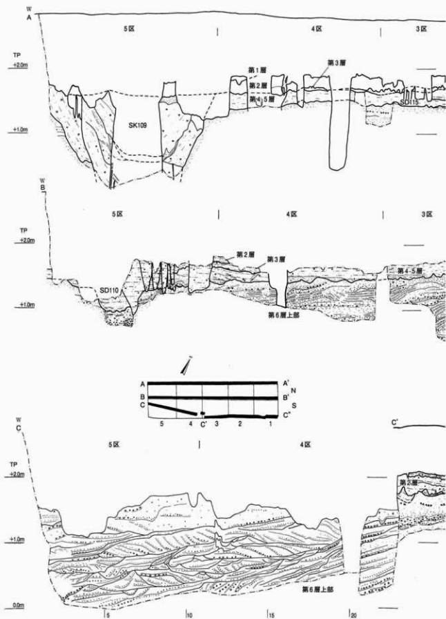
图8 A区东西地層断面图
