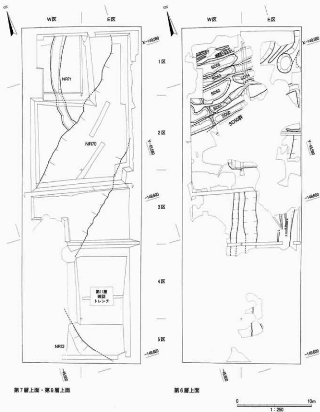
図15 B区遺構平面図(1)
