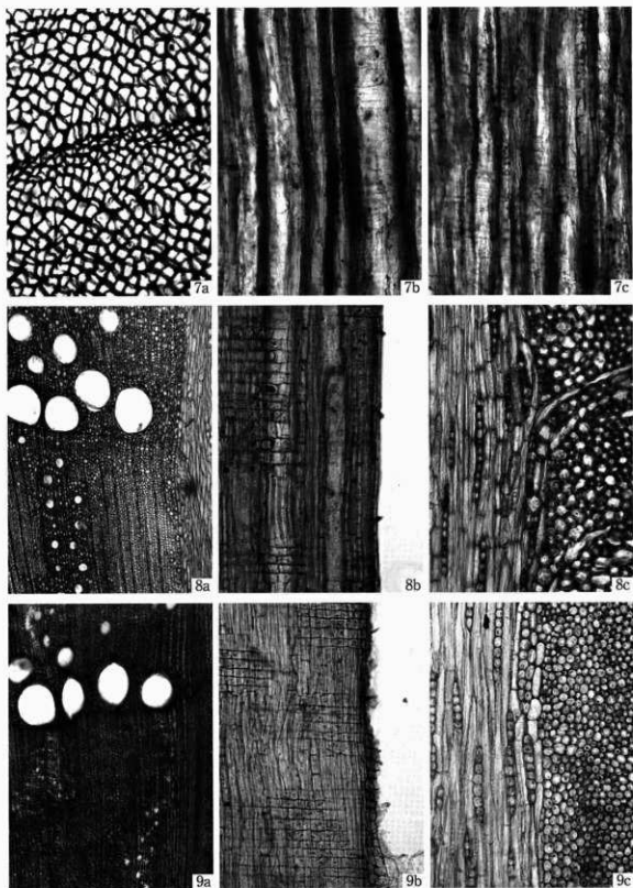
7. ヤナギ属<根材> (表6の試料43) 8. コナラ属コナラ亜属クヌギ節 (同25) 9. コナラ属コナラ亜属コナラ節 (同63) a: 木口, b: 柾目, c: 板目
