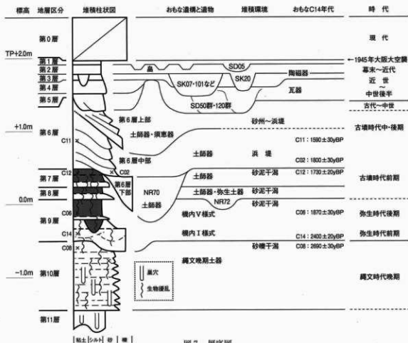
図7 層序図
