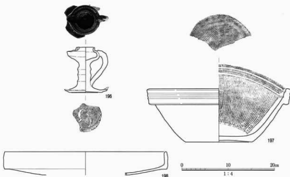
図30 SK14出土遺物実測図(2)
