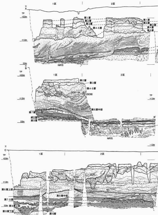
图10 B区南北地层断面图
