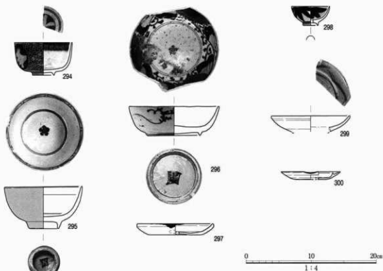
図35 SK32・35出土遺物実測図 SK32(294～297)、SK35(298～300)
