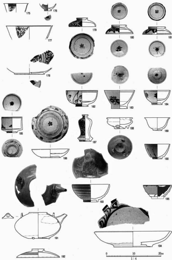
图29 SK14出土物实测图(1)
