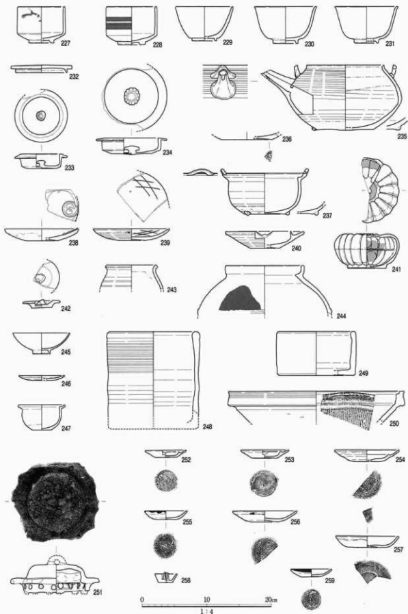
図32 SK19出土遺物実測図(2)
