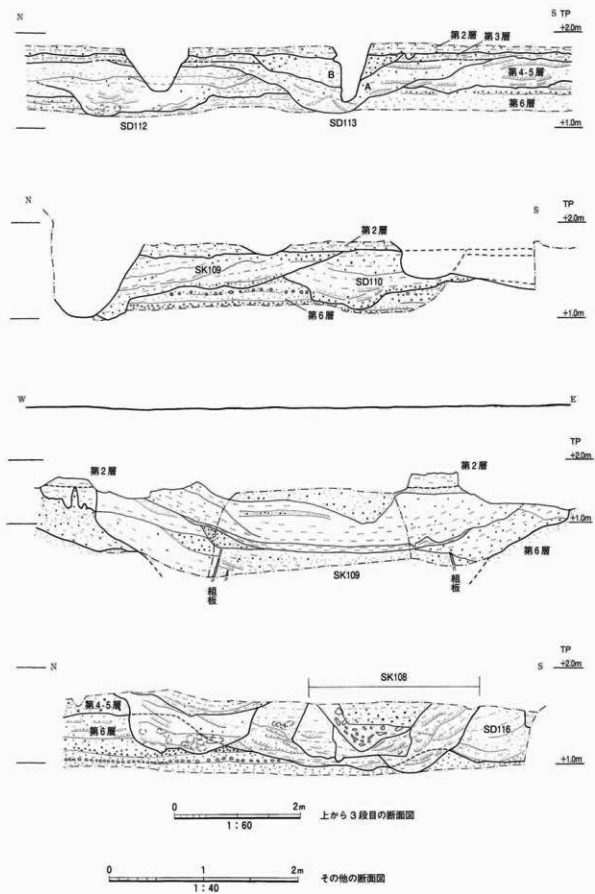
図19 A区遺構断面図
