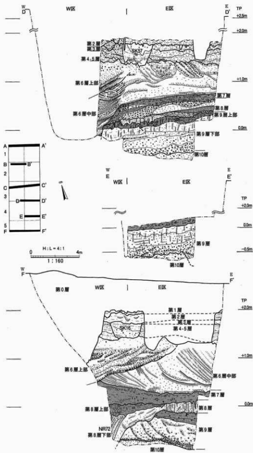
图12 B区东西地层断面图(2)
