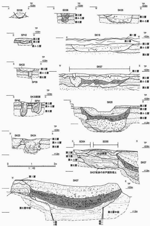
図28 B区遺構断面図(2)
