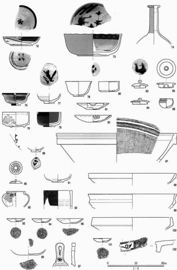
图24 SK105出土遗物实测图
