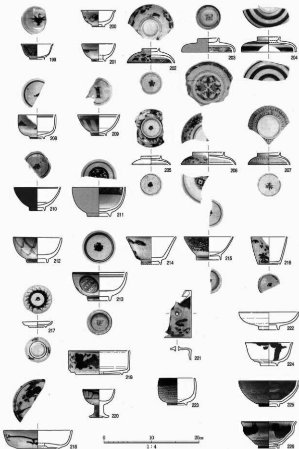
图31 SK19出土遗物实测图(1)
