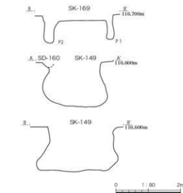
第48図 II区 区割14断面図
