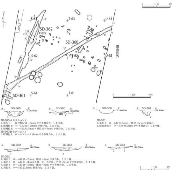
第84図 V区 区割10 (SD)
