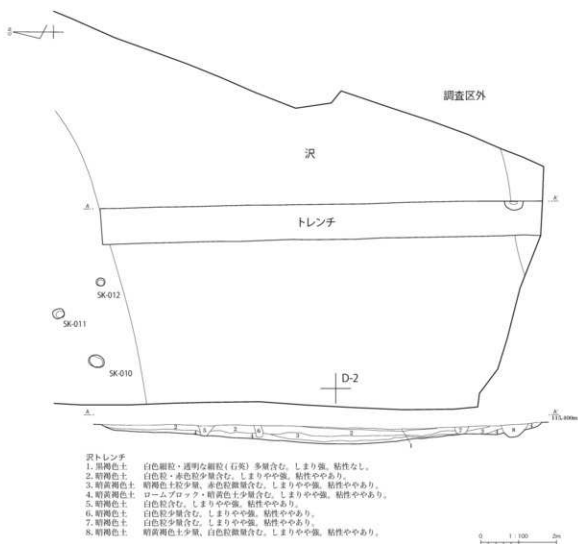
第97図 Ⅰ-5区 区割9
