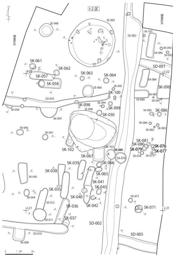
第19图 1-2・1-3区 区割8
