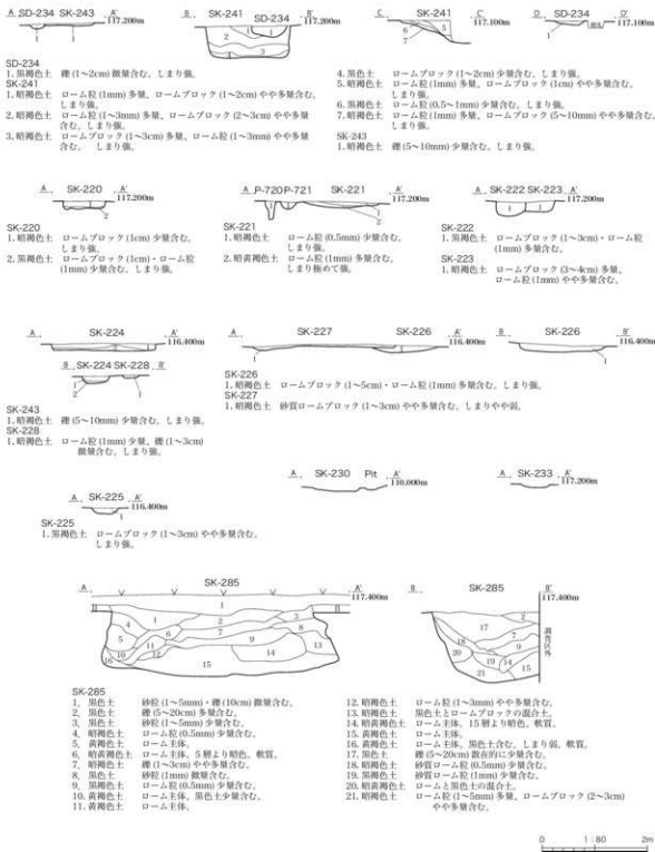
第35図 II区 区割6断面図
