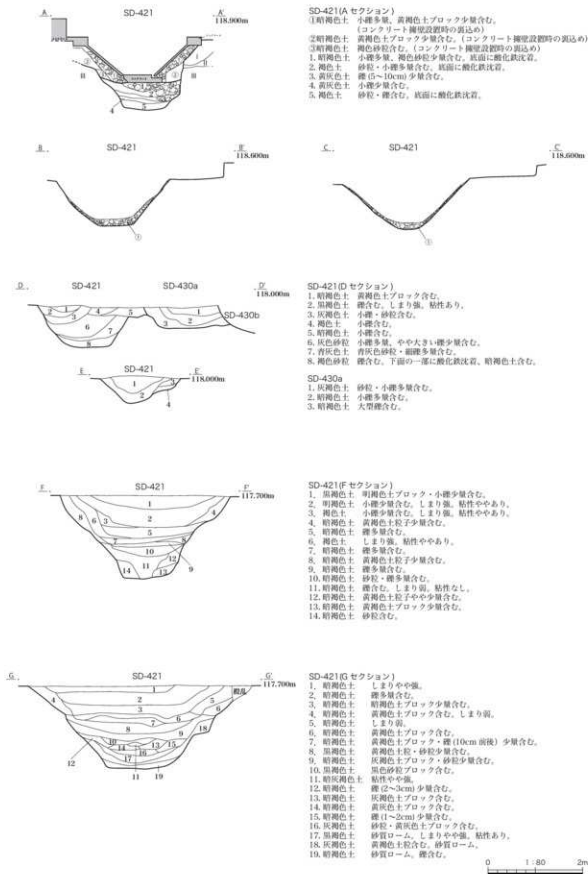
第60図 Ⅲ区 断面図(1)
