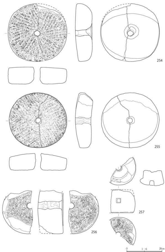
第124図 石臼実測図(1) 254～257
