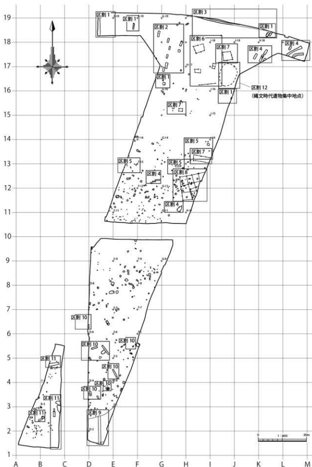
第88図 1-4・1-5・1-6区 区劃配置図
