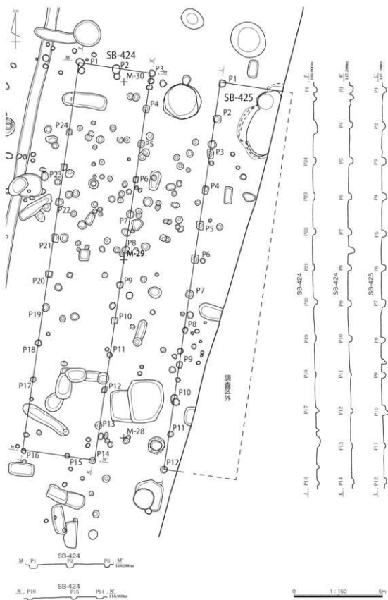
第57図 II区 区割20(SB-424・425)
