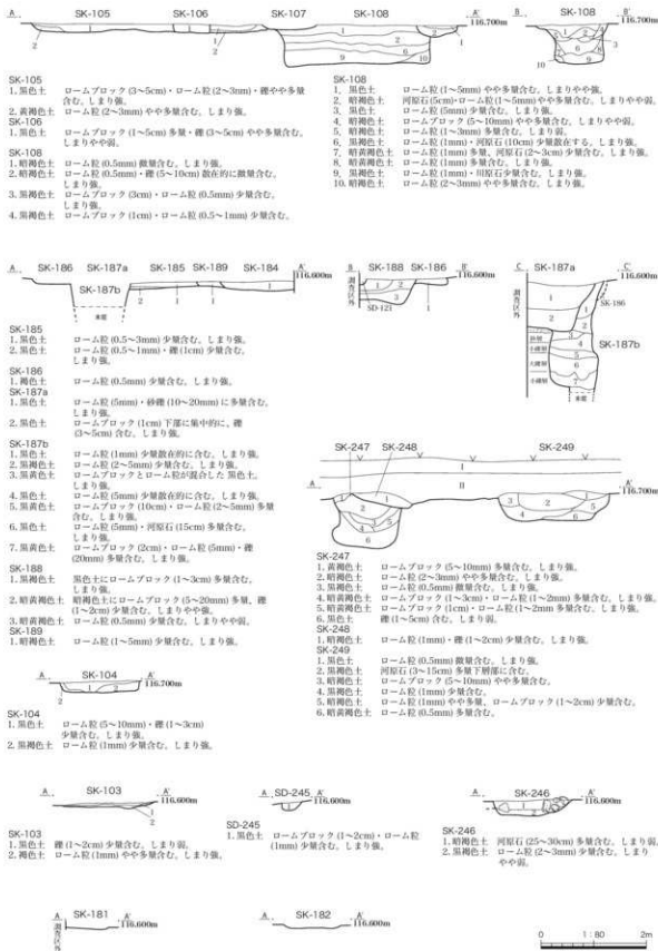
第52图 II区 区割16断面图
