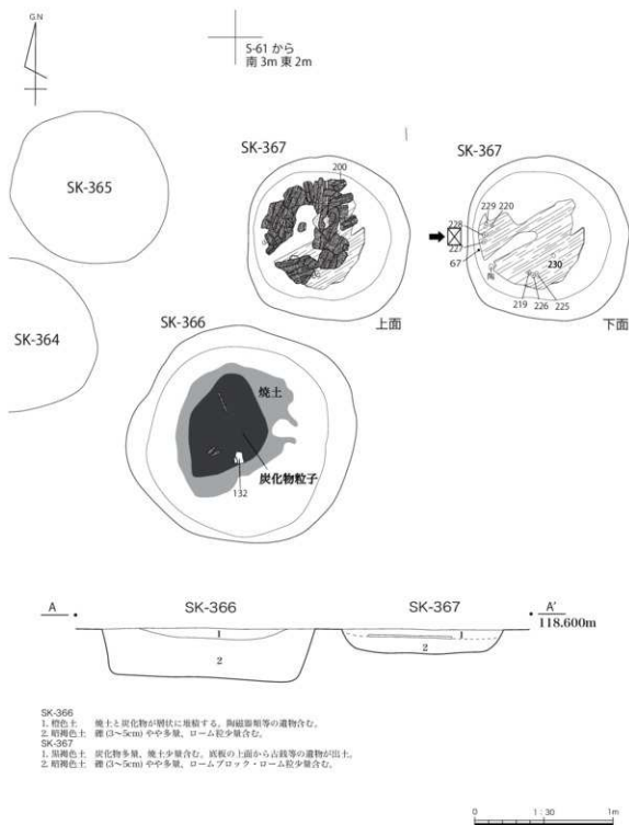
第 87 図 V 区 SK-366・367 (墓墳)
