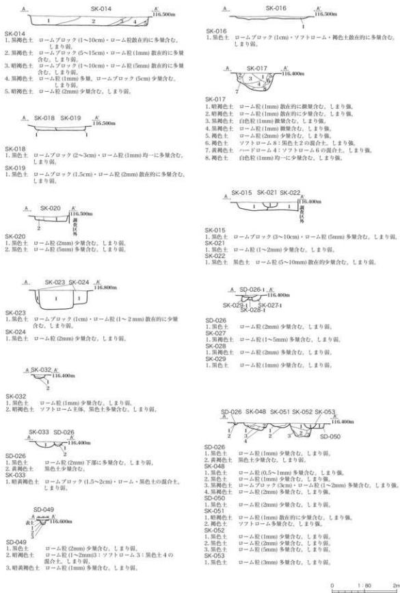
第23図 1・2・1・3区 区割10断面図
