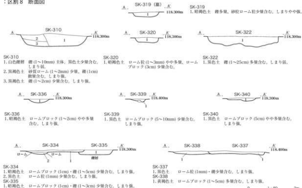
第82図 V区 区別7・8断面図
