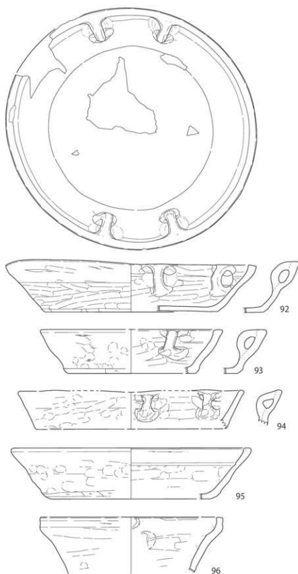
第108図 内耳土器実測図(5) 92～96
