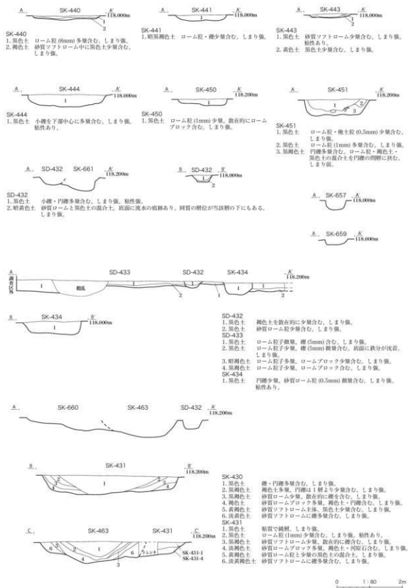
第 67 图 IV 区 区割 4 断面图
