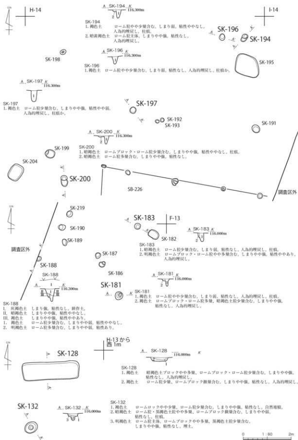
第93図 I-4区 区割5
