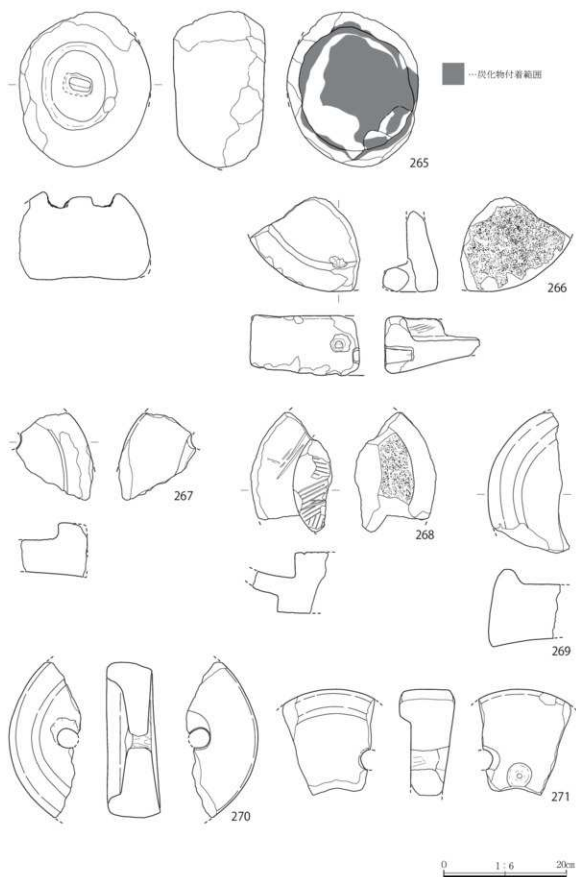
第127図 石臼・石製灯明具実測図 265～271
