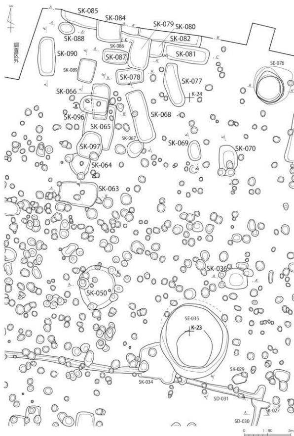
第12図 I - 1区 区割2
