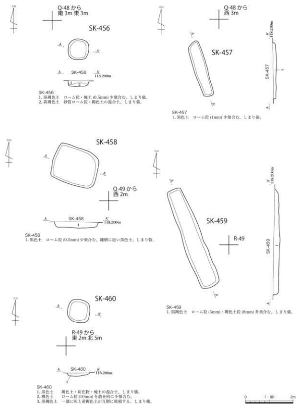
第 63 図 IV 区 区割 1
