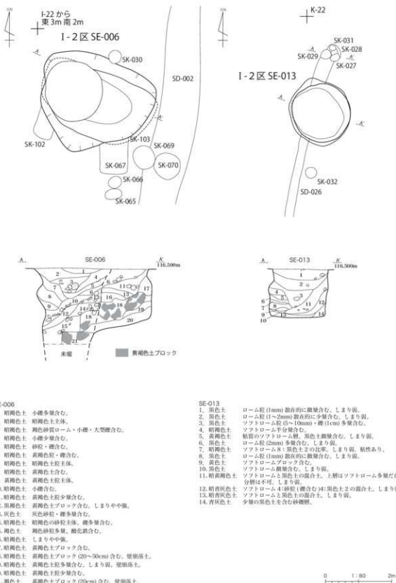
第25図 I-2・I-3区 区割12 (井戸)
