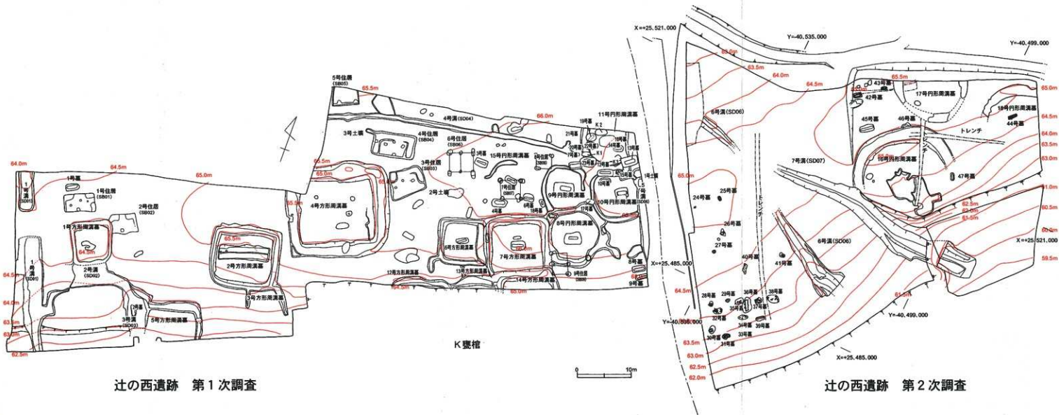
第3図 辻の西遺跡第1次調査・第2次調査遺構配置図 [1/500]
