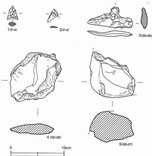
第12図 溝 (S D-06-07) 柱穴出土石製品 [1/2]
