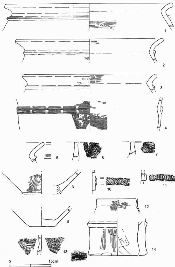
第11圖 溝(SD-06)出土土器 [1/4]
