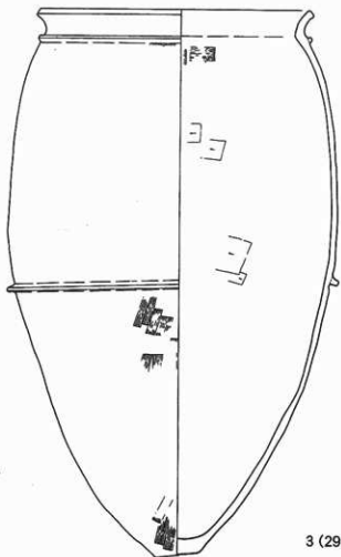
第6図 辻の西遺跡 第2次調査 27・28・29号壺棺 [1/8]
