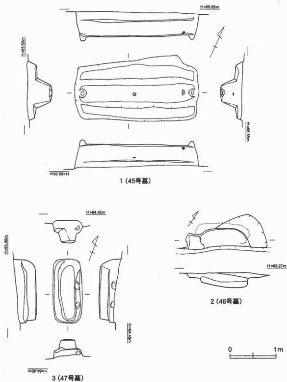
第15図 辻の西遺跡第2次調査 45号木棺墓 45号・46号・47号土槨墓 [1/40]
