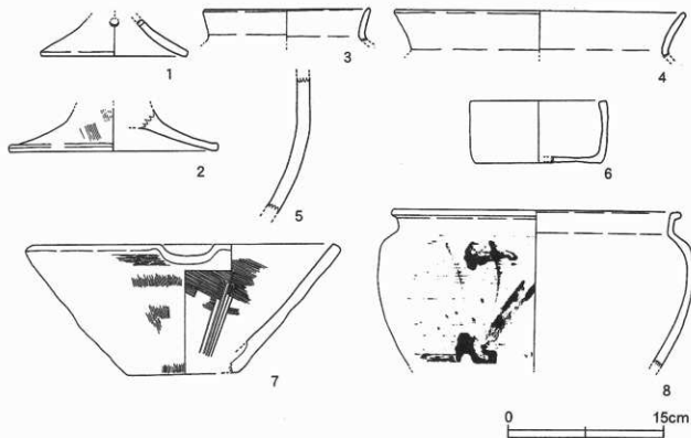
第17図 溝(S D 07) 出土土器 [1/4]
