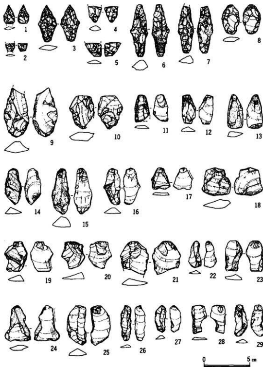
第10圖 石器実測図(1)
