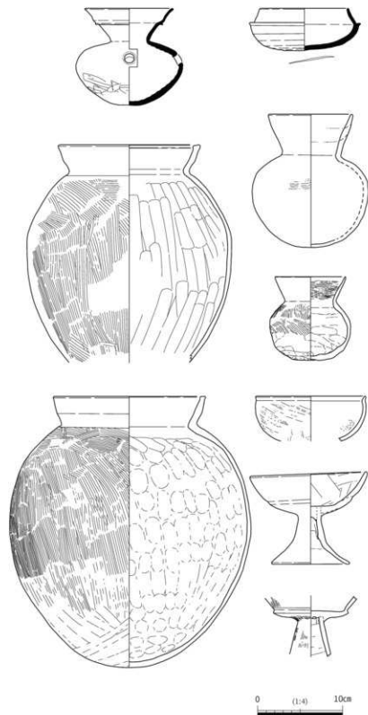
図13 III・IV区 S0155・S0175流路出土土器
