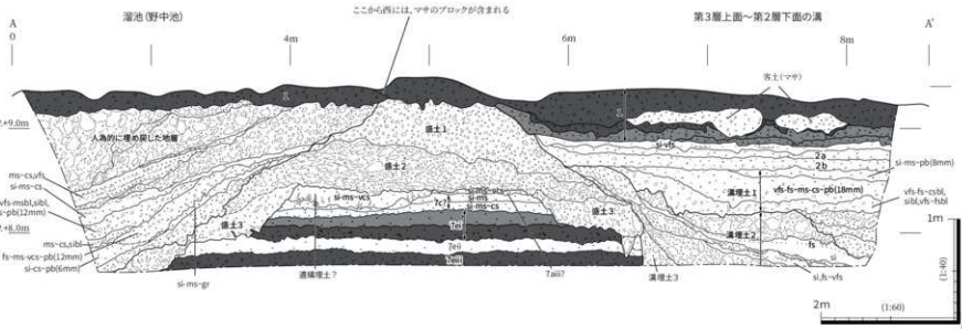
図 16 II区 第3 a層上面「野中池」堤断面図
