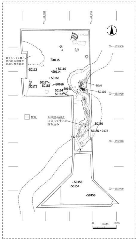
図11 III・IV区 第7 a ii層関連遺構平面図（古墳時代中期、5世紀）
