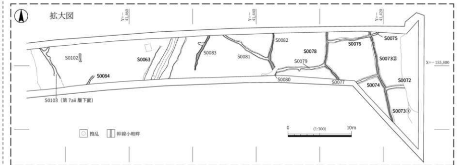
図8 II区 第7c層上面平面図(弥生時代後期～庄内式期頃、2～3世紀)
