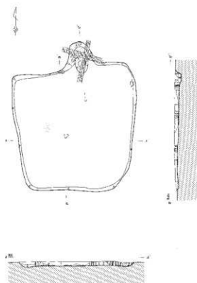
第58号住居跡 (58H: A-A', B-B')
