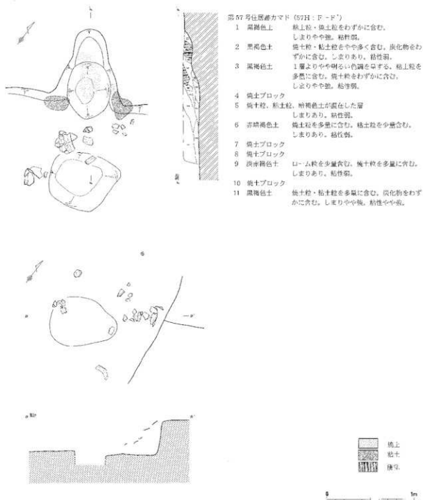
第12図 第56号・第57号住居跡 3 (56H・57H: 1/30)
