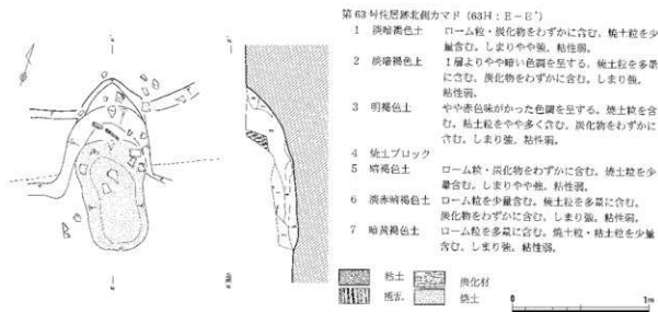
第20図 第62号・第63号住居跡 3 (62H・63H: 1/30)
