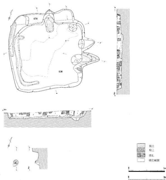
第62号・第63号住居跡 (62H・63H: A-A', B-B')
