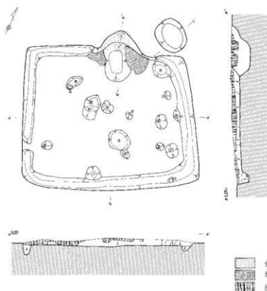
第1号住居跡 (1H: A-A', B-B')
