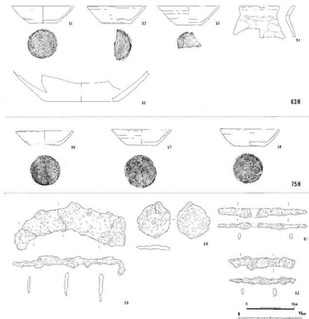
第24図 東台遺跡第35地点出土遺物3 (1/4、1/3)
