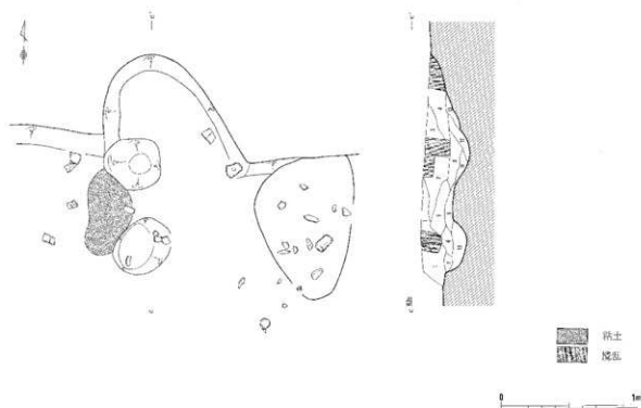
第59号住居跡カマド (59H : C-G)
