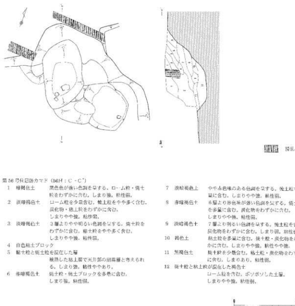
第11図 第56号・第57号住居跡2 (56H・57H: 1/30)
