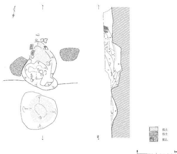
第60号住居跡方マド (60H: E-W)
