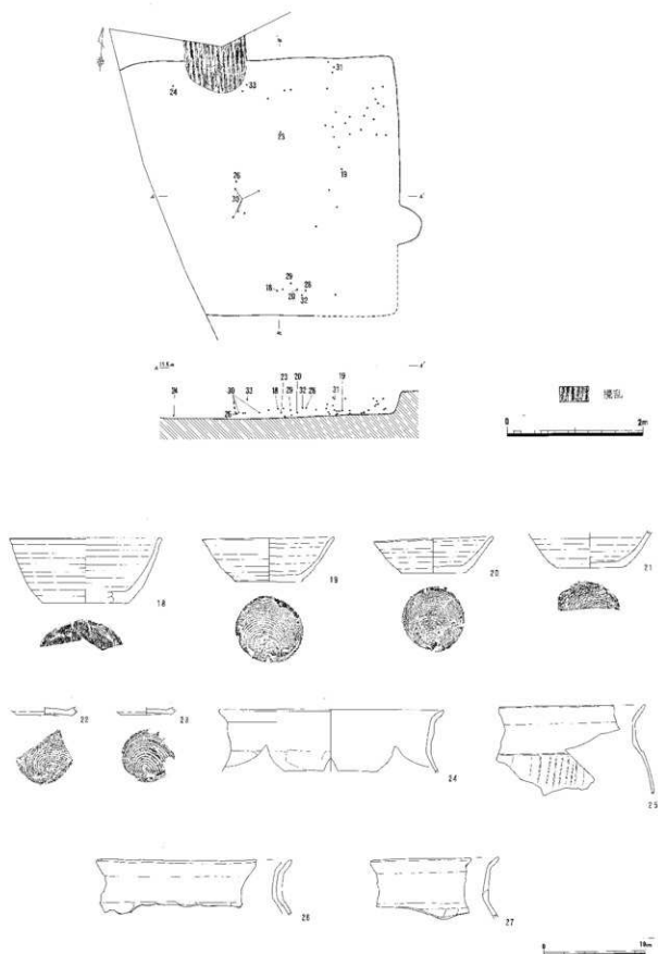
第21図 第37号住居跡及び出土遺物 (37H : 1/60、1/4)
