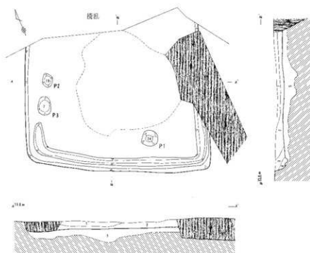
第38号住居跡土層解説 (38H : A-A', B-B')
