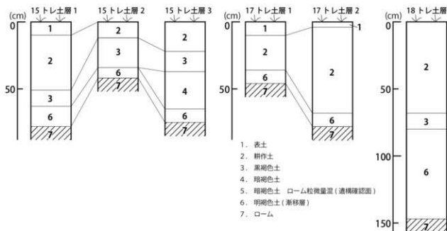
第4図 土層図② (1/20)
