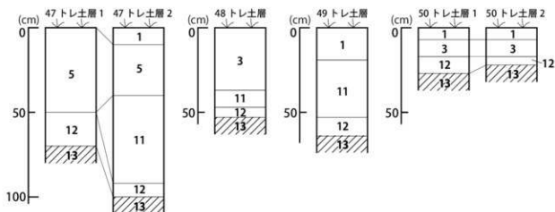
第10図 土層図① (1/20)
