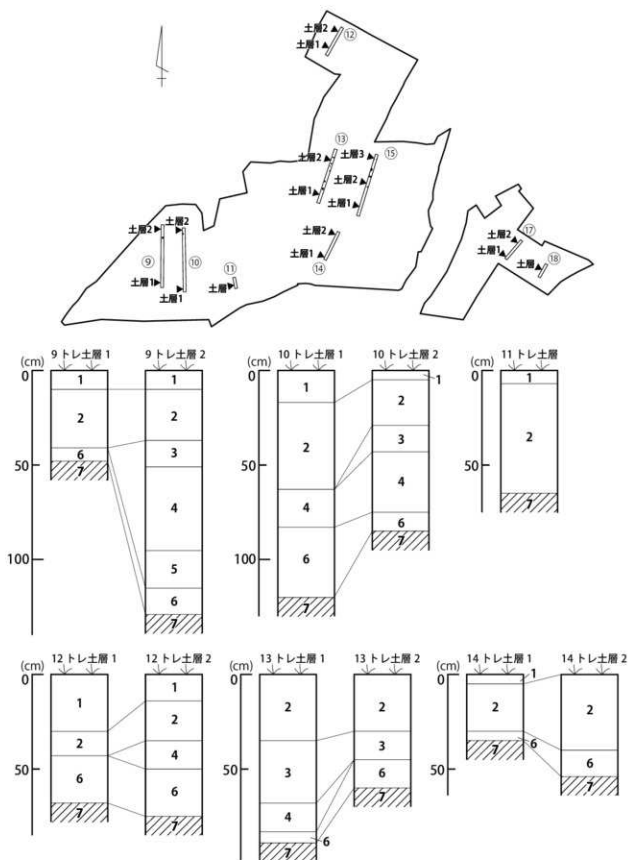
第3図 トレンチ配置図 (1/2,000)・土層図① (1/20)
