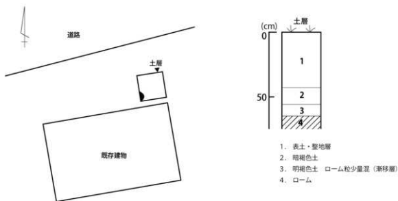
第28図 トレンチ配置図 (1/200)・土層図 (1/20)
