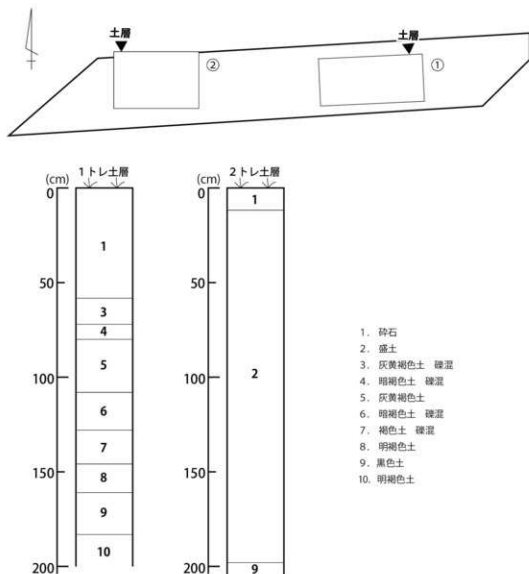
第30図 トレンチ配置図 (1/200)・土層図 (1/20)
