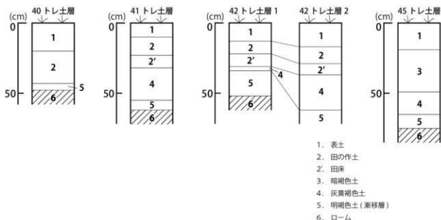
第22図 土層図 (1/20)
