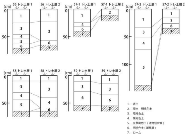
第14図 土層図 (1/20)
