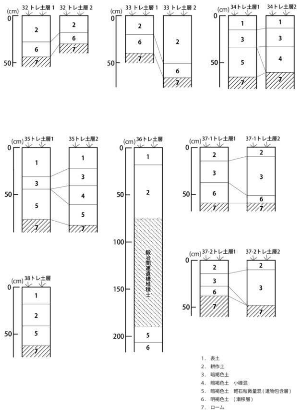
第8図 土層図② (1/20)
