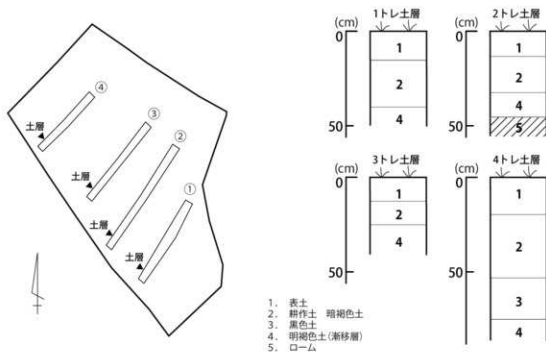
第24図 トレンチ配置図 (1/800)・土層図 (1/20)
