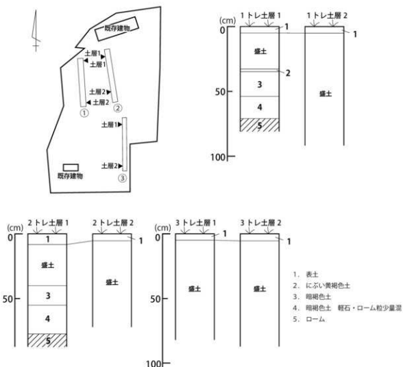
第26図 トレンチ配置図 (1/800)・土層図 (1/20)
