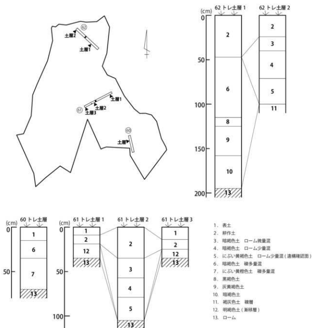
第16図 トレンチ配置図 (1/2,000)・土層図 (1/20)
