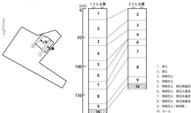
第32図 トレンチ配置図 (1/800)・土層図 (1/20)
