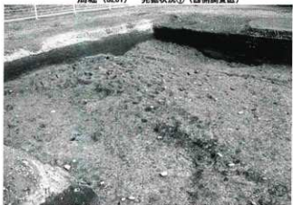
周堀 (SZ01) スロープ状部分完掘状況① (調査区西側)
