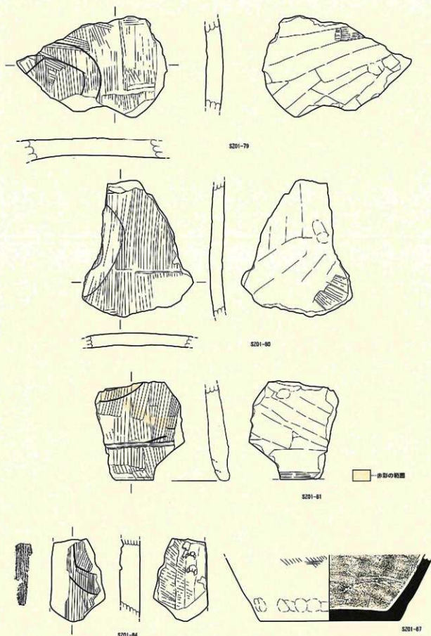
第10図 周堀 (SZ01) 出土遺物④ (S=1/3)
