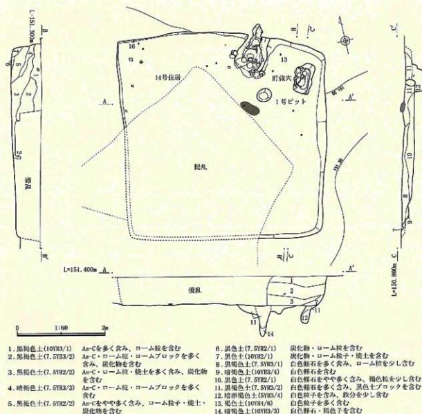
第34図 14号住居平面図・断面図(S=1/60)
