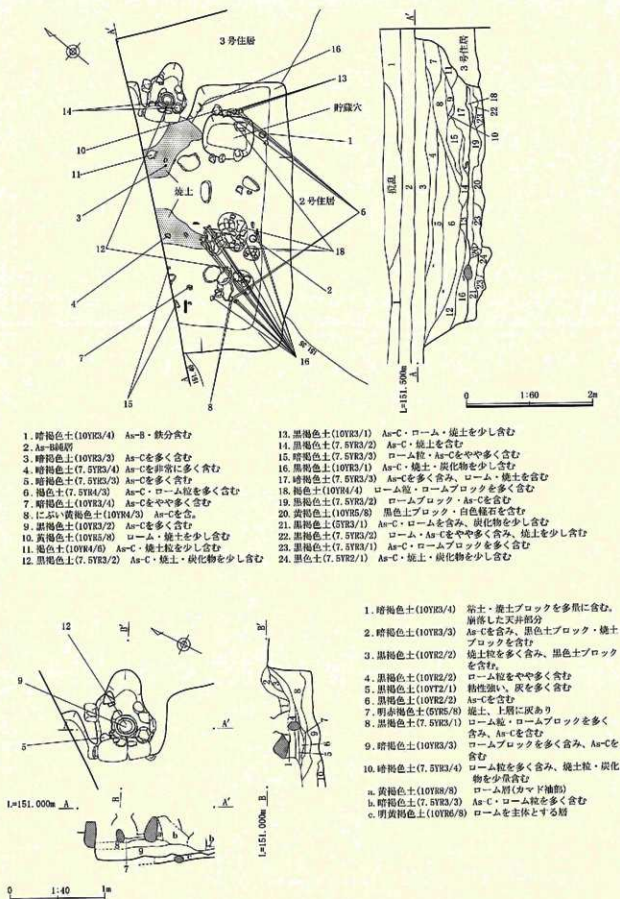
第7図 2号住居平面図・断面図(S=1/60) カマド平面図・断面図(S=1/40)
