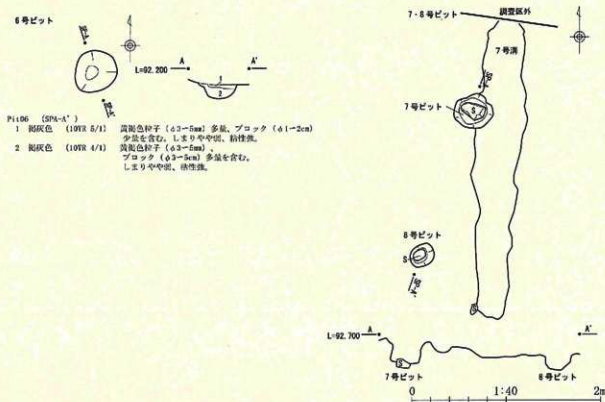
第21図 6～8号ビット平面図・断面図 (S=1/40)
