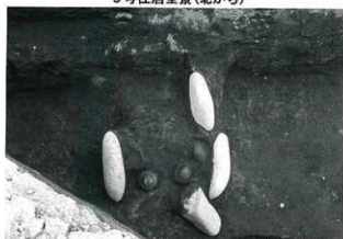
9号住居カマド遺物取り上げ後の支脚と袖石(北から)
