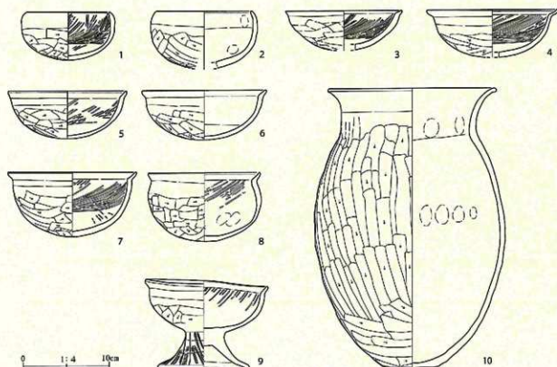
第45図 19号住居出土遺物(S=1/4)
