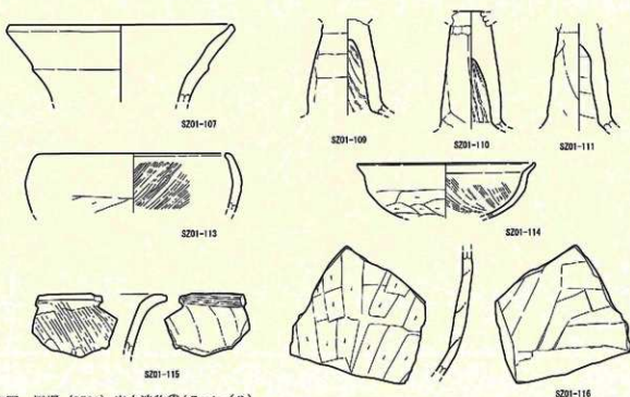
第12図 周堀 (SZ01) 出土遺物⑧ (S=1/3)
