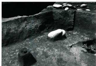
6号住居出土金床及び1号炉(東から)
