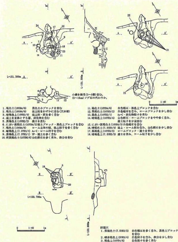
第35図 14号住居カマド平面図・断面図 (S=1/40) 貯蔵穴平面図・断面図 (S=1/40)
