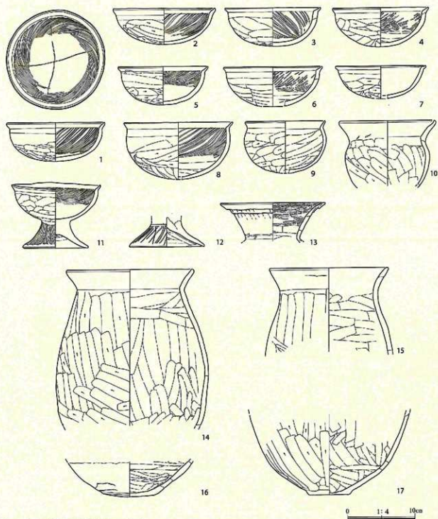
第29図 11号住居出土土遺物(S=1/4)
