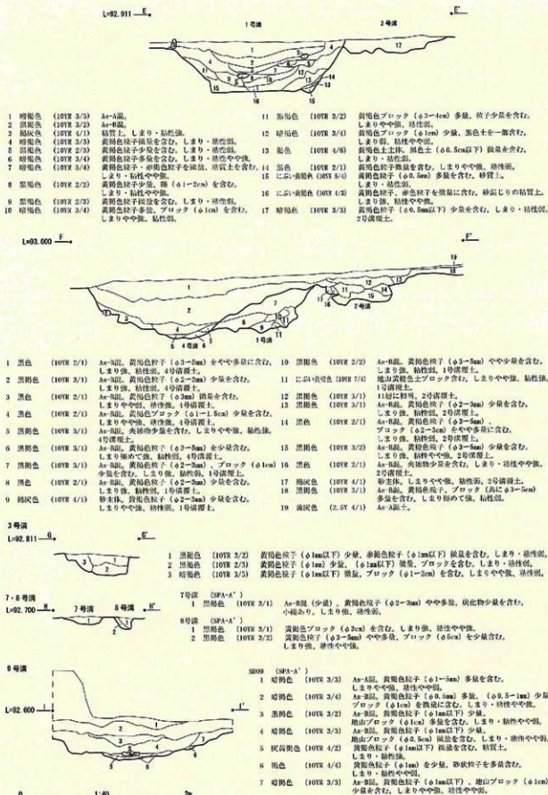
第13図 溝断面図 (S=1/40)
