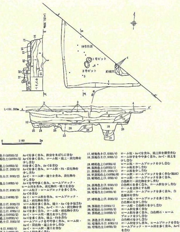
第42図 18号住居平面図・断面図(S=1/60)
