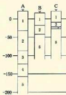
土層柱状図
