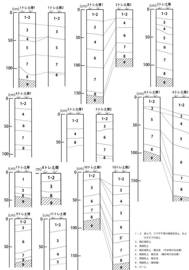
第4図 土層図 (1/20)
