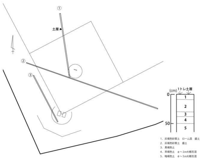
第17図 トレンチ配置図 (1/400)・土層図 (1/20)
