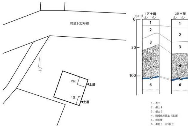
第 7 図 トレンチ配置図 (1/300)・土層図 (1/20)
