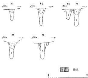
第11図 第23号住居跡2 (23J : 1/60)
