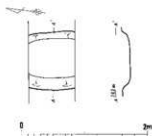
第28図 第32号土坑 (32HD : 1/60)
