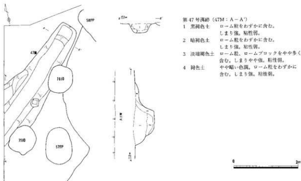
第24図 第47号溝跡 (47M: 1/60)
