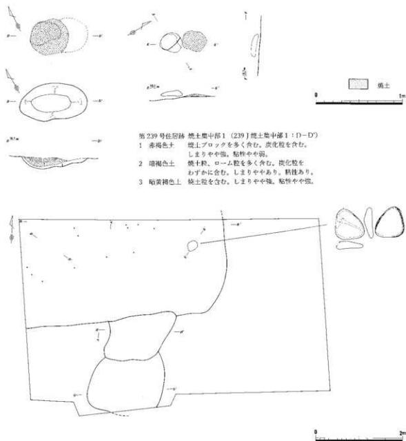
第5図 第239号住居跡焼土集中部・遺物出土状況 (239 J : 1/30・1/60)
