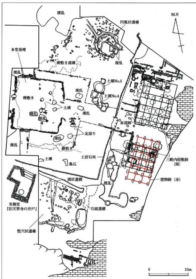
第6図 主な遺構配置図
