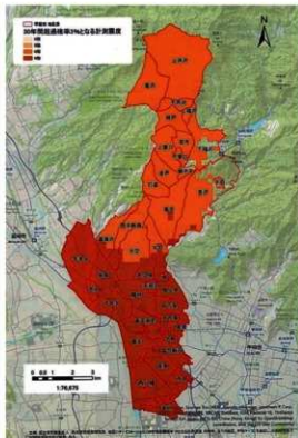
図25 確率的地震動予想地図 〔『甲斐市国土強靱化地域計画』から転載〕
