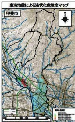
図26 液状化危険度マップ(甲斐市) (山梨県ウェブサイトから転載)
