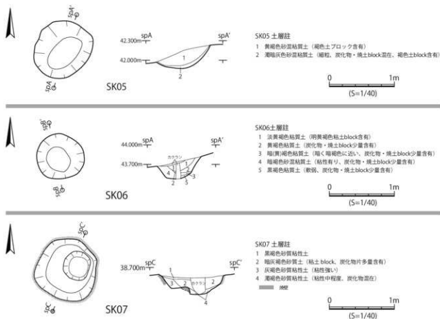
第39図 土坑SK05、SK06、SK07 平面図・断面図
