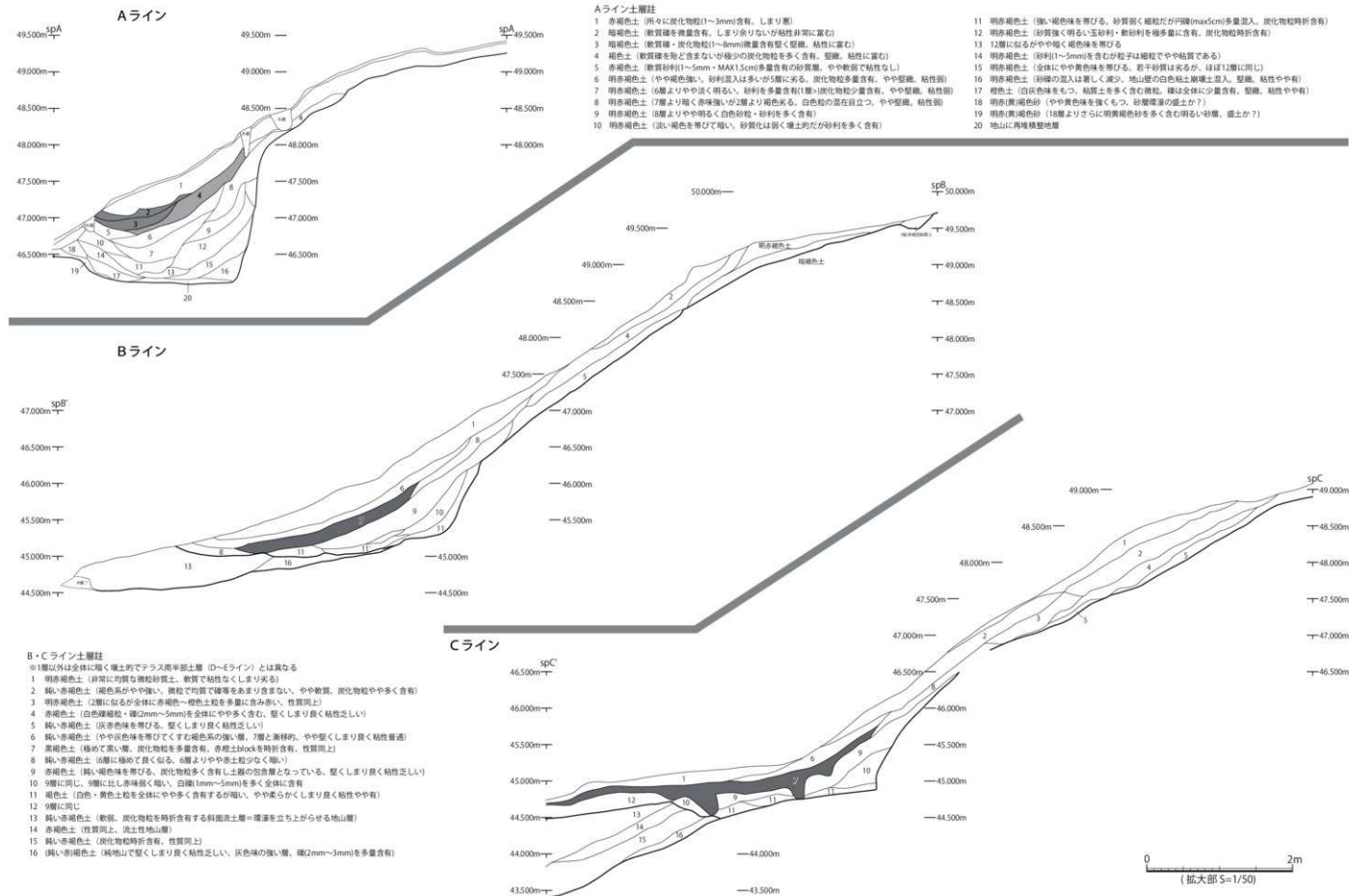
第18図 環濠土層断面図 (1)
