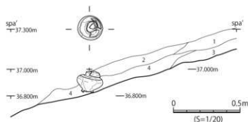
第35図 2号火葬墓 平面図・断面図
