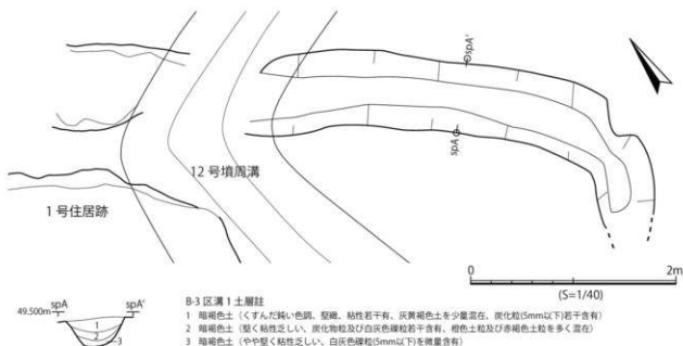
第26図 B-3溝1平面図・土層断面図
