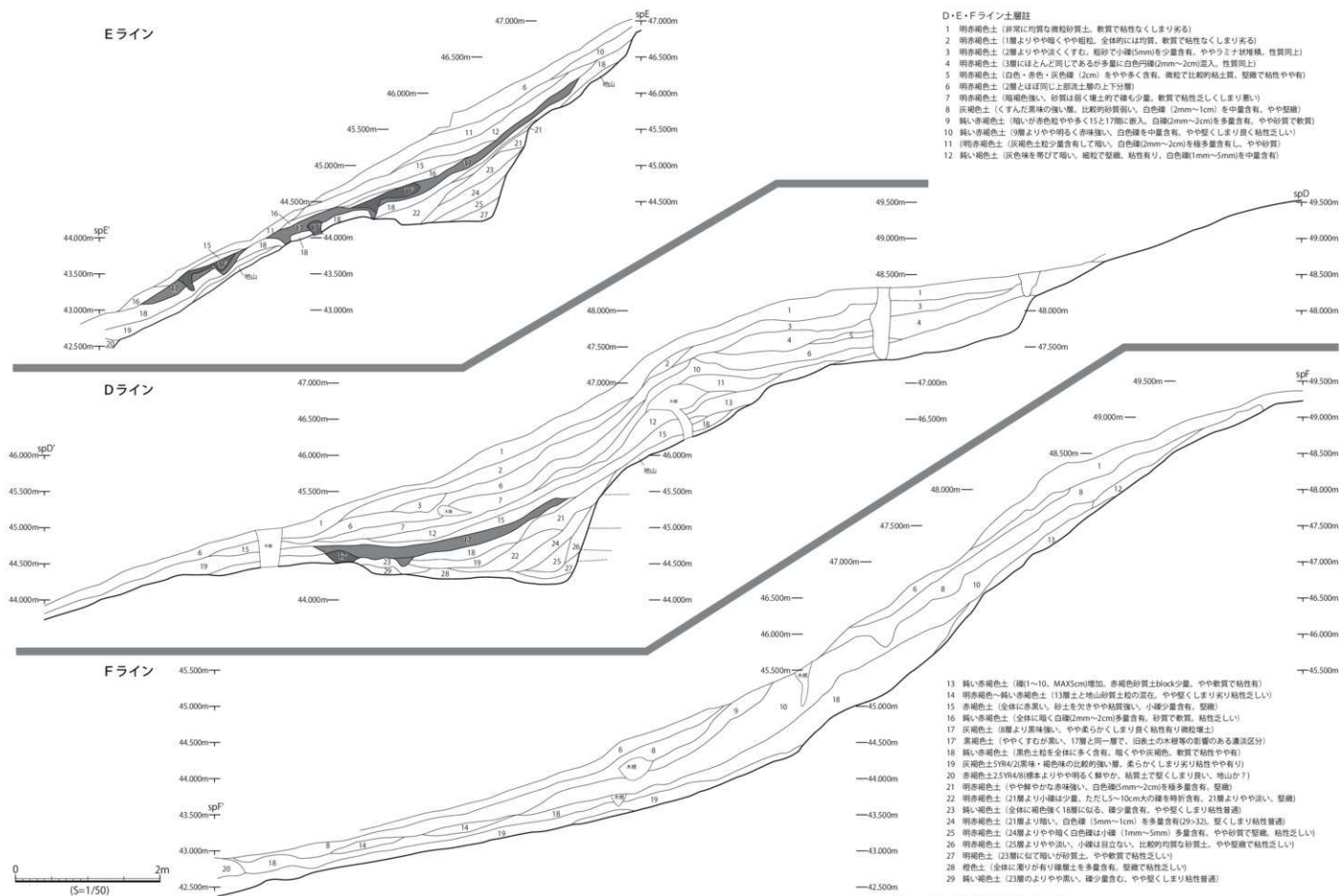
第19図 環濠土層断面図(2)
