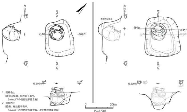
第32図 1号火葬墓 平面図・断面図
