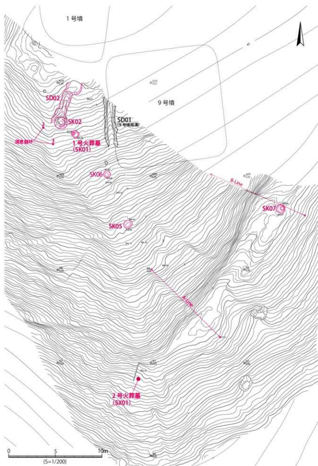
第 31 図 B-2 区 奈良時代遺構分布図
